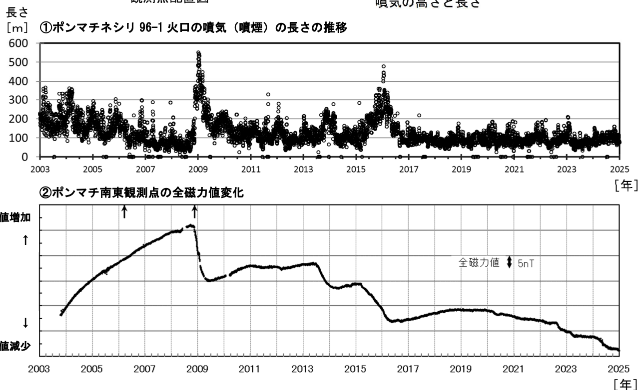
図5 雌阿寒岳 ホンマチネシリ96-1火口の噴気（噴煙）の長さと全磁力値の経過及び全磁力観測点配置図（2003年～2024年12月）
