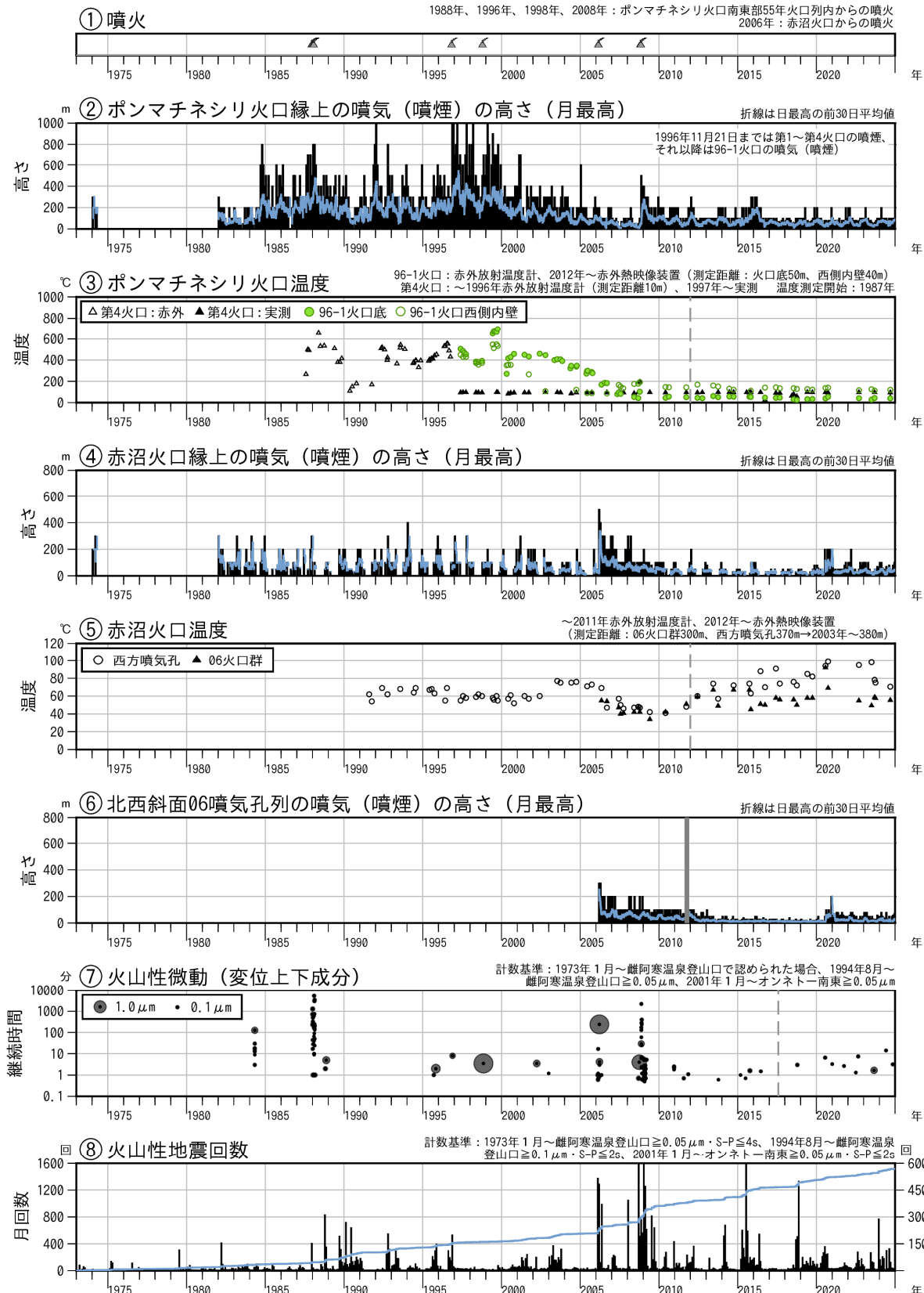
図4 雌阿寒岳 火山活動経過図（1973年1月～2024年12月）
