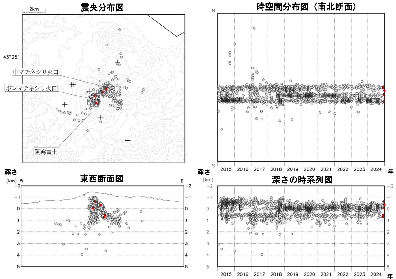
図6 雌阿寒岳 火山性地震の震源分布（2015年1月～2024年12月） ●：2015年1月～2024年11月の震源 ●：2024年12月の震源 +：地震観測点
