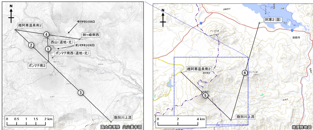
図8 雌阿寒岳 GNSS連続観測の基線図
