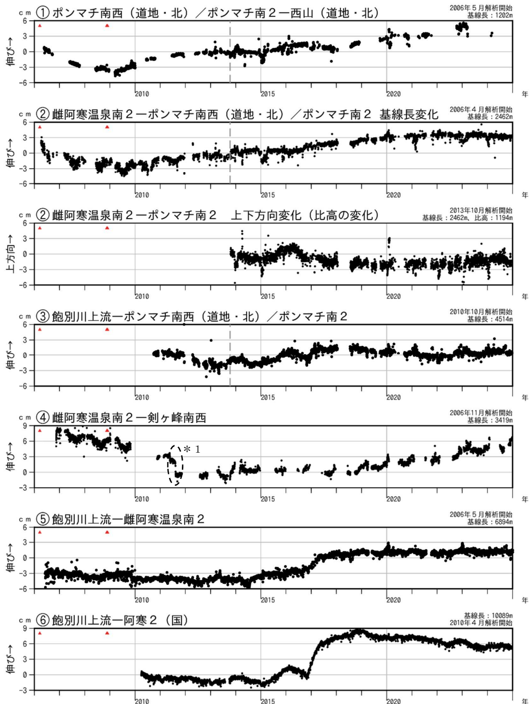
図7 雌阿寒岳 GNSS連続観測による基線長及び比高の変化（2006年4月～2024年12月）
