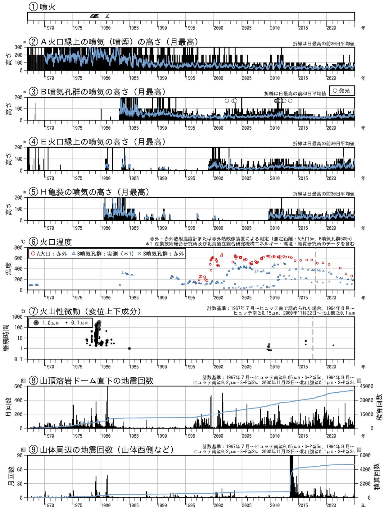
図2 樽前山 火山活動経過図（1967年1月～2024年12月）
