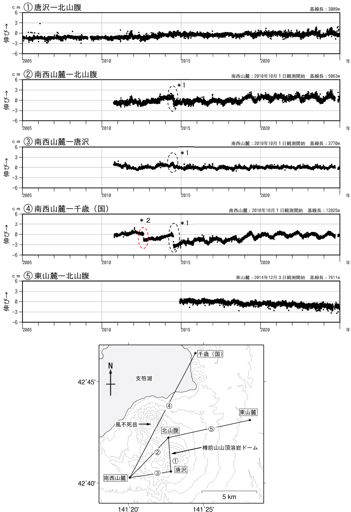
図 4 樽前山 GNSS連続観測による基線長変化（2005年1月～2024年12月）及び観測点配置図
