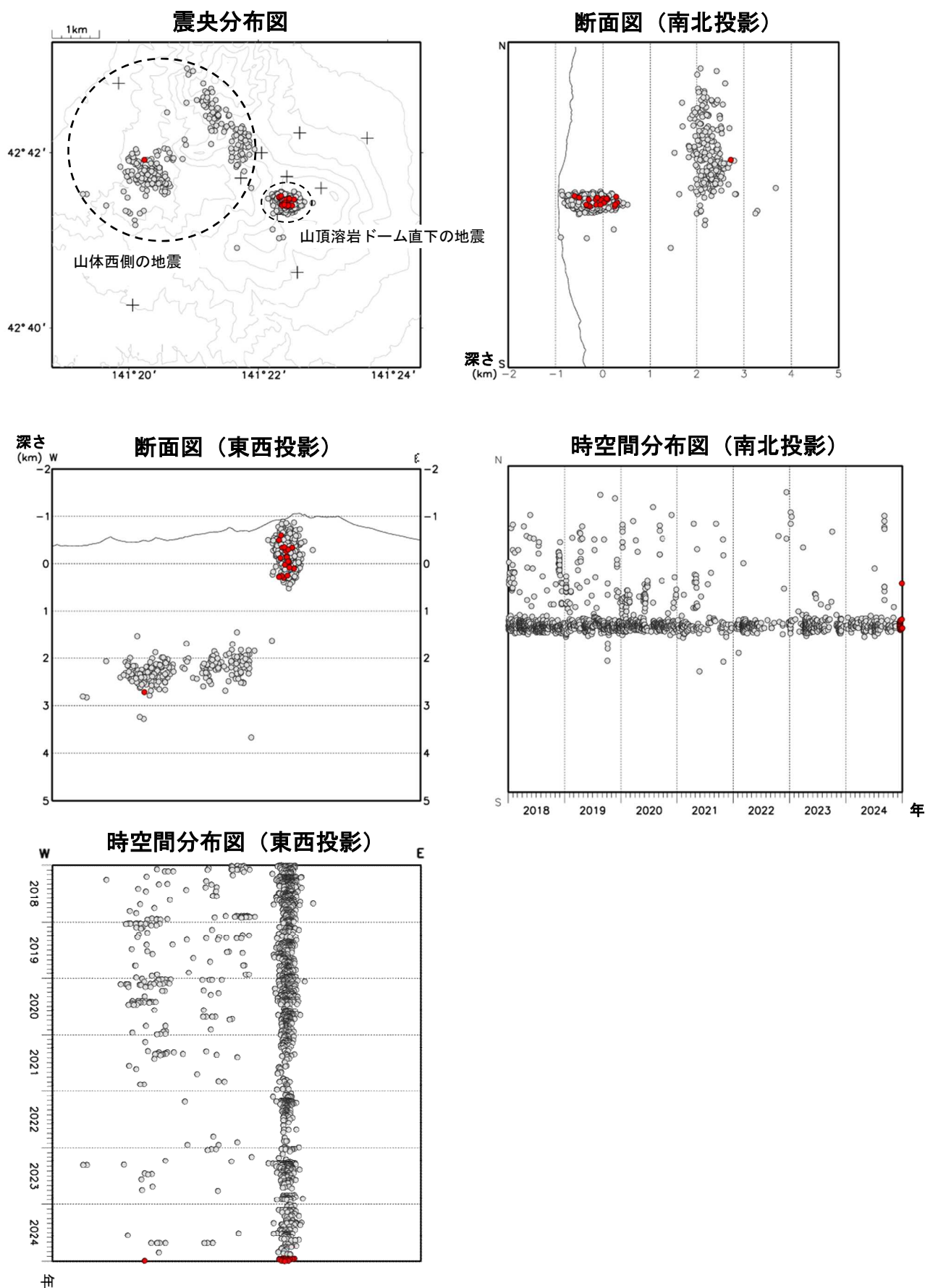
図3 樽前山 火山性地震の震源分布（2018年1月～2024年12月）
