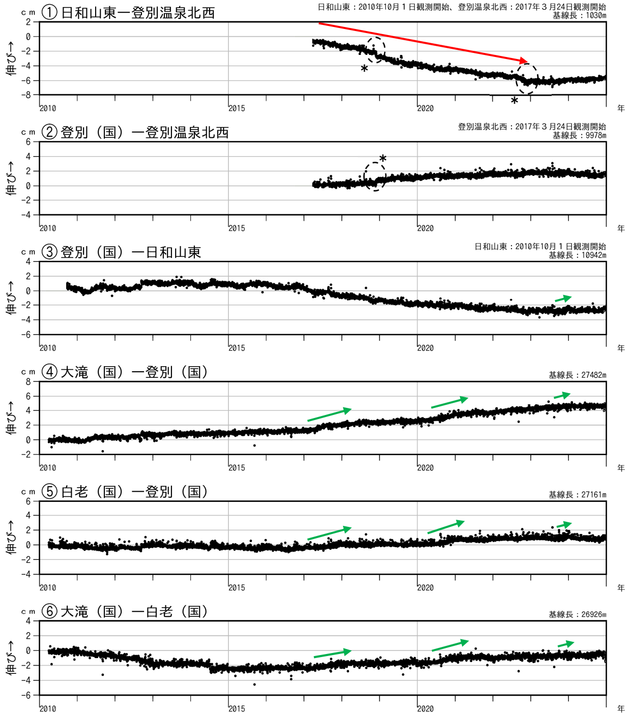
図3 倶多楽 GNSS連続観測による基線長変化（2010年4月～2024年12月）
