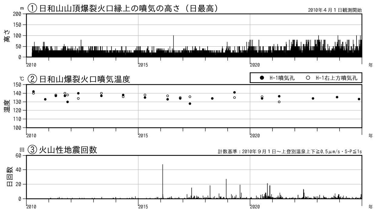
図2 倶多楽 火山活動経過図（2010年1月～2024年12月）
