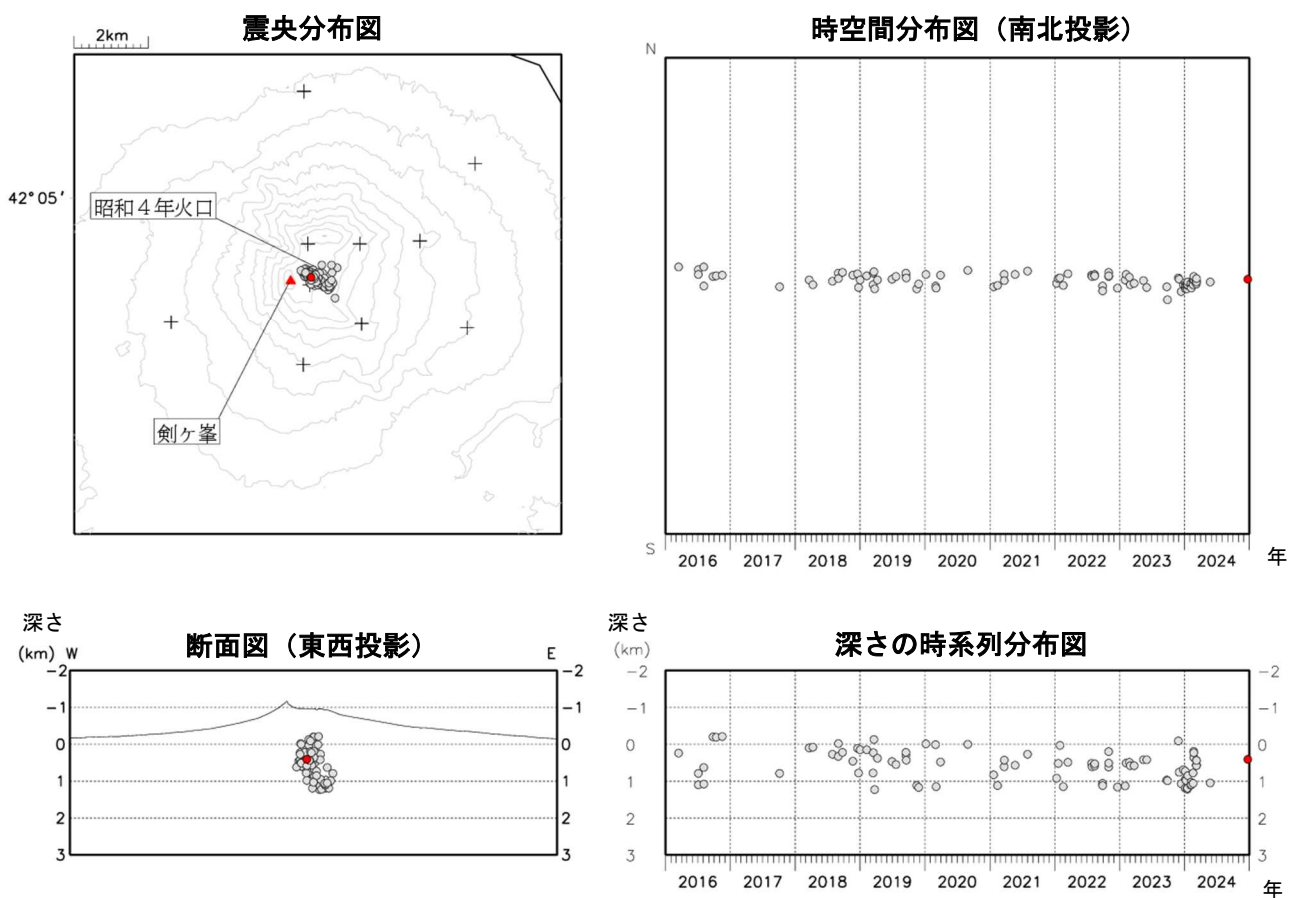
図4 北海道駒ヶ岳 火山性地震の震源分布（2016年1月～2024年12月）
