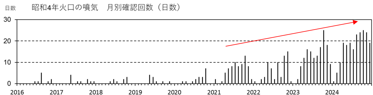
図2 北海道駒ヶ岳 昭和4年火口のごく弱い噴気を観測した日数（2016年1月～2024年12月） 山頂部に設置した剣ヶ峰監視カメラ及び駒ヶ岳山頂（道）監視カメラ（位置は図7、 図8参照）による観測結果です。 冬季は雪氷付着のため欠測日が多くなる傾向があります。
