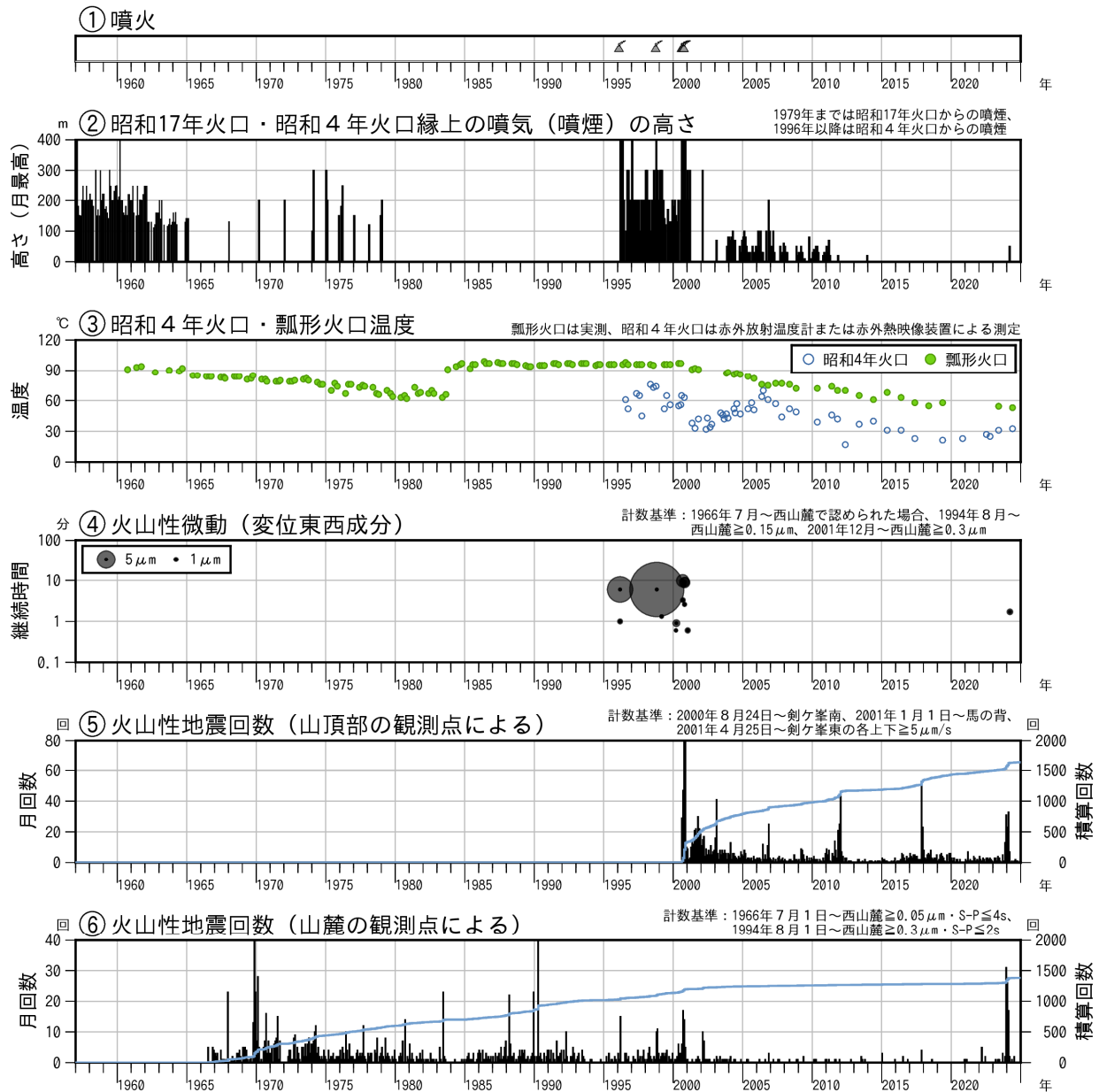
図1 北海道駒ヶ岳 火山活動経過図（1957年1月～2024年12月） 各火口の位置は図7、図8を参照してください。
