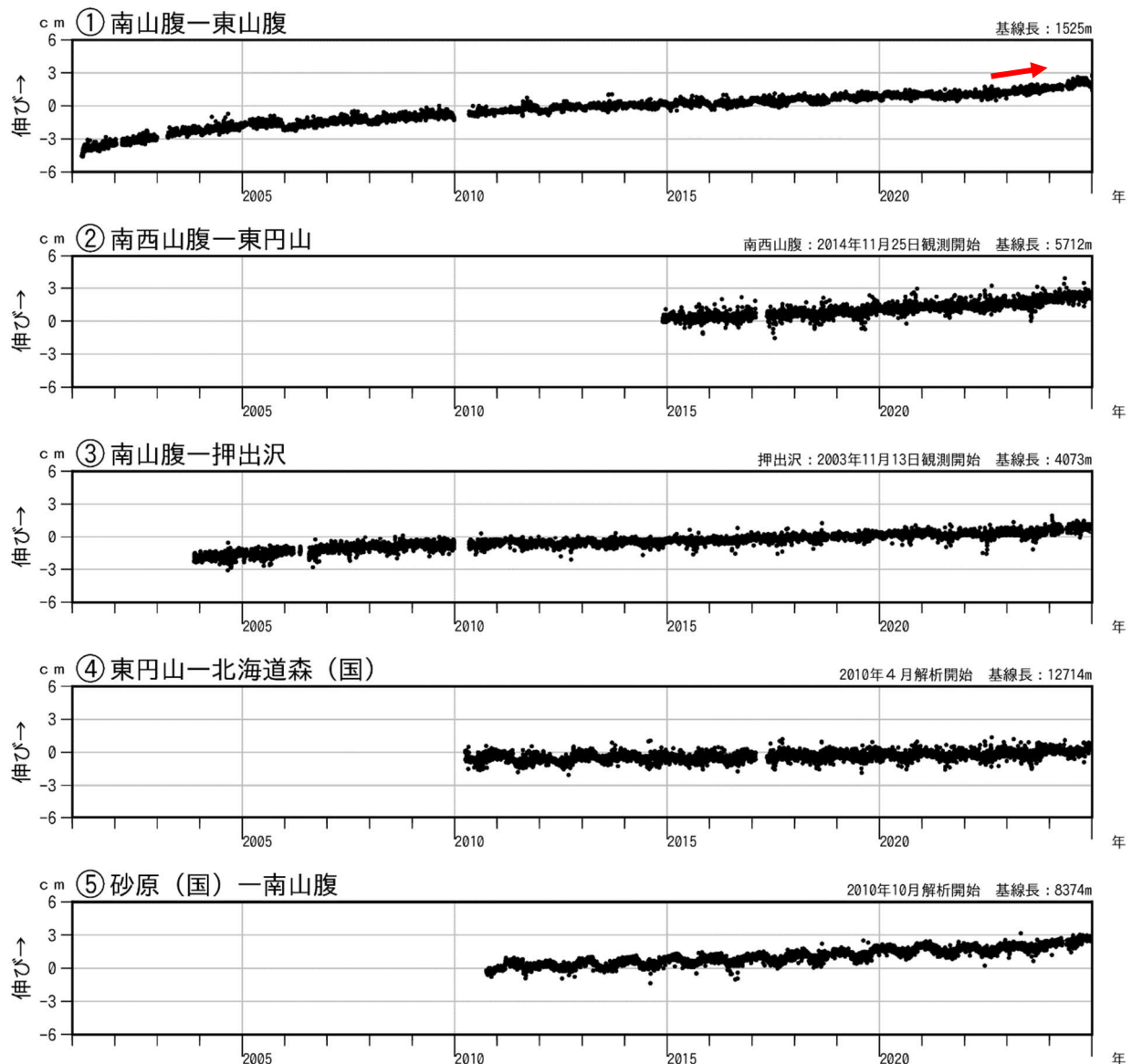
図5 北海道駒ヶ岳 GNSS連続観測による基線長変化（2001年4月～2024年12月）
