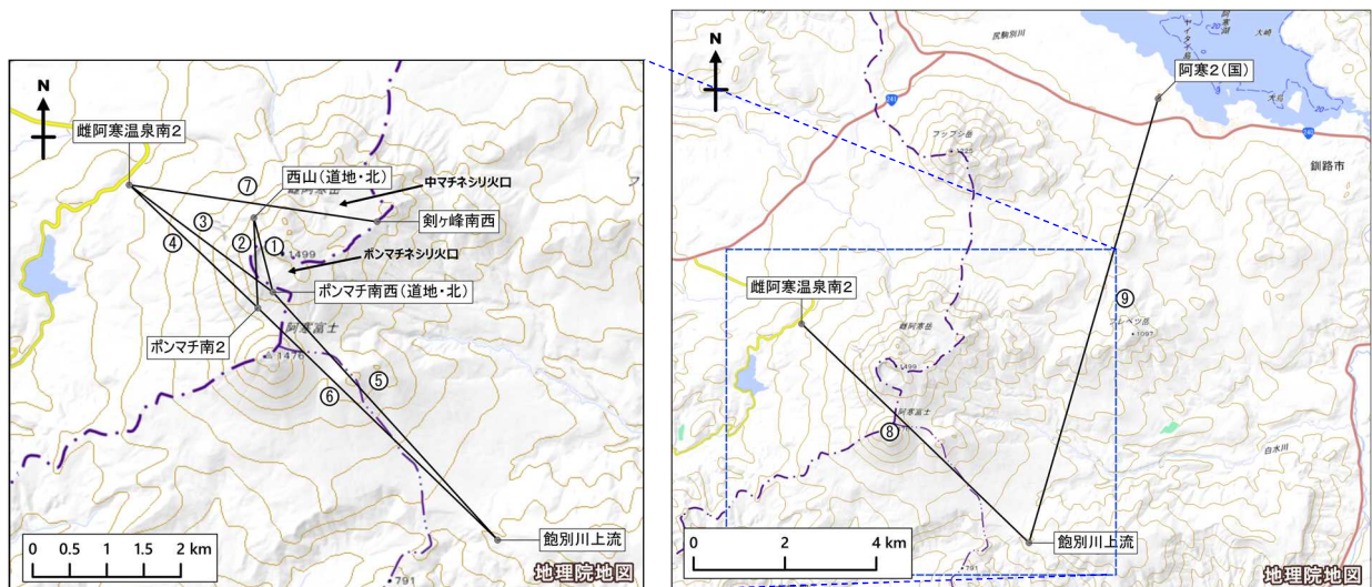
図8 雌阿寒岳 GNSS連続観測の基線図
