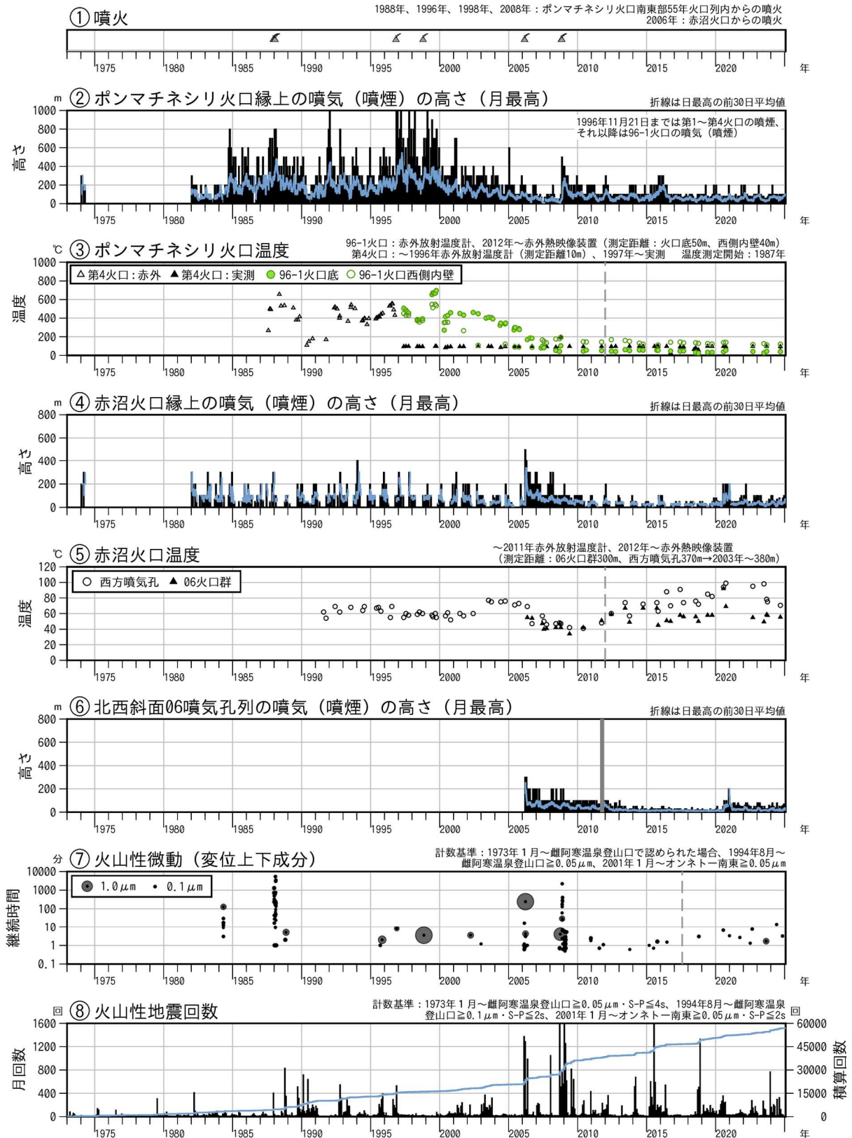
図4 雌阿寒岳 火山活動経過図（1973年1月～2025年1月）
