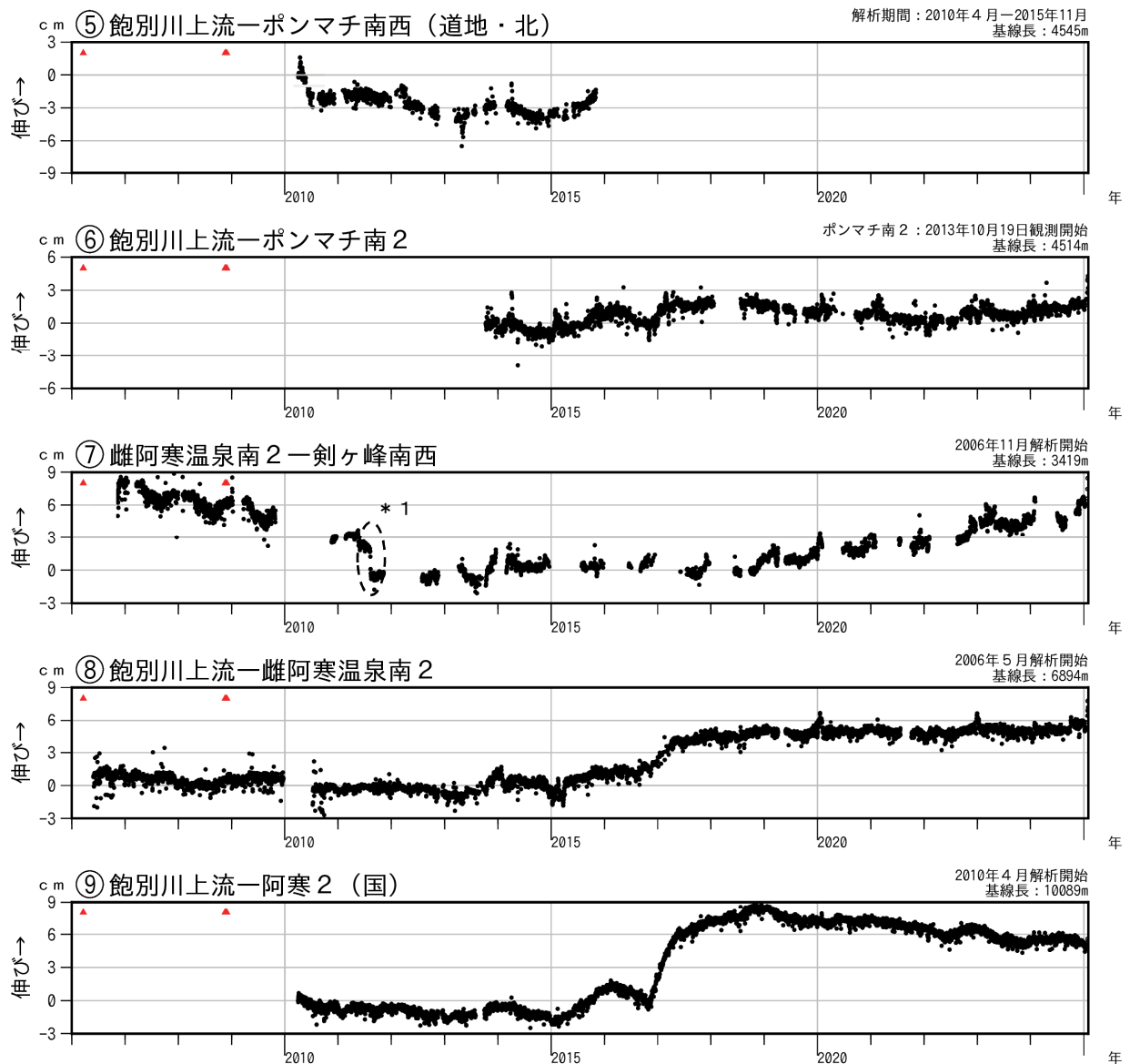
図7-2 雌阿寒岳 GNSS連続観測による基線長の変化（2006年4月～2025年1月）
