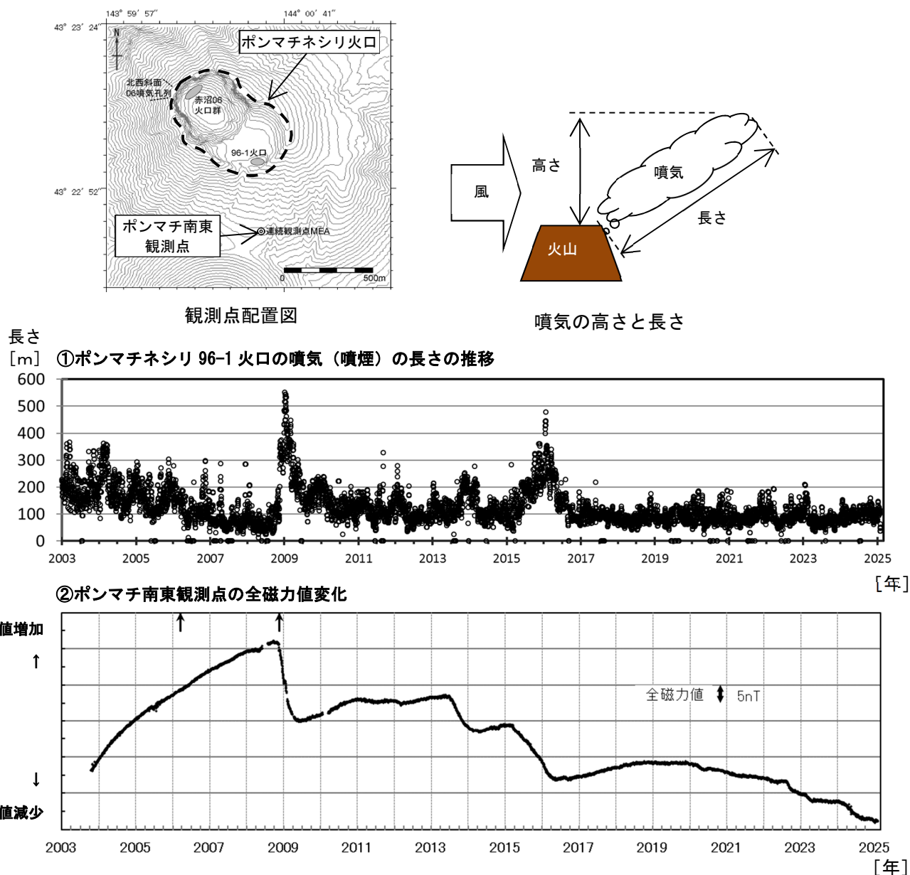
図5 雌阿寒岳 ホンマチネシリ96-1火口の噴気（噴煙）の長さと全磁力値の経過及び全磁力観測点配置図（2003年～2025年1月）
