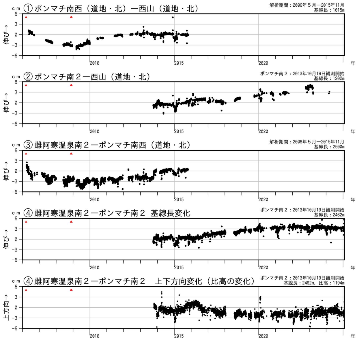
図7-1 雌阿寒岳 GNSS連続観測による基線長及び比高の変化（2006年4月～2025年1月）
