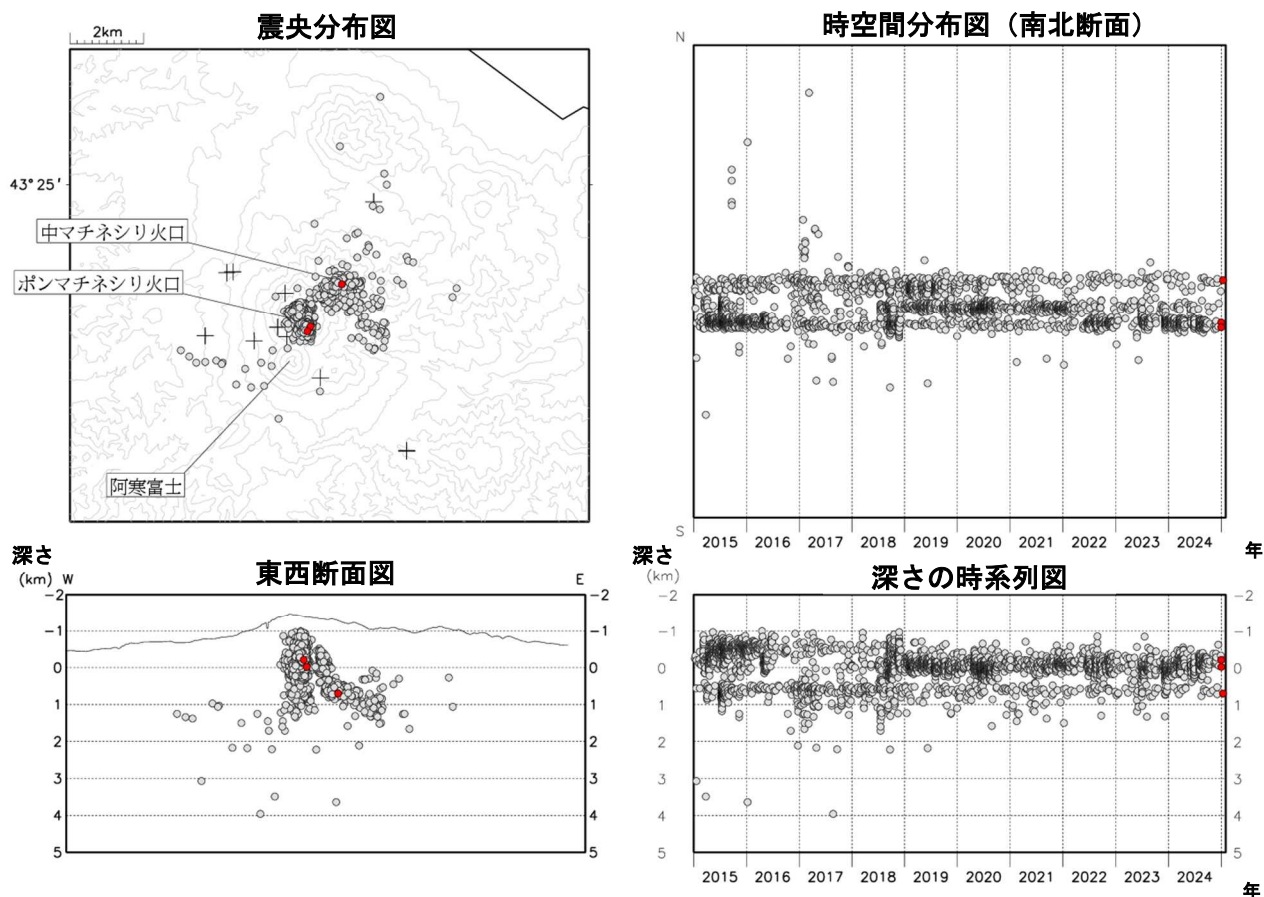
図 6 雌阿寒岳 火山性地震の震源分布（2015年 1 月～2025年 1 月） ●：2015年 1 月～2024年12月の震源 ●：2025年 1 月の震源 +：地震観測点
