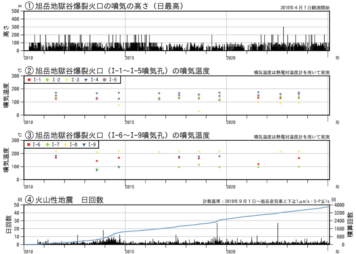
図2 大雪山 火山活動経過図（2010年4月～2025年1月）
