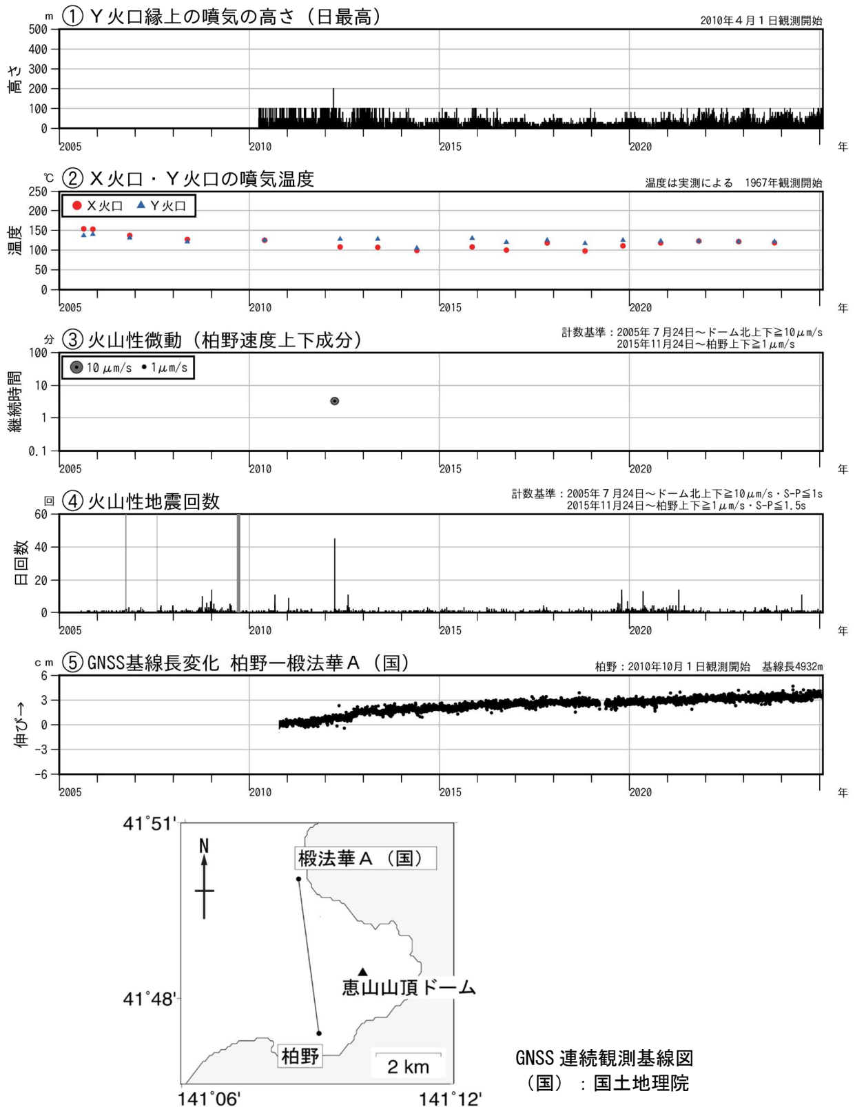
図 2 恵山 火山活動経過図（2005 年 7 月～2025 年 1 月） ④の灰色部分は機器障害による欠測期間を示します。 ⑤のグラフは上図の基線に対応しています。 ⑤のグラフの空白部分は欠測を示します。
