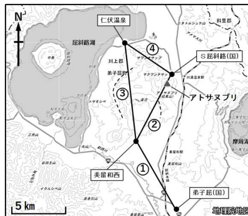
図4 アトサヌプリ GNSS連続観測による基線長変化（2010年10月～2025年2月）及び観測点配置図 冬季に凍上や積雪の影響によると考えられる変動がみられる基線があります。 ①の破線内の変動（* 1）は、弟子屈(国)付近の樹木の影響及び伐採によるものです。 グラフの空白部分は欠測を示します。 * 2 勝井義雄（1958）阿寒・屈斜路火山群、地球科学、39巻。 ・各基線①～④では、2021年秋頃からアトサヌプリ西側深部の膨張を示す基線長の変化が認められていましたが（ 赤矢印 ）、2024年1月以降は停滞しています。
