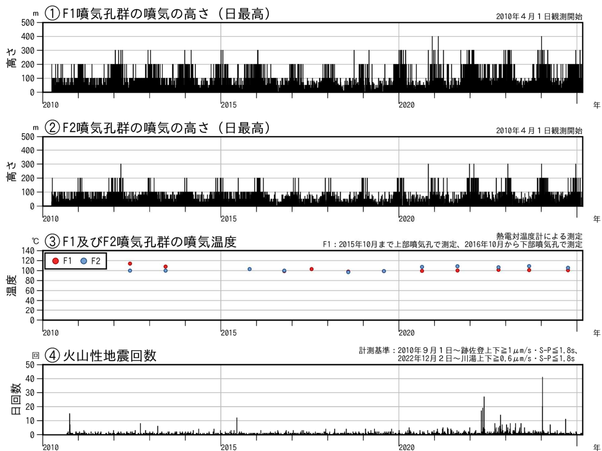
図1 アトサヌプリ 火山活動経過図（2010年4月～2025年2月）
