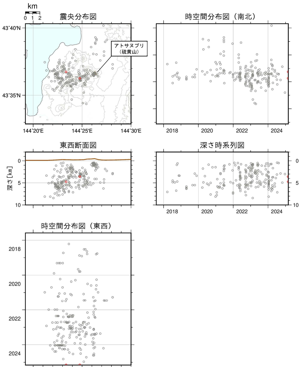
図3 アトサスプリ 火山性地震の震源分布（2017年8月～2025年2月） ○：2017年8月～2025年1月の震源 ○：2025年2月の震源
