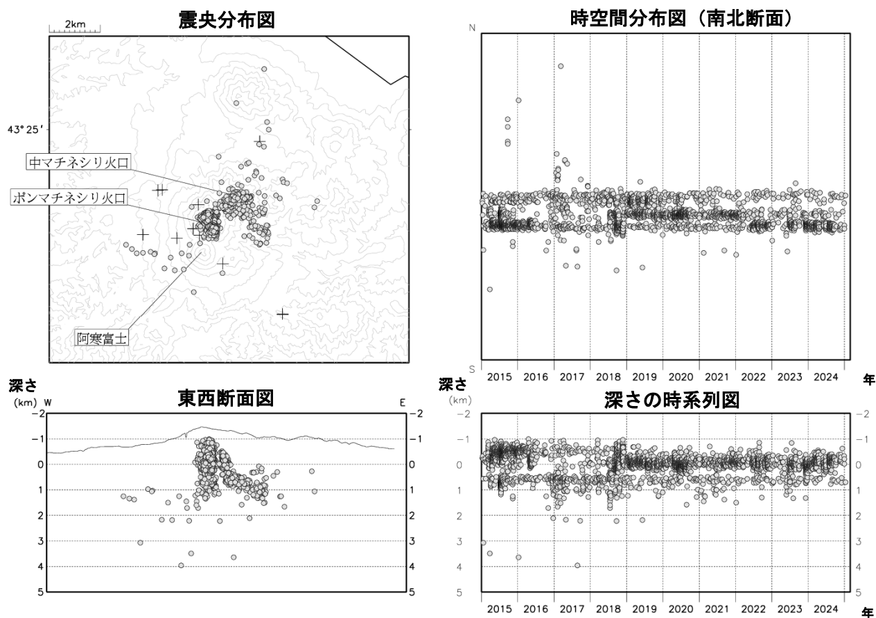
図6 雌阿寒岳 火山性地震の震源分布（2015年1月～2025年2月） ●：2015年1月～2025年1月の震源 +：地震観測点
