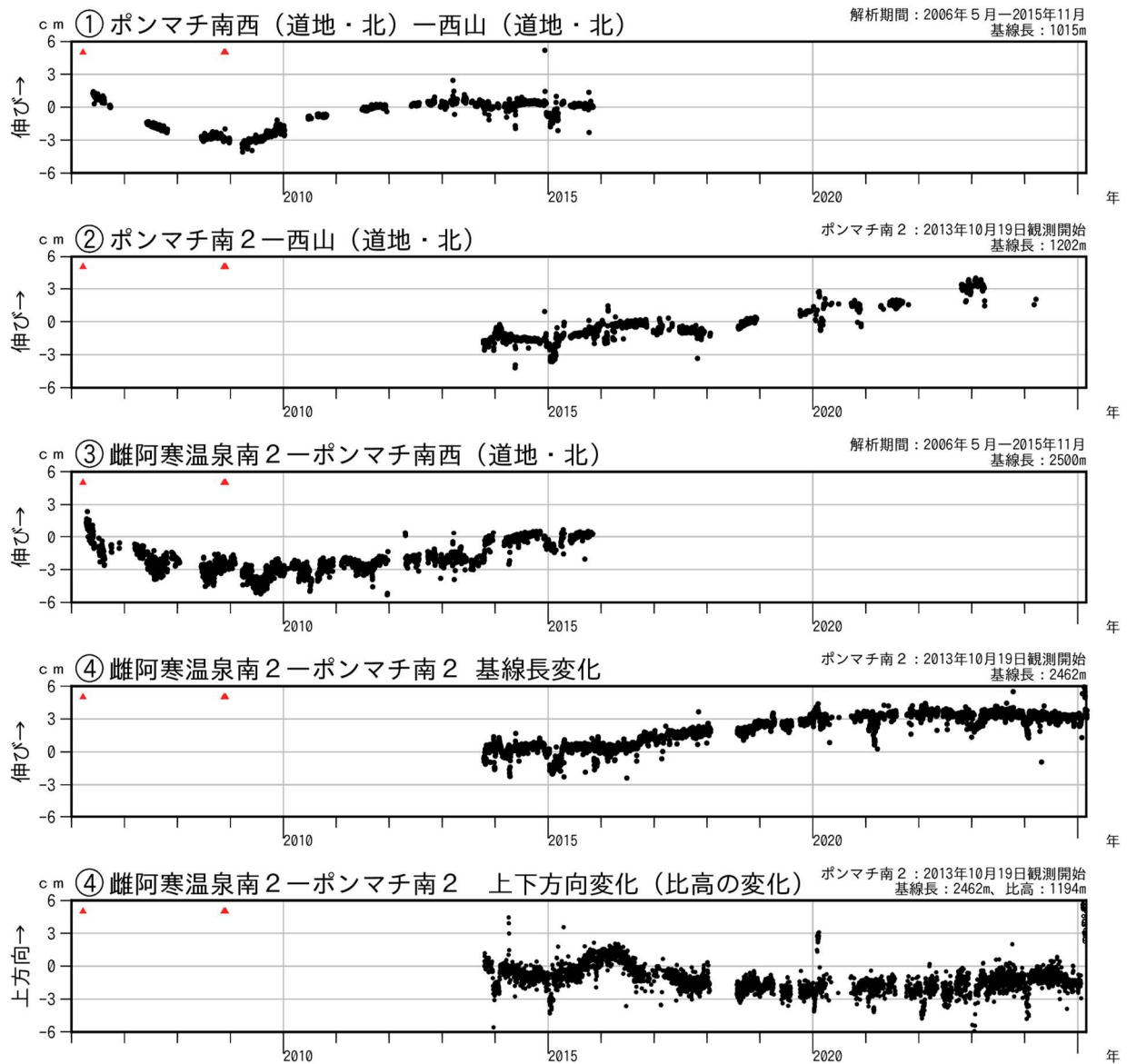
図7-1 雌阿寒岳 GNSS連続観測による基線長及び比高の変化（2006年4月～2025年2月）
