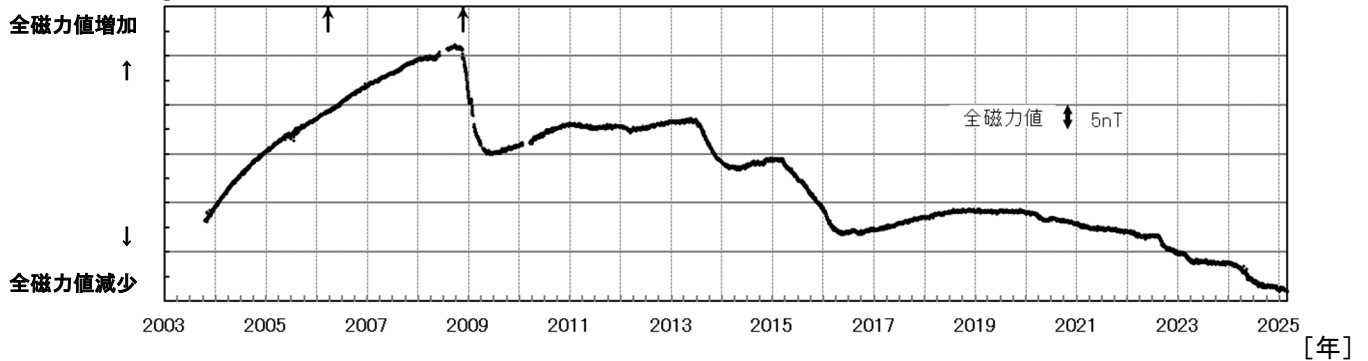
図5 雌阿寒岳 ポンマチネシリ96-1火口の噴気（噴煙）の長さや全磁力値の経過及び全磁力観測点配置図（2003年～2025年2月）
