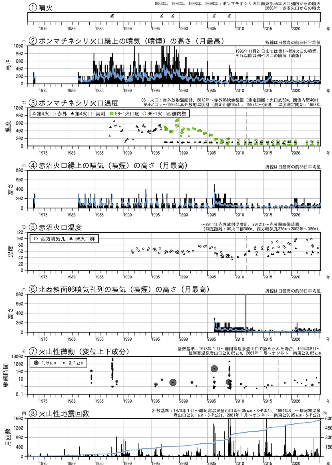
図4 雌阿寒岳 火山活動経過図（1973年1月～2025年2月）
