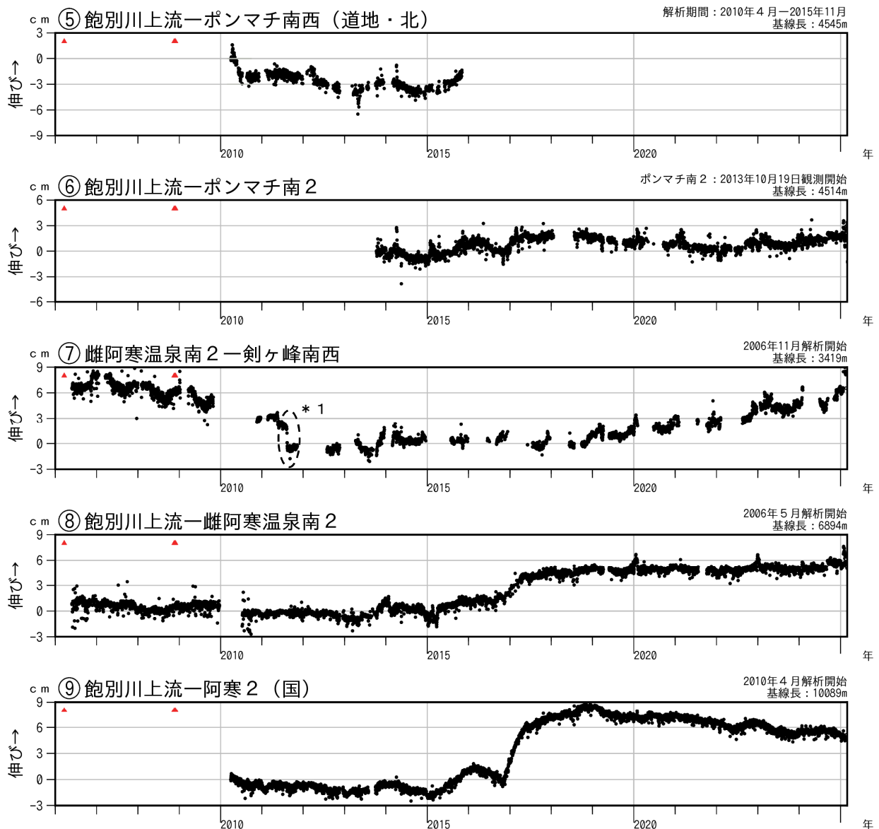
図7-2 雌阿寒岳 GNSS連続観測による基線長の変化（2006年 4 月～2025年 2 月）
