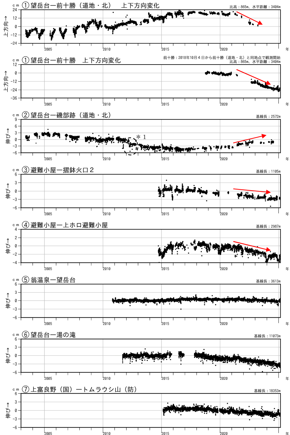
図5 十勝岳 GNSS連続観測による上下方向変化及び基線長変化（2003年5月～2025年2月）
