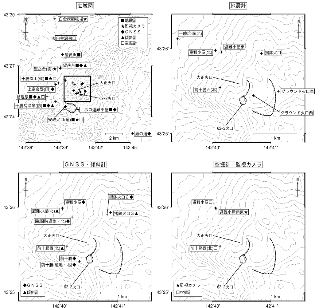
図7 十勝岳 観測点配置図
