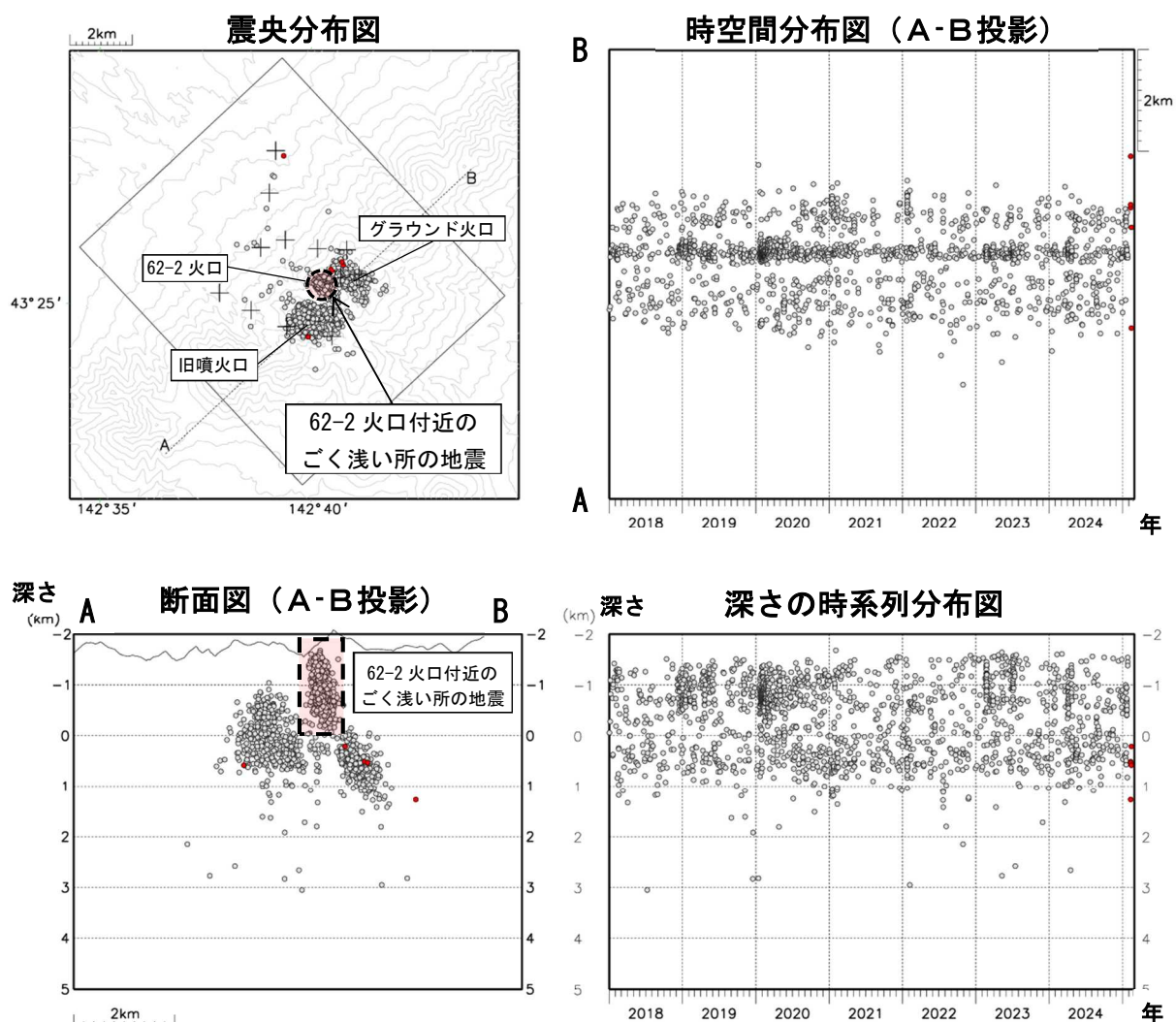
図4 十勝岳 火山性地震の震源分布（2018年1月～2025年2月）
