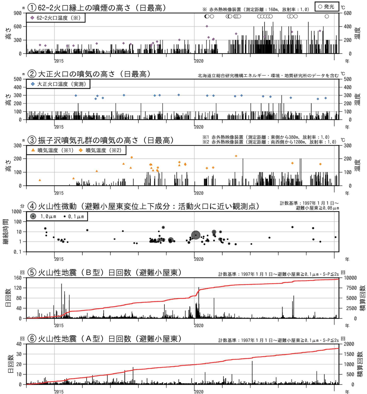
図2 十勝岳 火山活動経過図（2014年1月～2025年2月）
