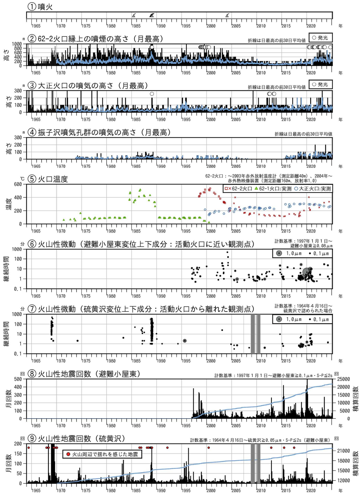
図1 十勝岳 火山活動経過図（1964年1月～2025年2月）
