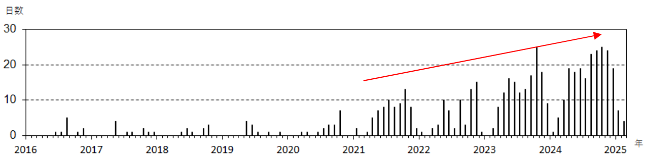
図2 北海道駒ヶ岳 昭和4年火口のごく弱い噴気を観測した日数（2016年1月～2025年2月） 山頂部に設置した剣ヶ峰監視カメラ及び駒ヶ岳山頂（道）監視カメラ（位置は図7、 図8参照）による観測結果です。 冬季は雪氷付着のため欠測日が多くなる傾向があります。
