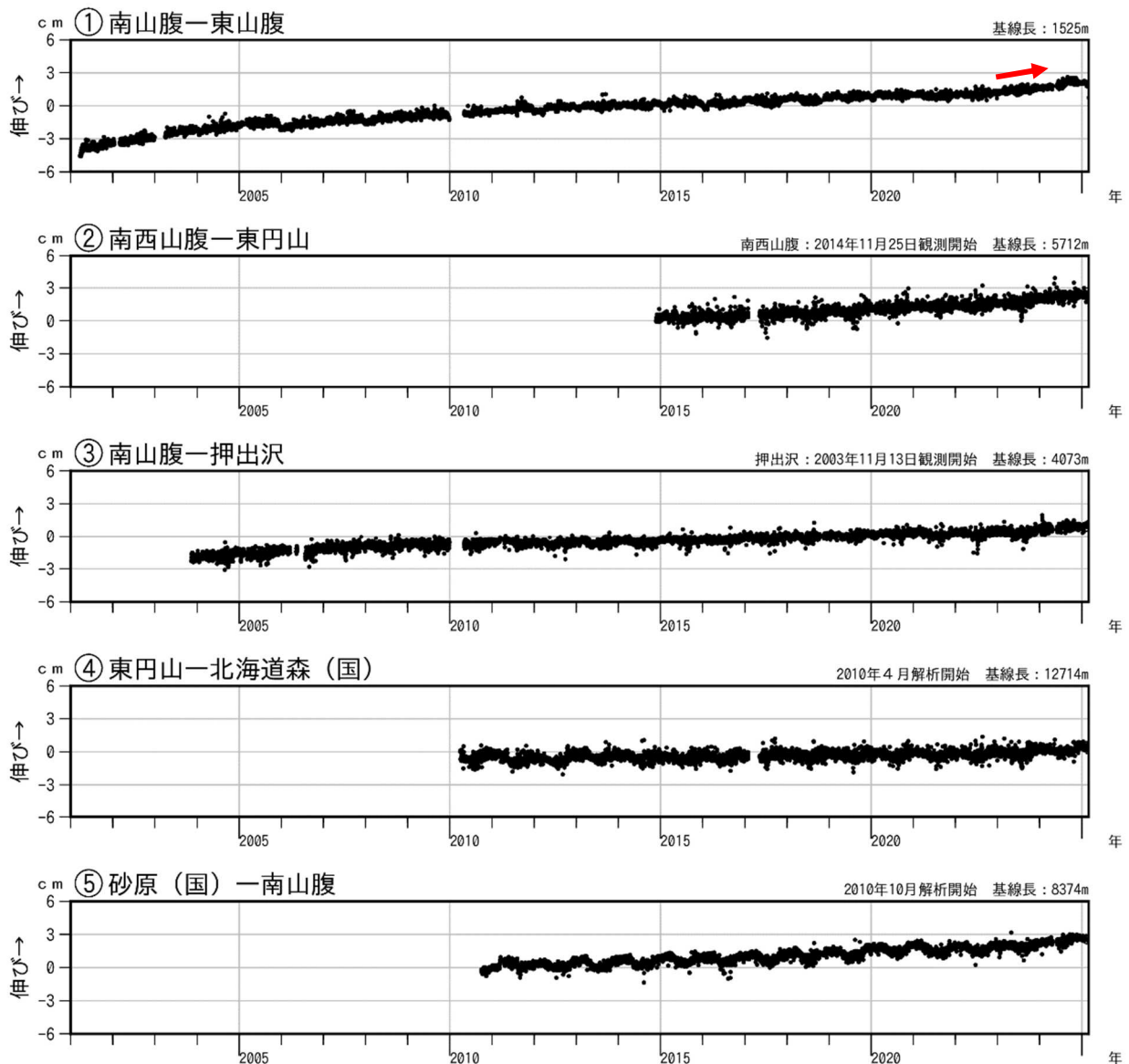
図5 北海道駒ヶ岳 GNSS連続観測による基線長変化（2001年4月～2025年2月） グラフ①～⑤は図6の観測点配置図の基線①～⑤に対応しています。 グラフの空白部分は欠測を示します。
