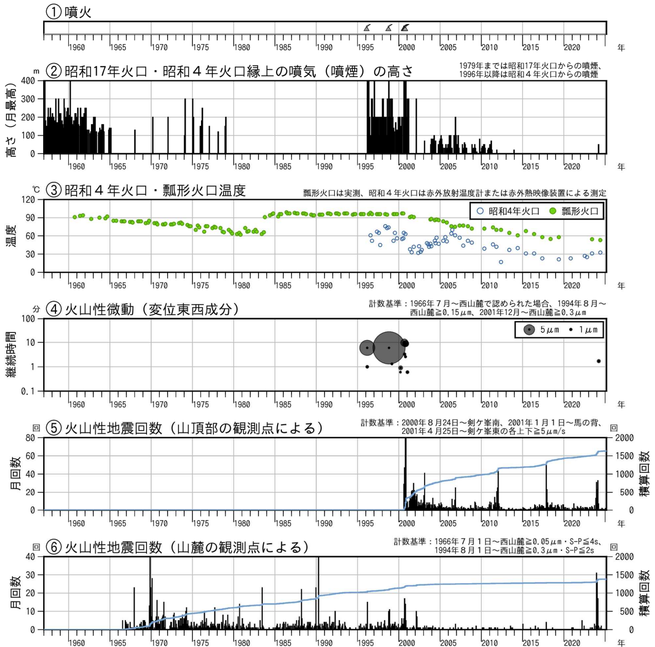
図1 北海道駒ヶ岳 火山活動経過図（1957年1月～2025年2月） 各火口の位置は図7、図8を参照してください。
