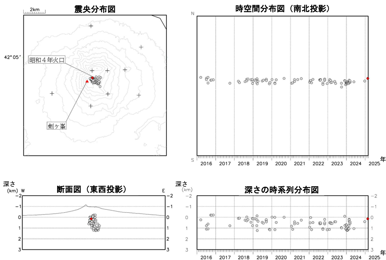
図4 北海道駒ヶ岳 火山性地震の震源分布（2016年1月～2025年2月）
