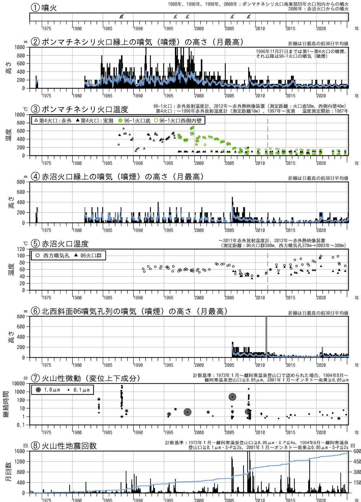
図4 雌阿寒岳 火山活動経過図（1973年1月～2025年3月）
