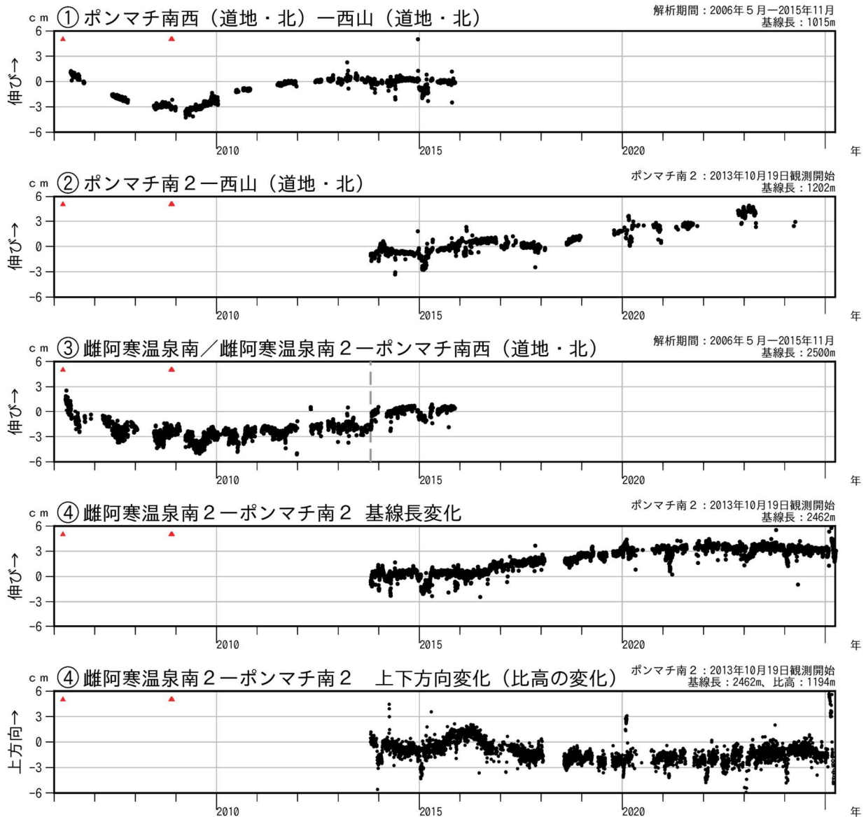
図7-1 雌阿寒岳 GNSS連続観測による基線長及び比高の変化（2006年4月～2025年3月）
