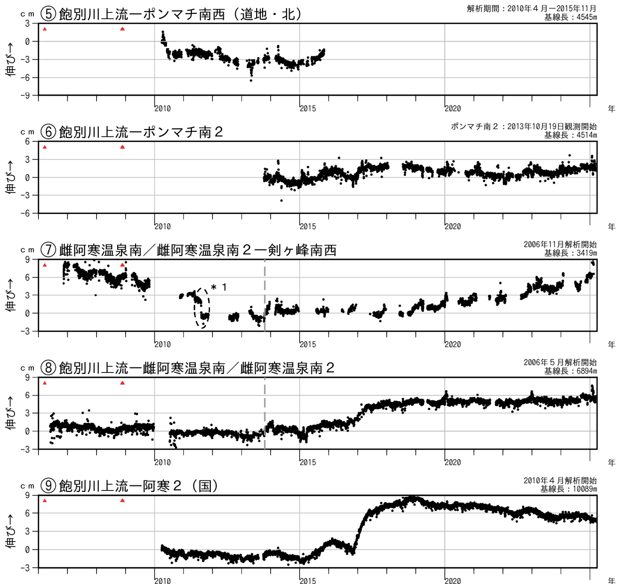
図7-2 雌阿寒岳 GNSS連続観測による基線長の変化（2006年 4 月～2025年 3 月）
