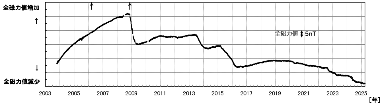
図5 雌阿寒岳 ポンマチネシリ96-1火口の噴気（噴煙）の長さや全磁力値の経過及び全磁力観測点配置図（2003年～2025年3月）
