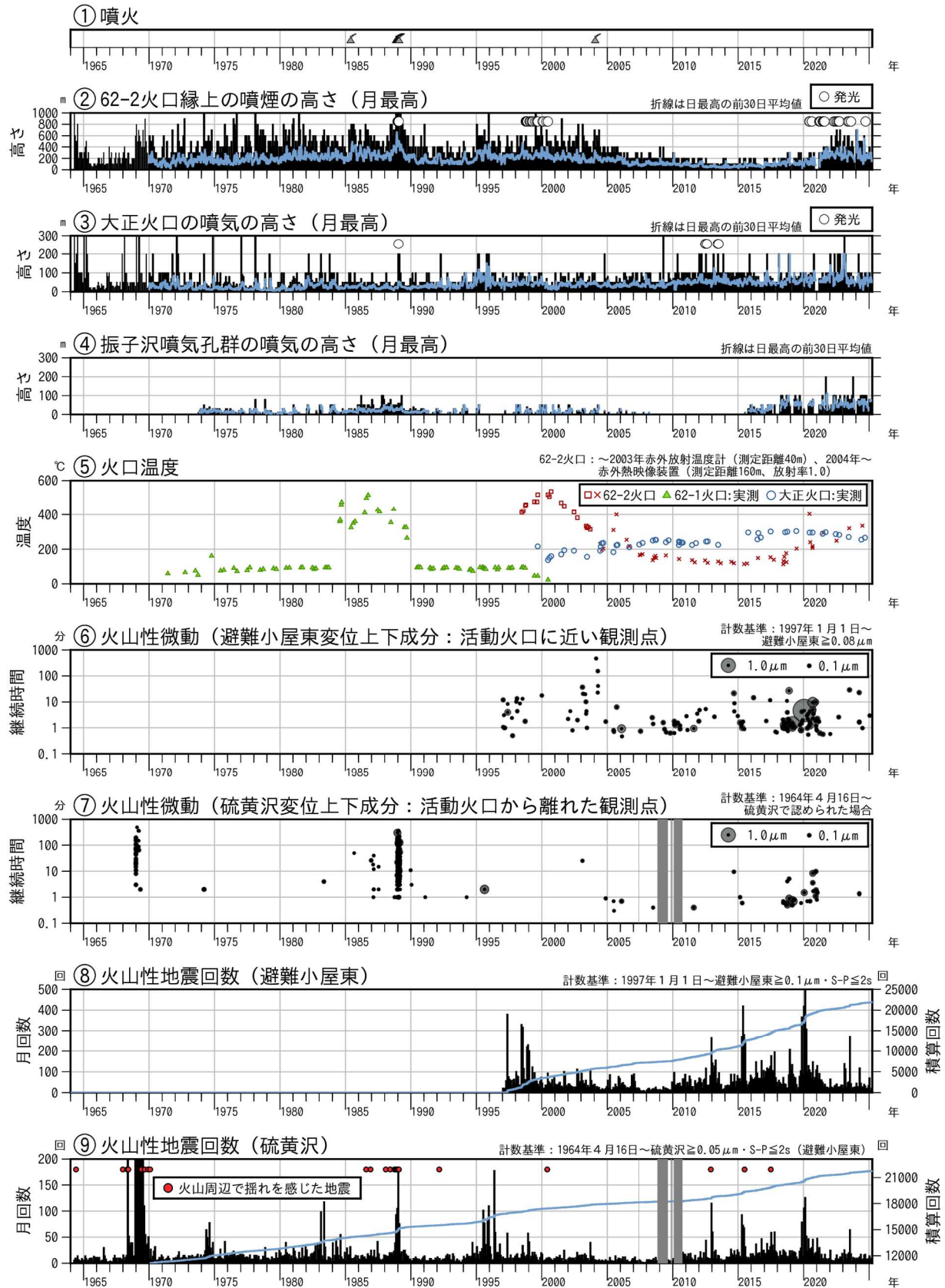
図1 十勝岳 火山活動経過図（1964年1月～2025年3月）
