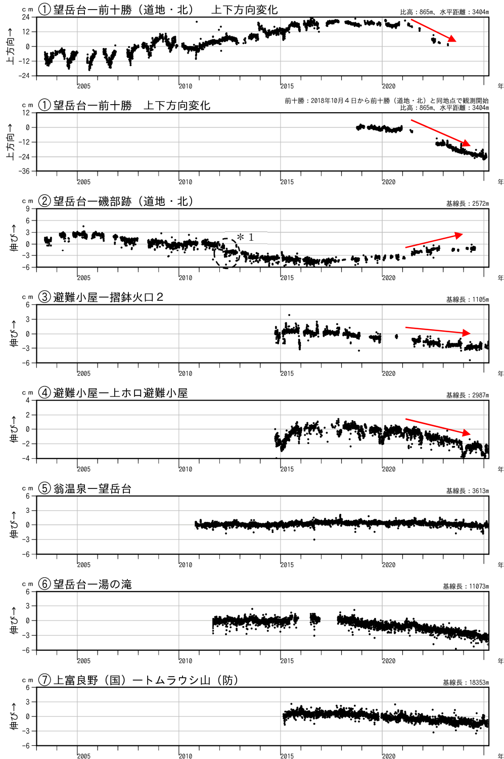
図5 十勝岳 GNSS連続観測による上下方向変化及び基線長変化（2003年5月～2025年3月）
