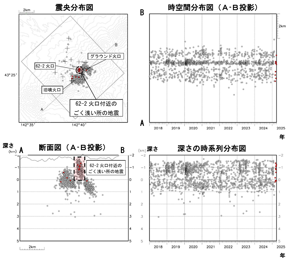
図4 十勝岳 火山性地震の震源分布（2018年1月～2025年3月）
