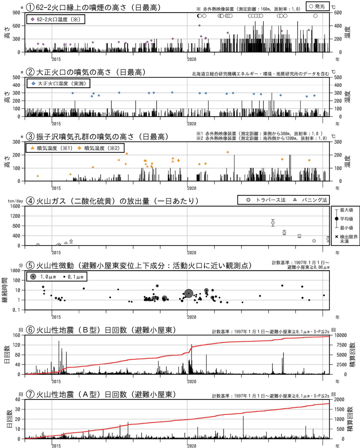
図2 十勝岳 火山活動経過図（2014年1月～2025年3月）
