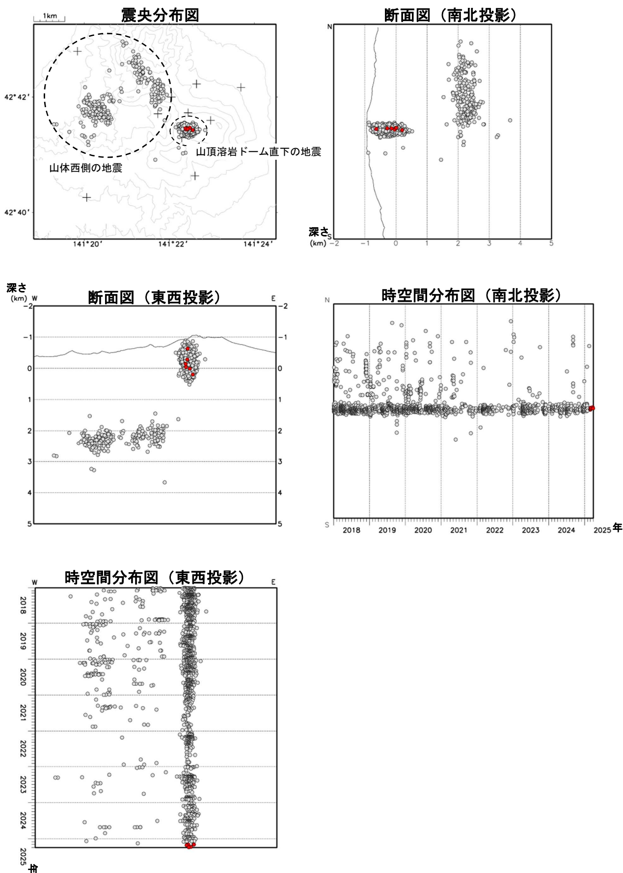
図3 樽前山 火山性地震の震源分布（2018年1月～2025年3月）
