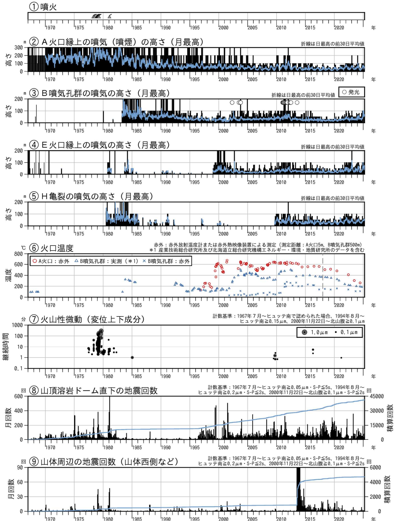
図2 樽前山 火山活動経過図（1967年1月～2025年3月）
