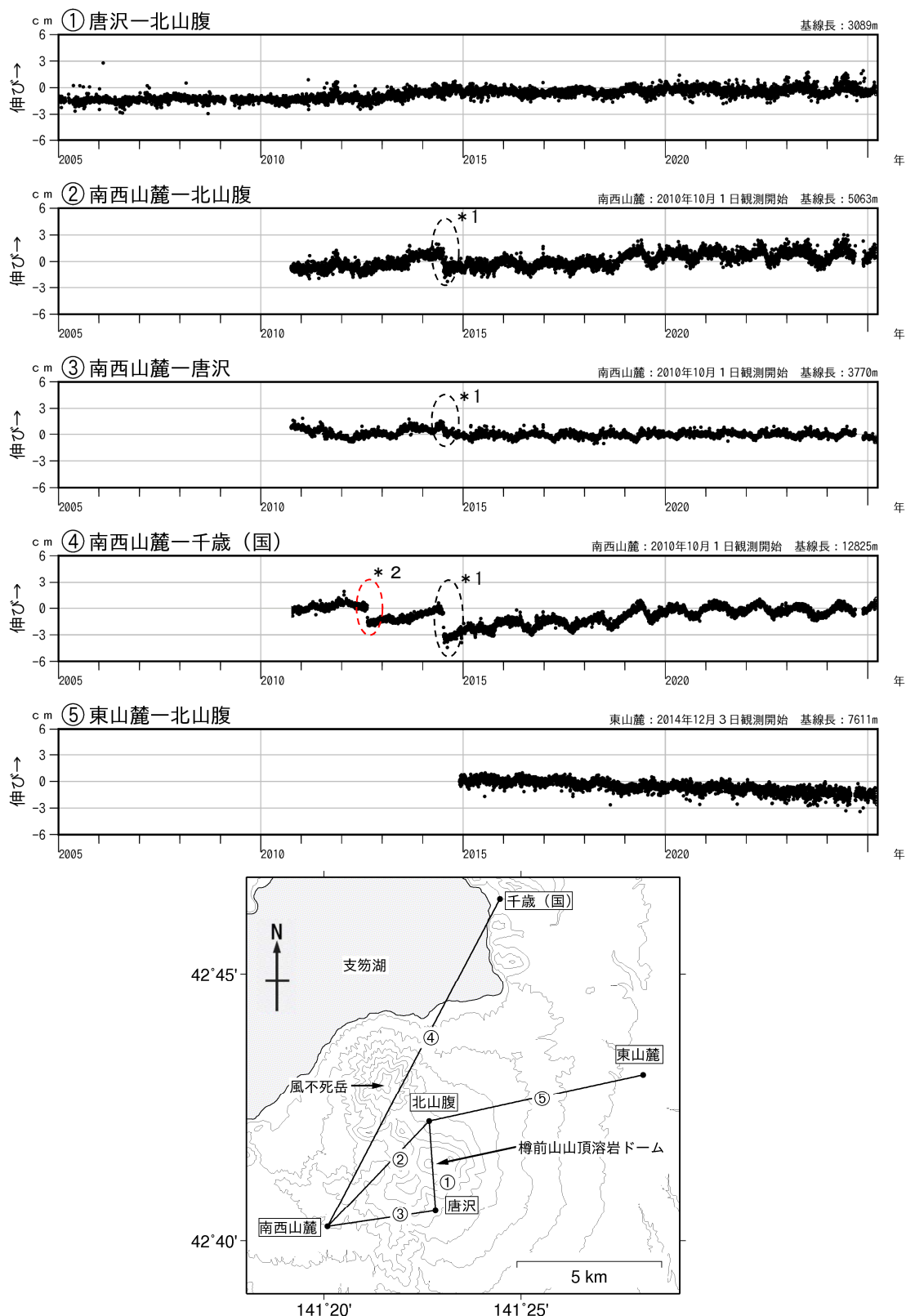
図 4 樽前山 GNSS連続観測による基線長変化（2005年1月～2025年3月）及び観測点配置図 グラフ①～⑤は観測点配置図の基線①～⑤に対応しています。 グラフ中の空白部分は欠測を示しています。
