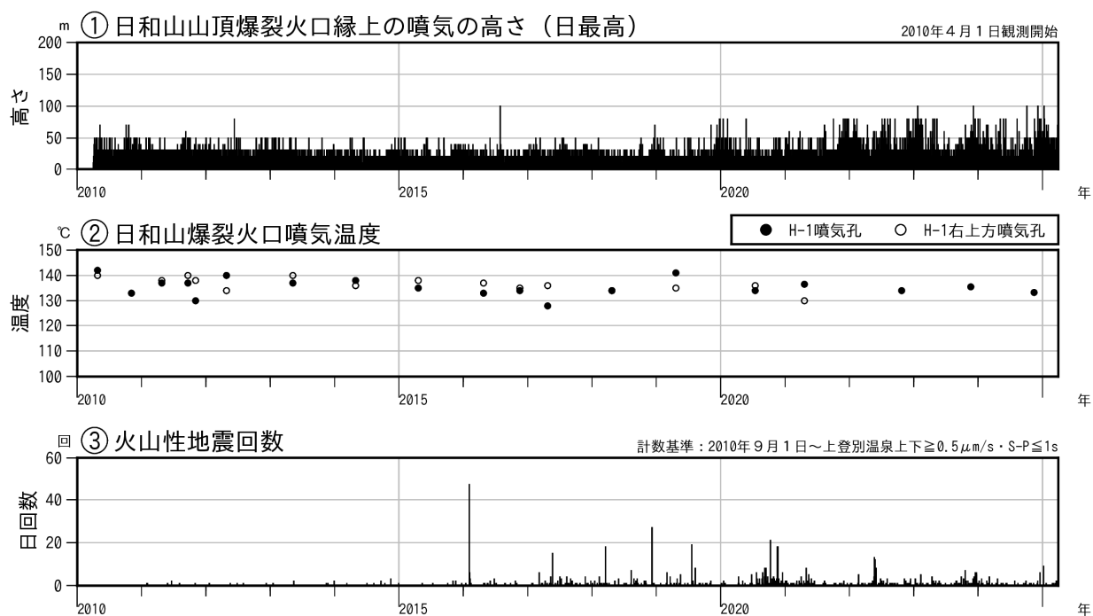
図 2 倶多楽 火山活動経過図（2010年 1 月～2025年 3 月）
