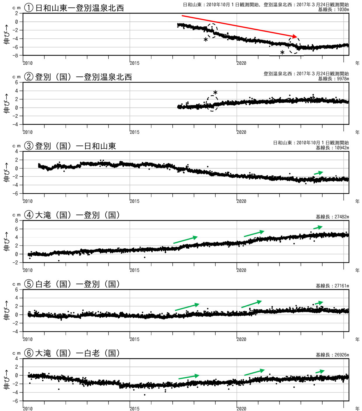
図3 倶多楽 GNSS連続観測による基線長変化（2010年4月～2025年3月）
