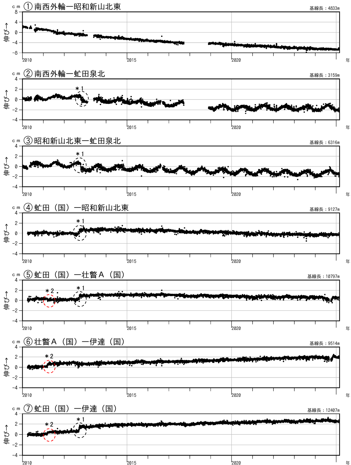
図4 有珠山 GNSS連続観測による基線長変化（2010年1月～2025年3月）
