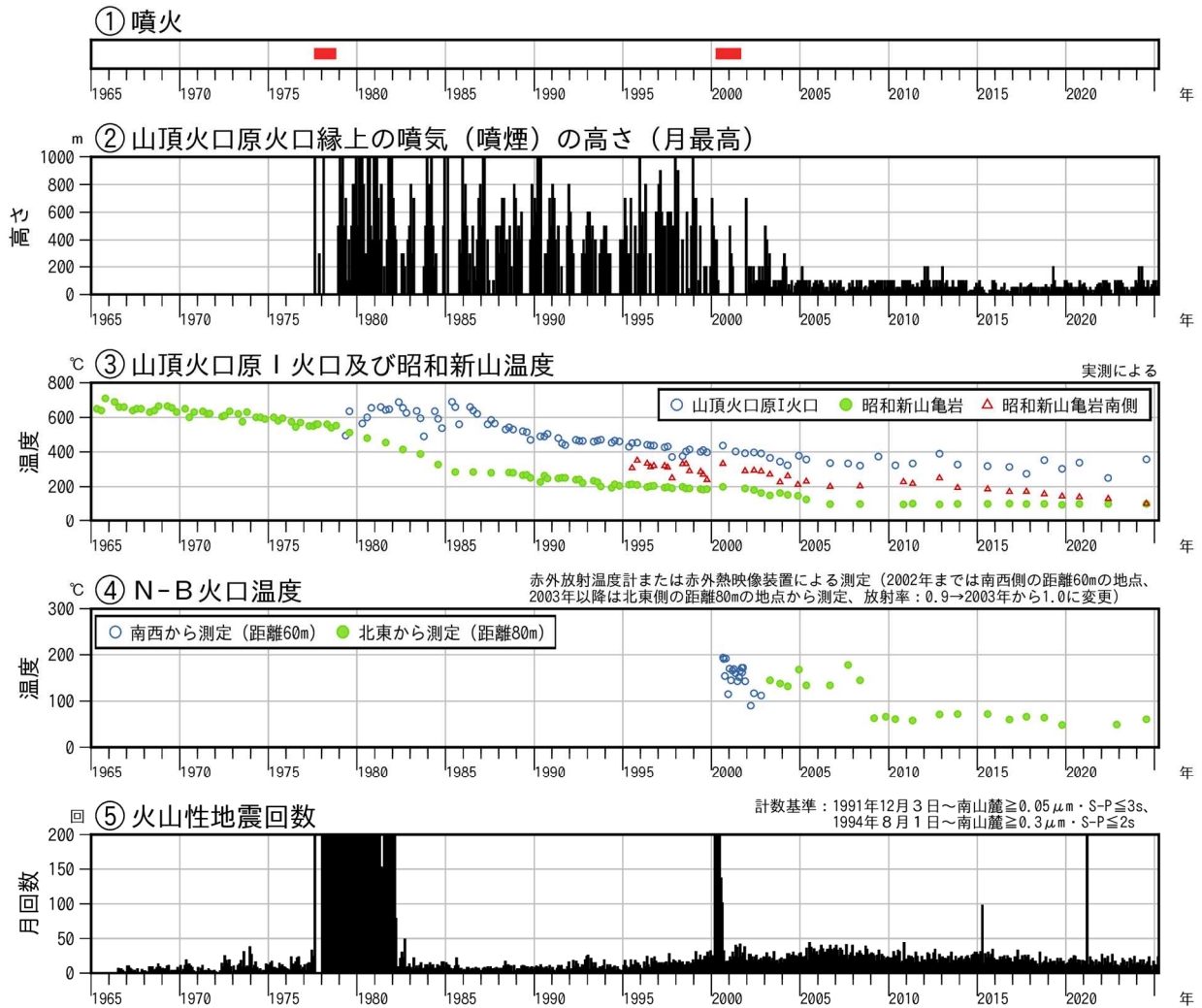
図1 有珠山 火山活動経過図（1965年1月～2025年3月）
