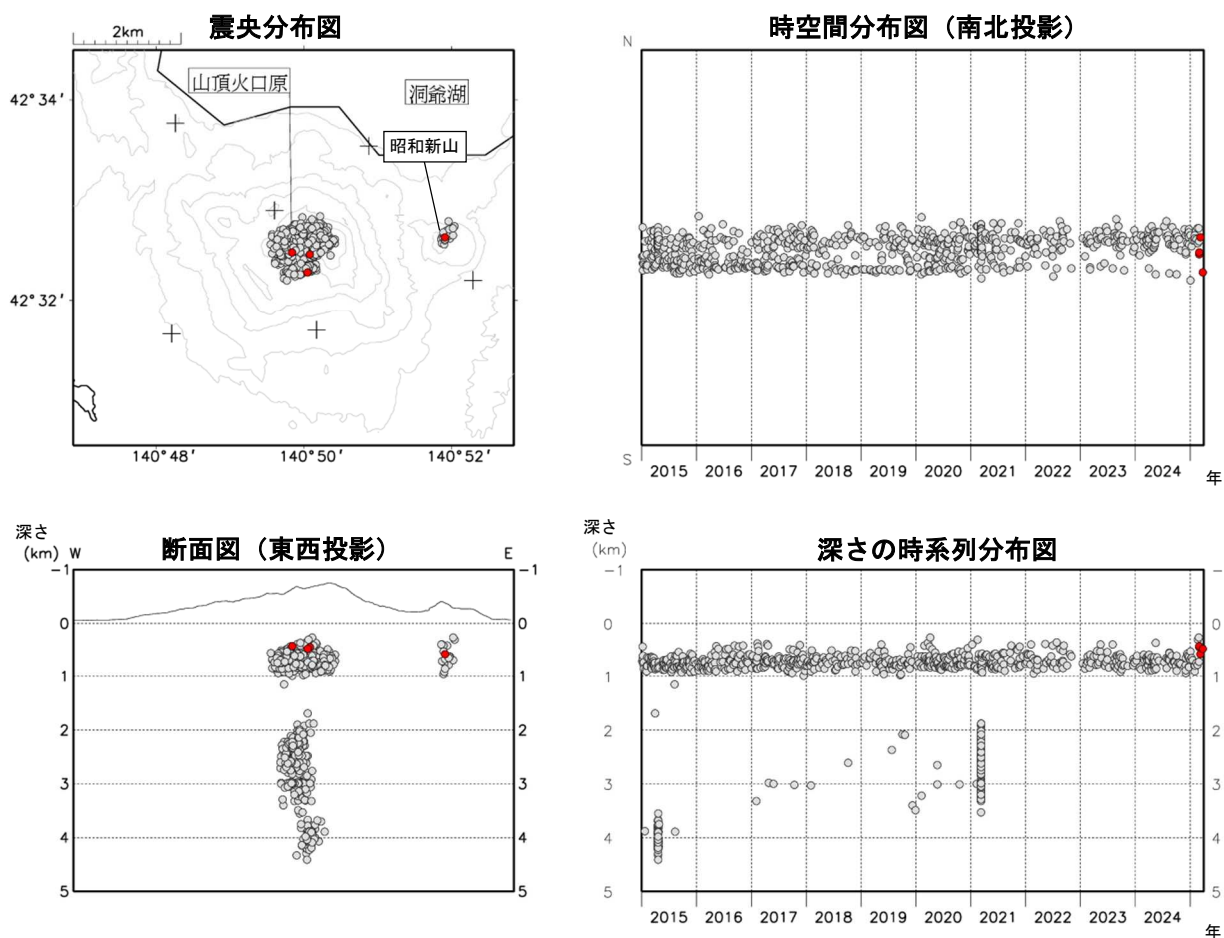
図3 有珠山 火山性地震の震源分布（2015年1月～2025年3月）
