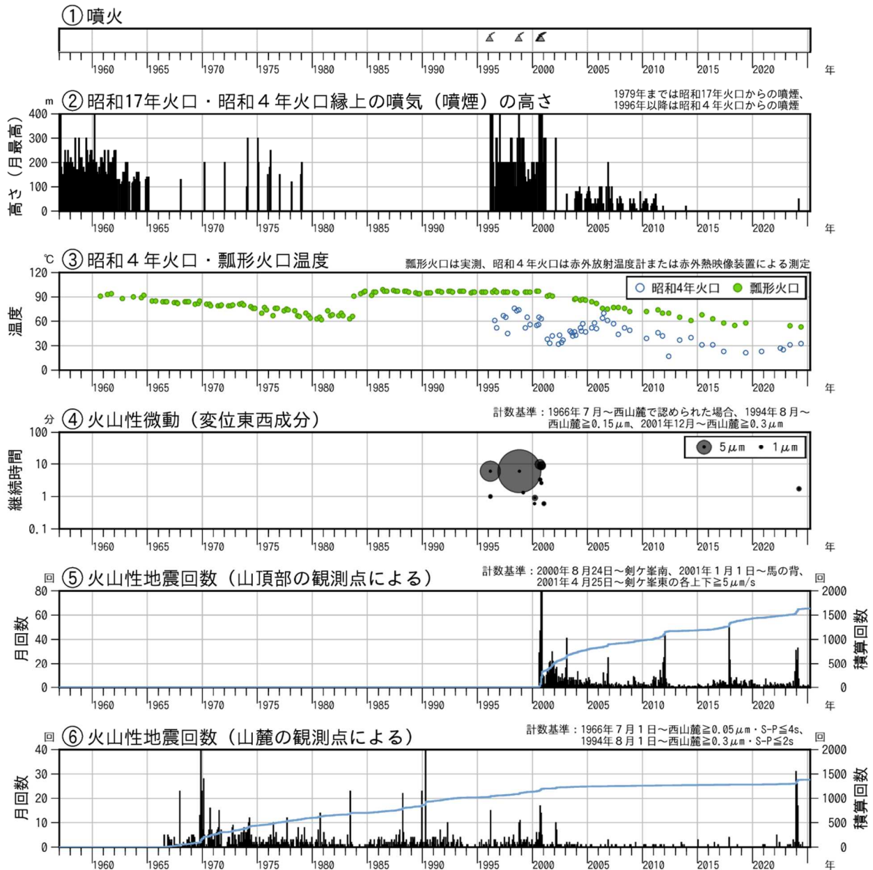
図1 北海道駒ヶ岳 火山活動経過図（1957年1月～2025年3月） 各火口の位置は図7、図8を参照してください。
