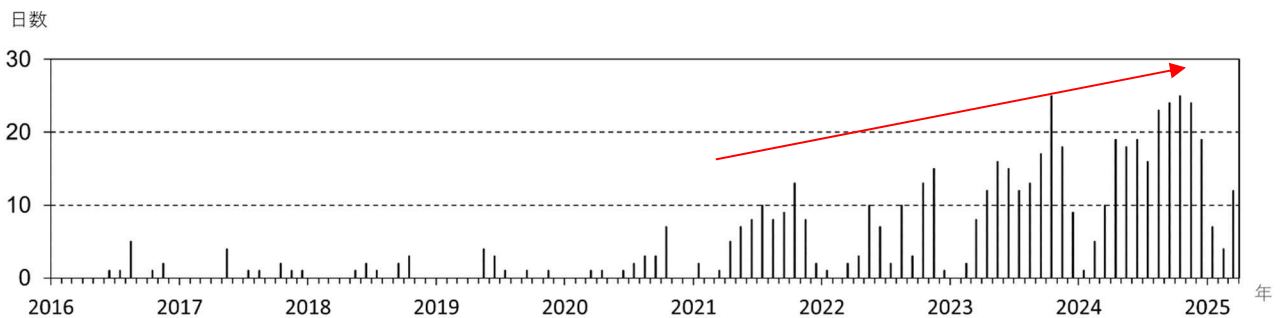
図2 北海道駒ヶ岳 昭和4年火口のごく弱い噴気を観測した日数（2016年1月～2025年3月） 山頂部に設置した剣ヶ峰監視カメラ及び駒ヶ岳山頂（道）監視カメラ（位置は図7、 図8参照）による観測結果です。 冬季は雪氷付着のため欠測日が多くなる傾向があります。
