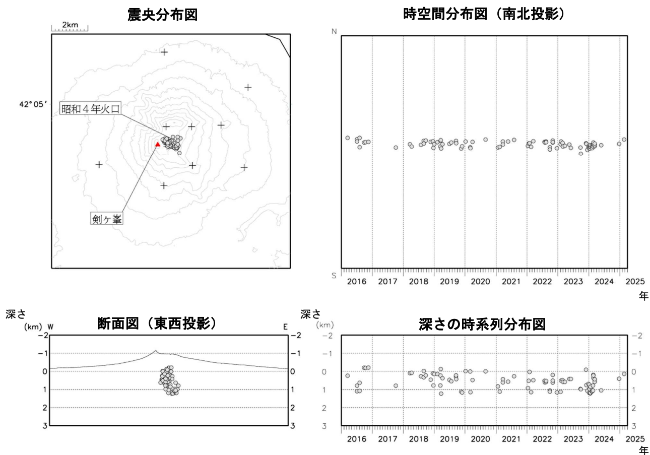
図4 北海道駒ヶ岳 火山性地震の震源分布（2016年1月～2025年3月）
