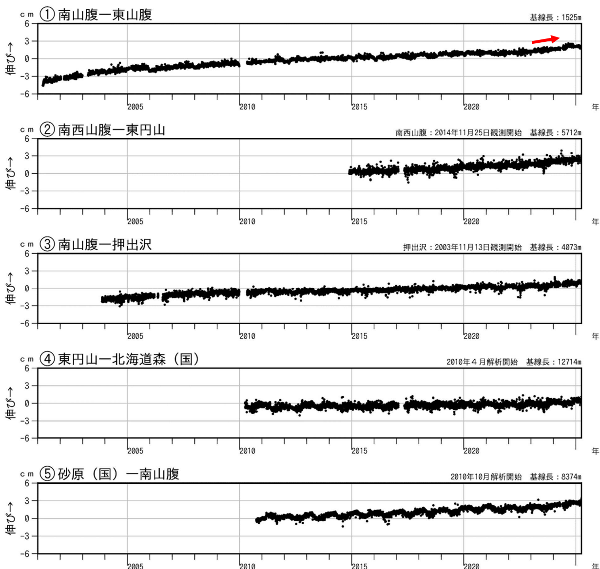
図5 北海道駒ヶ岳 GNSS連続観測による基線長変化（2001年4月～2025年3月） グラフ①～⑤は図6の観測点配置図の基線①～⑤に対応しています。 グラフの空白部分は欠測を示します。
