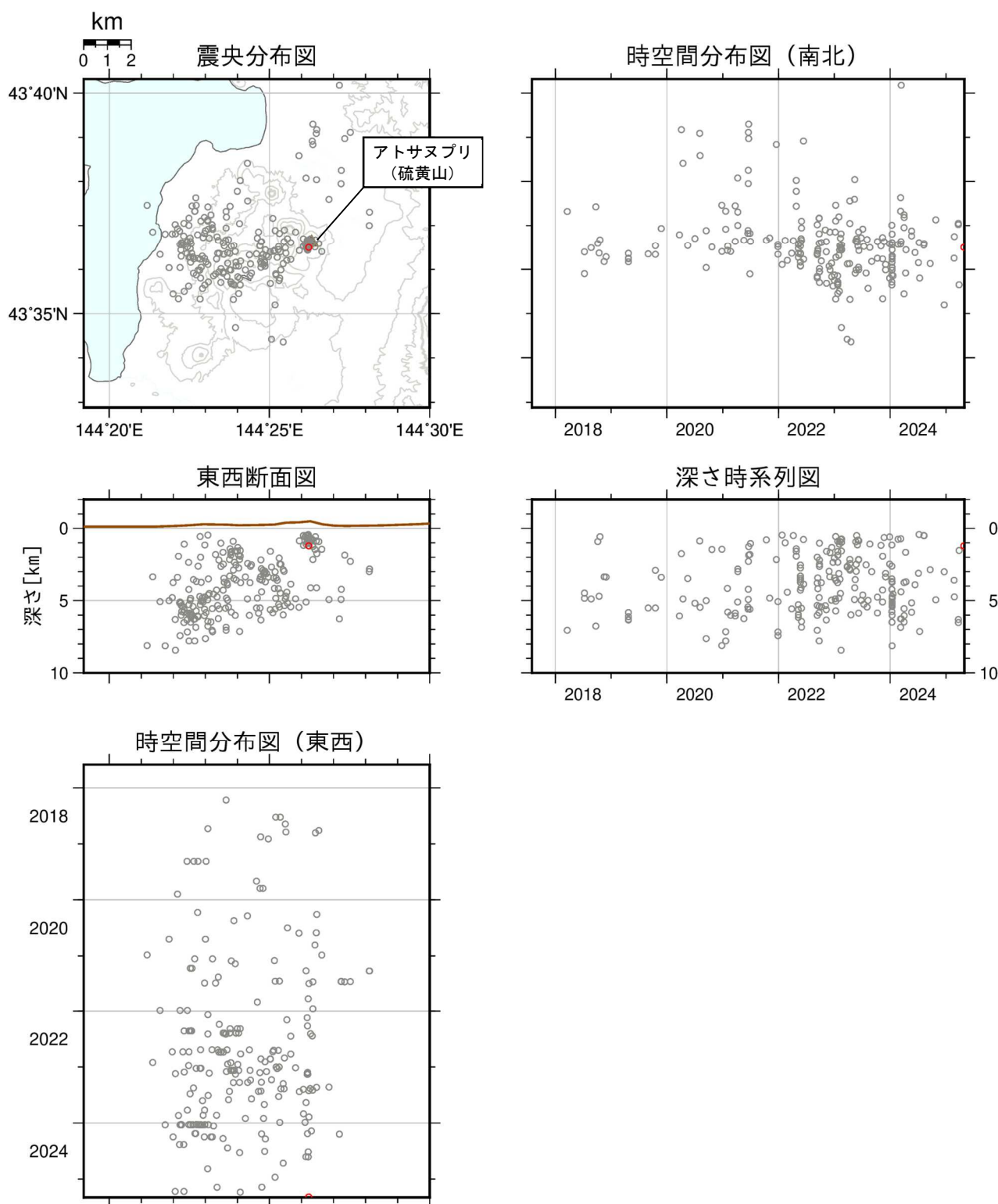
図3 アトサヌプリ 火山性地震の震源分布（2017年8月～2025年4月） ○：2017年8月～2025年3月の震源 ○：2025年4月の震源
