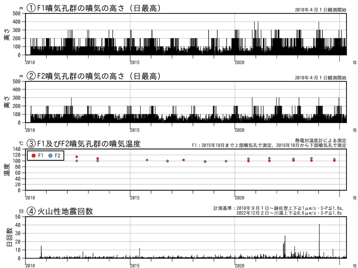
図1 アトサヌプリ 火山活動経過図（2010年4月～2025年4月）
