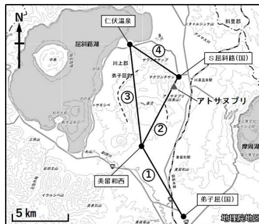
図4 アトサヌプリ GNSS連続観測による基線長変化（2010年10月～2025年4月）及び観測点配置図
