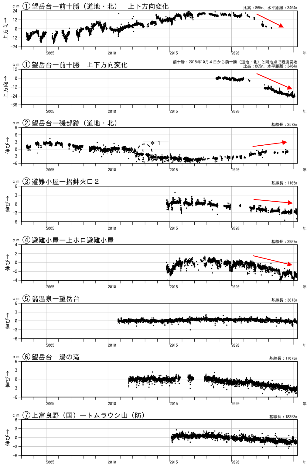
図5 十勝岳 GNSS連続観測による上下方向変化及び基線長変化（2003年5月～2025年4月）
