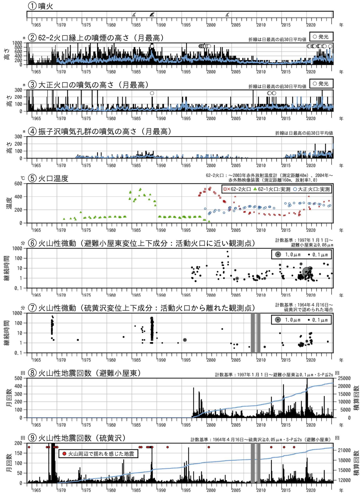
図1 十勝岳 火山活動経過図（1964年1月～2025年4月）
