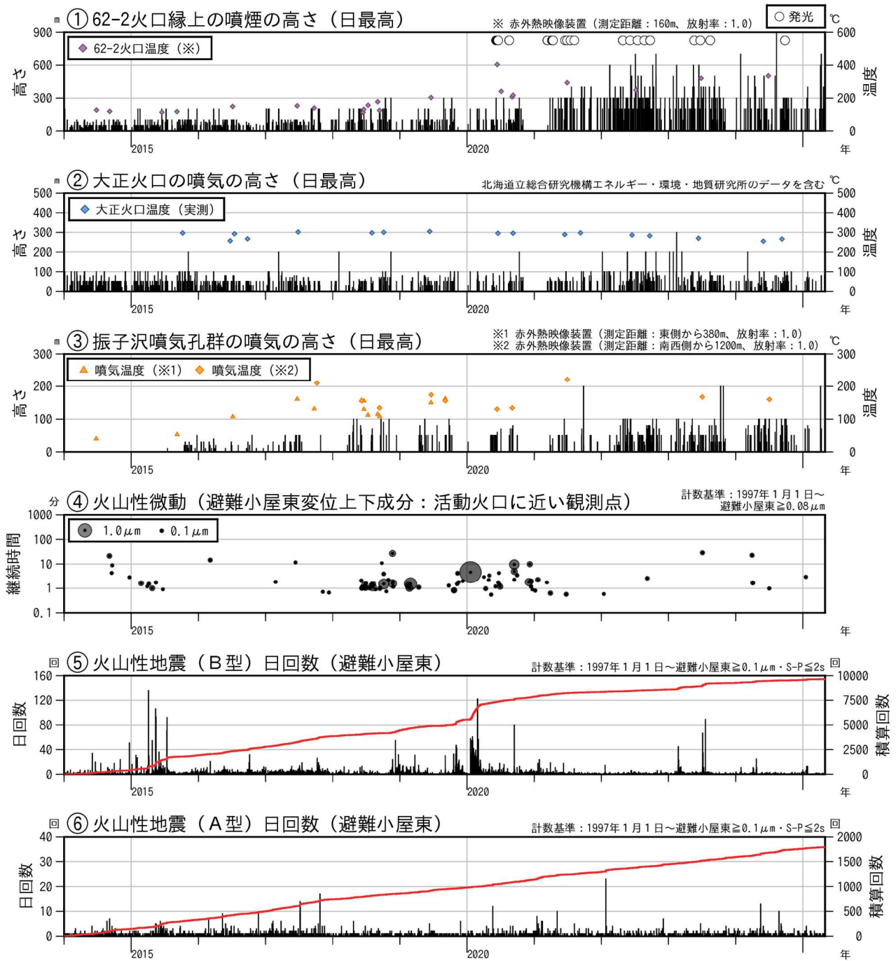
図2 十勝岳 火山活動経過図（2014年1月～2025年4月）
