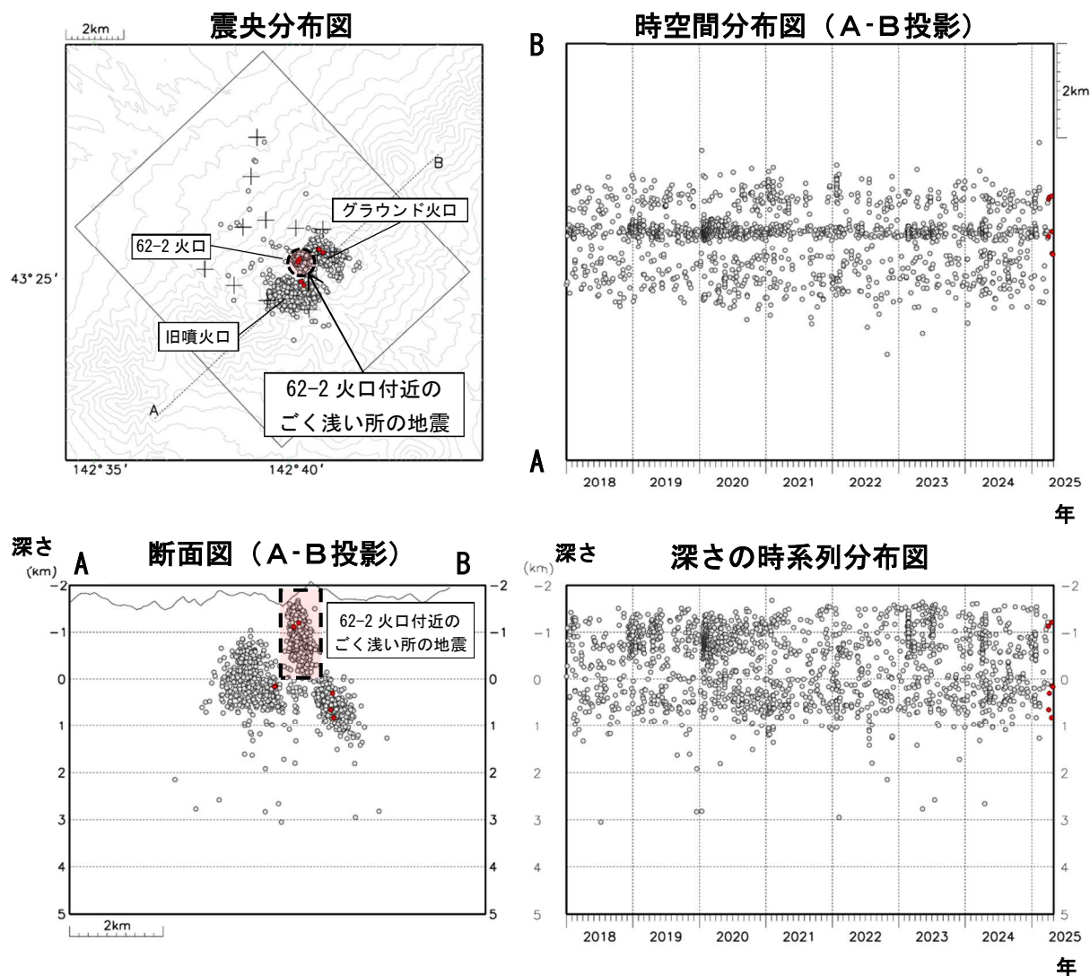
図4 十勝岳 火山性地震の震源分布（2018年1月～2025年4月） ●：2018年1月～2025年3月の震源 ●：2025年4月の震源 ＋：地震観測点
