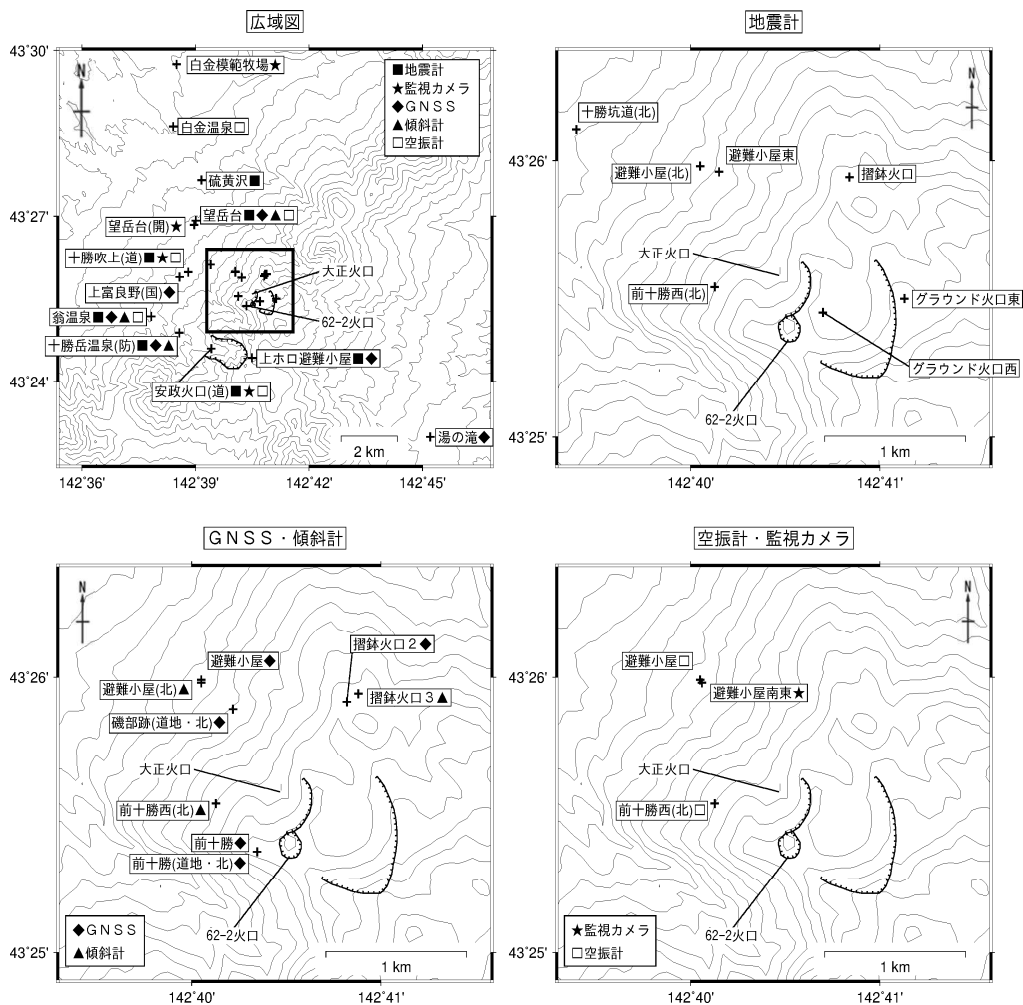
図7 十勝岳 観測点配置図
