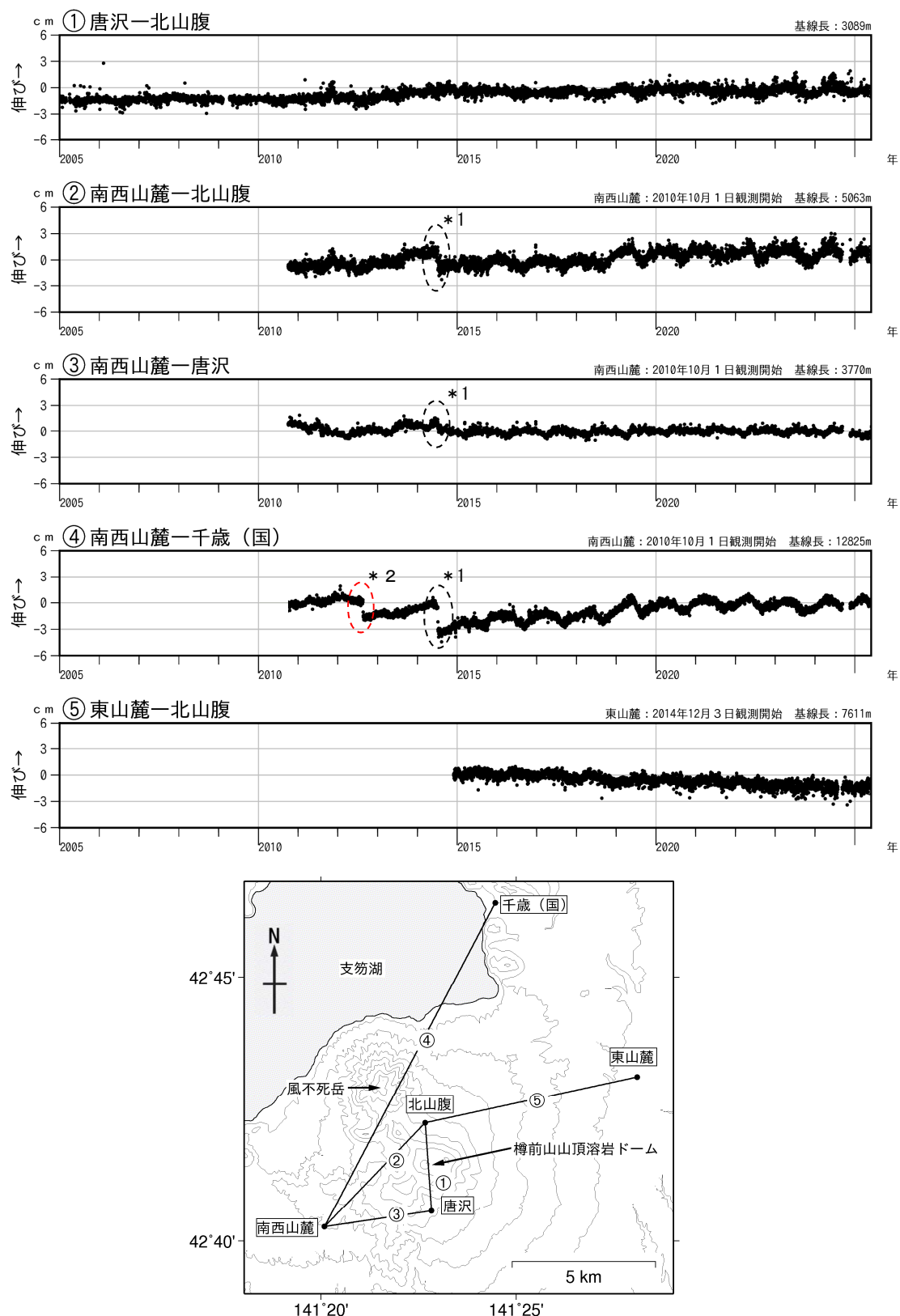
図4 樽前山 GNSS連続観測による基線長変化（2005年1月～2025年5月）及び観測点配置図
