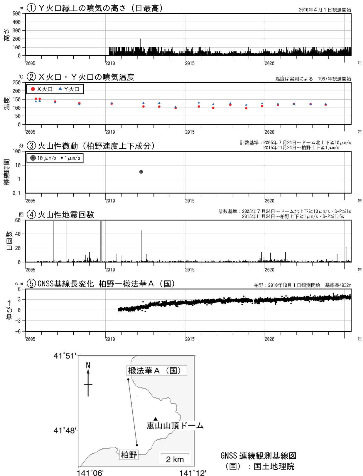
図 2 恵山 火山活動経過図（2005 年 7 月～2025 年 5 月） ④の灰色部分は機器障害による欠測期間を示します。 ⑤のグラフは上図の基線に対応しています。 ⑤のグラフの空白部分は欠測を示します。
