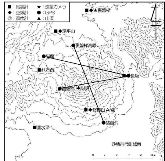
磐梯山火山観測点配置図
