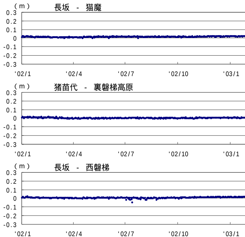
GPS 基線長変化図 (2002.01 ~ 2003.01)
