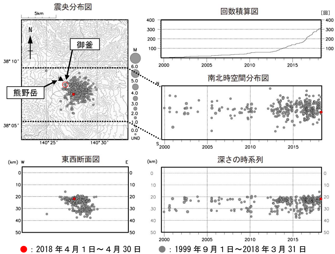
図 3 蔵王山 広域地震観測網による深部低周波地震活動（1999 年 9 月～2018 年 4 月）
