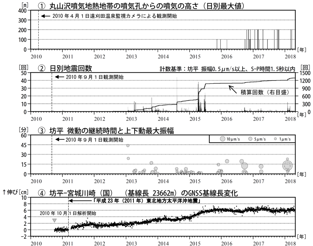
図2 蔵王山 火山活動経過図（2010年4月～2018年4月）
