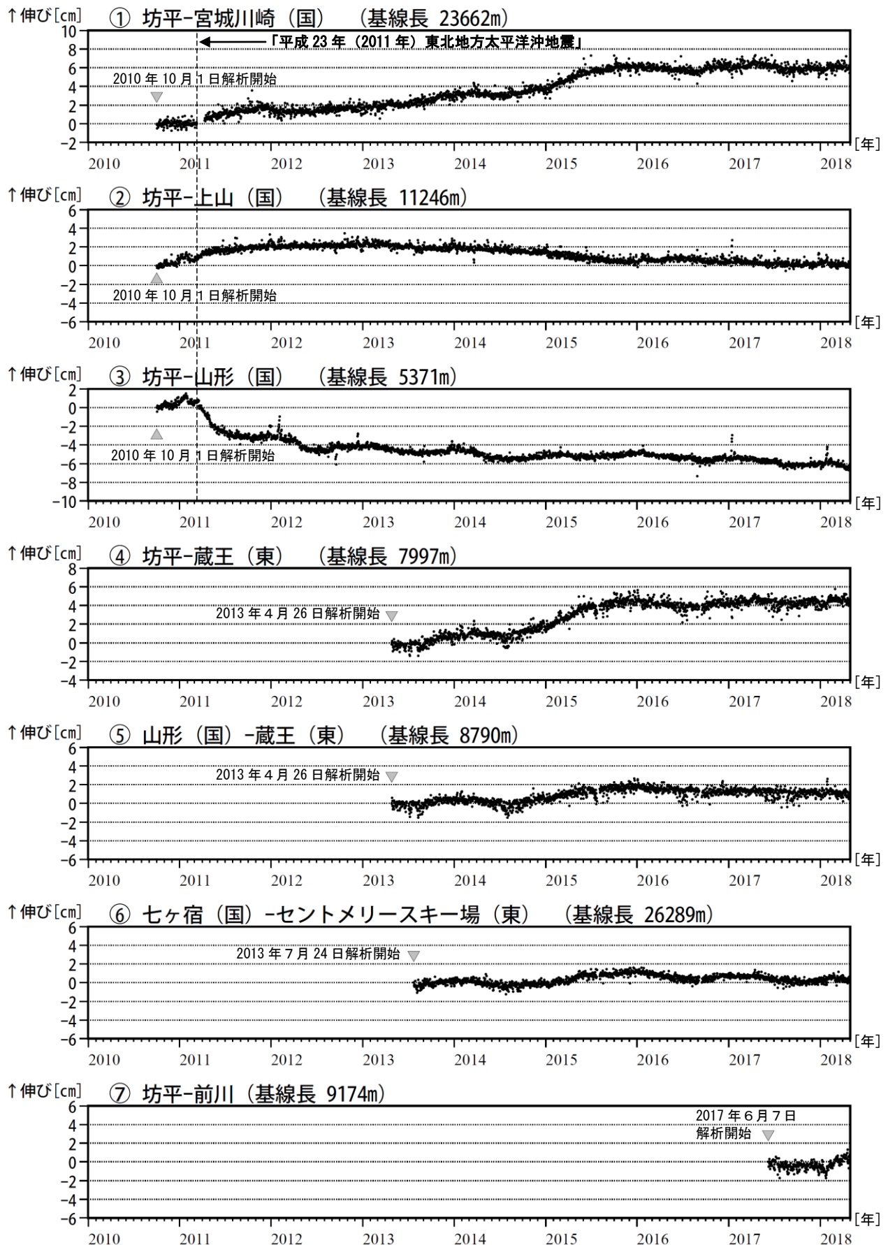
図 4 蔵王山 GNSS 基線長変化図 (2010 年 10 月～2018 年 4 月)
