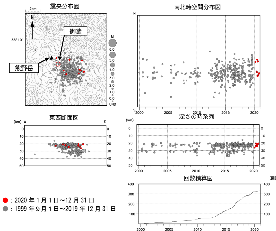
図 10 蔵王山 広域地震観測網による深部低周波地震活動（1999 年 9 月～2020 年 12 月）
