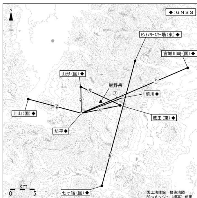
図13 蔵王山 GNSS 観測基線図
