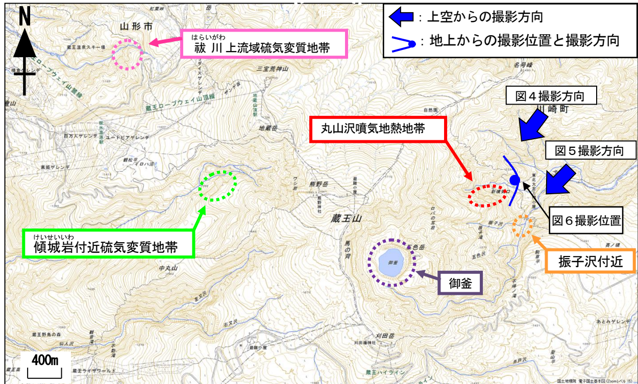
図3 蔵王山 写真と地表面温度分布撮影位置及び撮影方向
