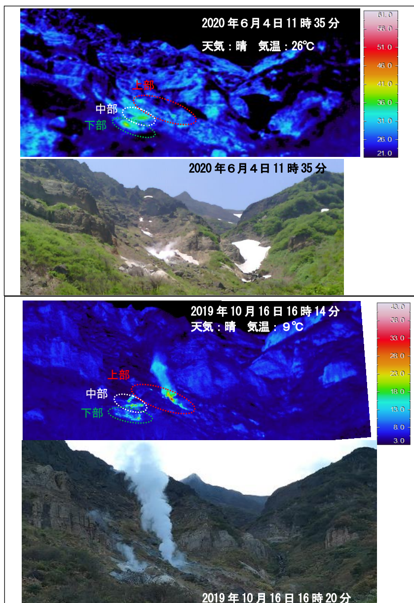
図6 蔵王山 東方向から撮影した丸山沢の状況（下段）と地表面温度分布（上段） ・地熱域以外で温度の高い部分は、岩等が日射により温められたことによるものと推定されます。
