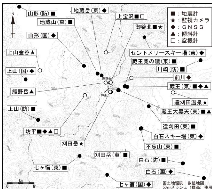
図12 蔵王山 観測点配置図
