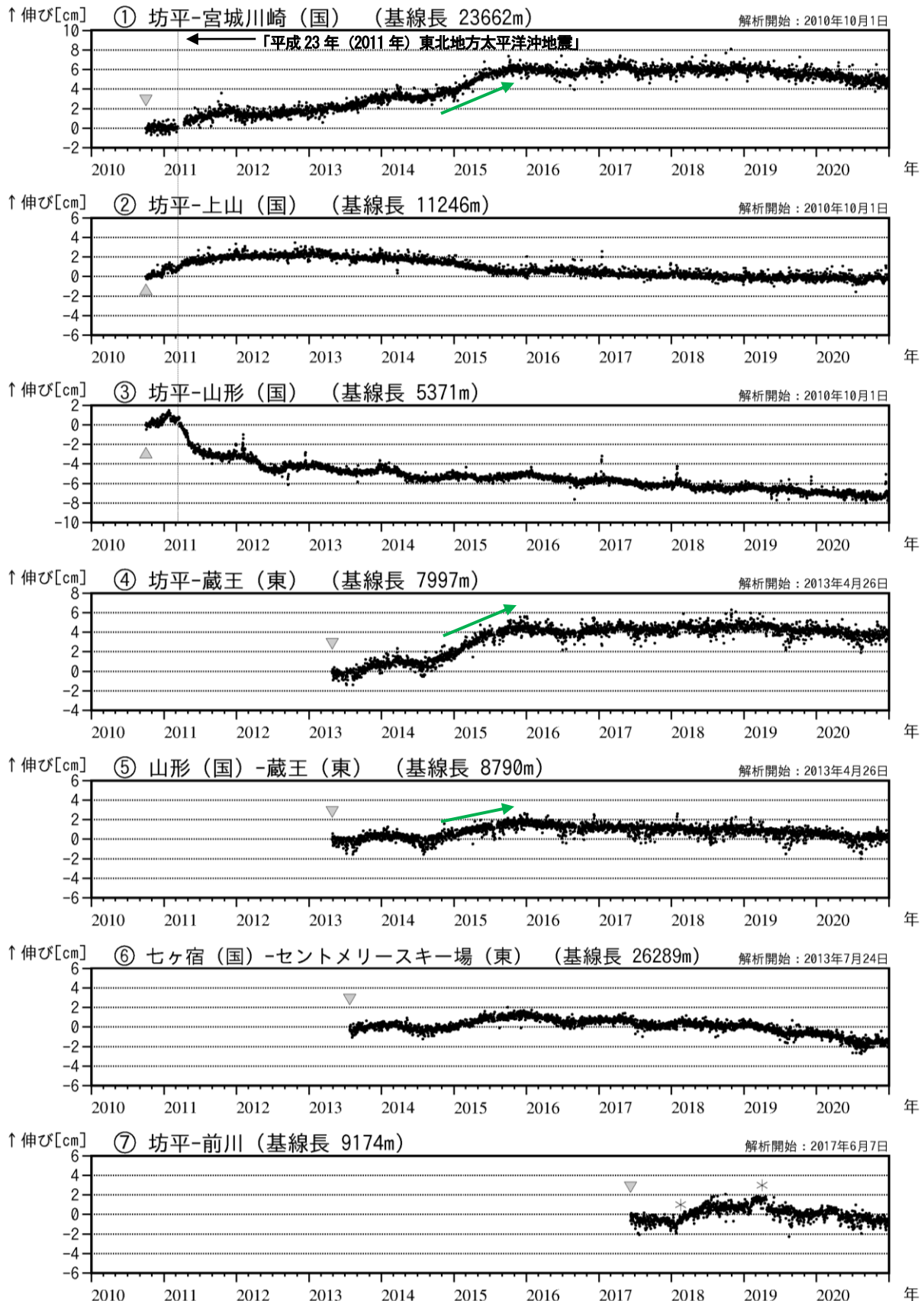
図 11 蔵王山 GNSS 基線長変化図 (2010 年 10 月～2020 年 12 月)
