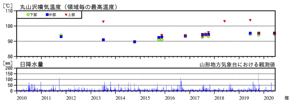
図7 蔵王山 丸山沢の噴気温度（領域毎の最高温度）の経過（2010年1月～2020年6月） ・地熱域周辺の複数地点を観測した中の最高値を示しています。
