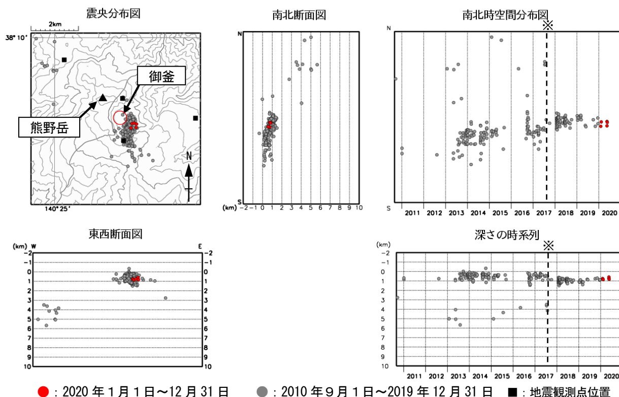
図9 蔵王山 地震活動 (2010 年 9 月 ~ 2020 年 12 月)
