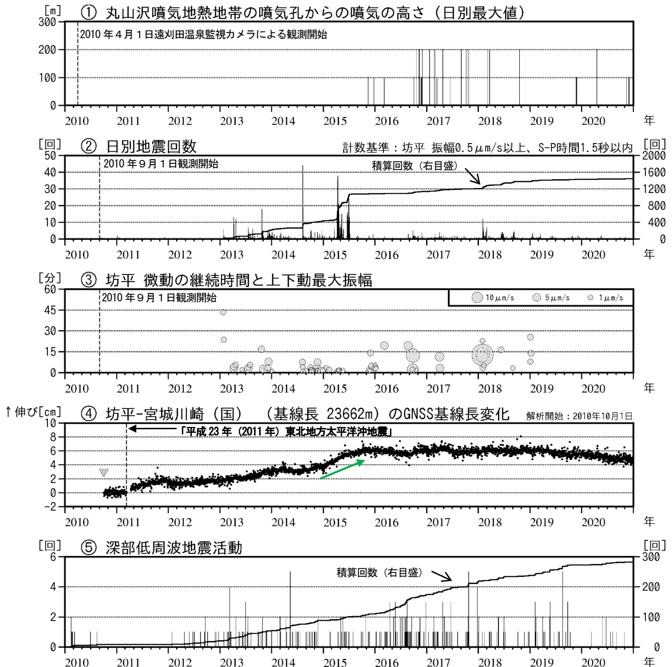
図8 蔵王山 火山活動経過図（2010年4月～2020年12月）
