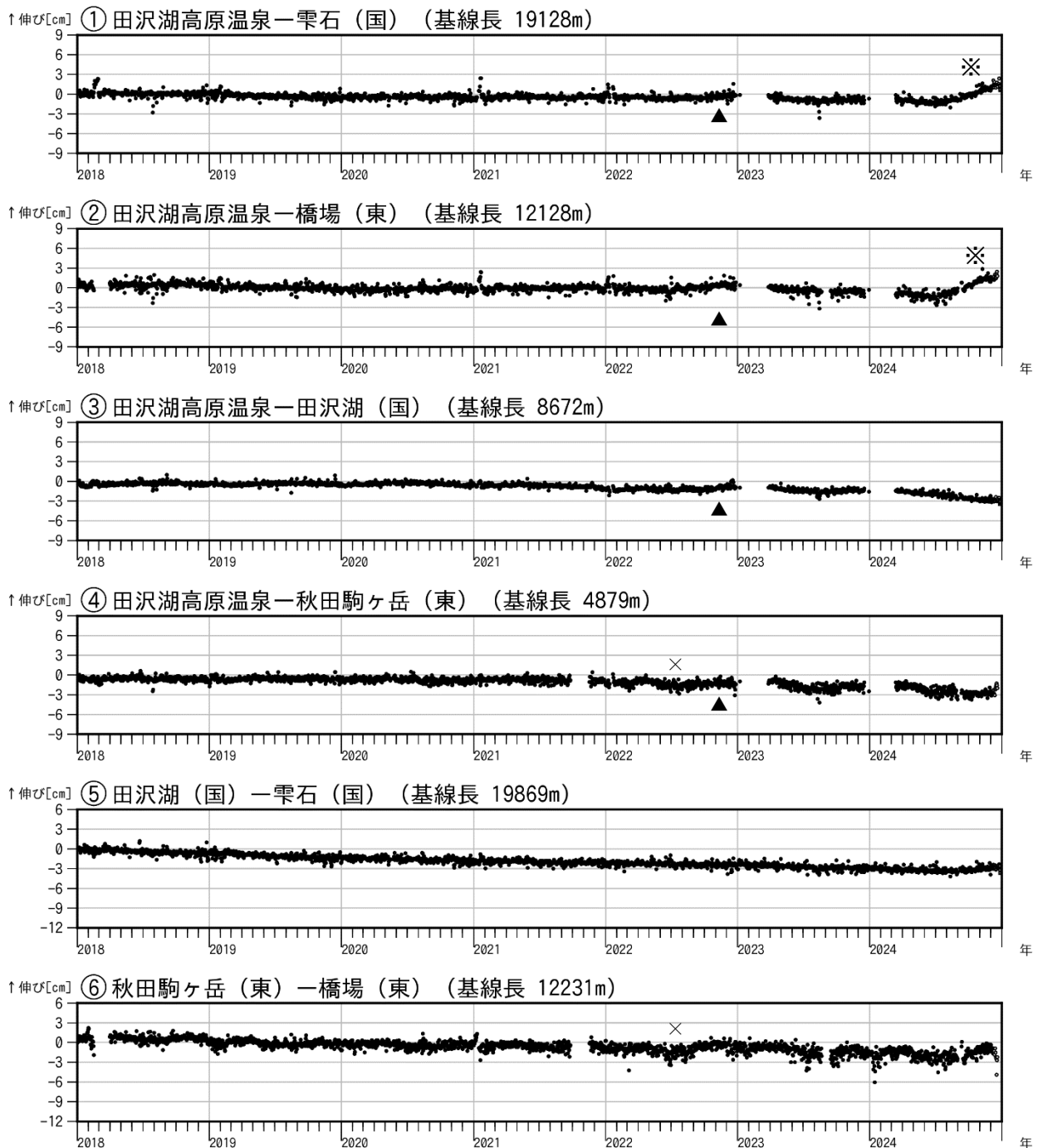
図14 秋田駒ヶ岳 GNSS 基線長変化図 (2018年1月～2024年12月)
