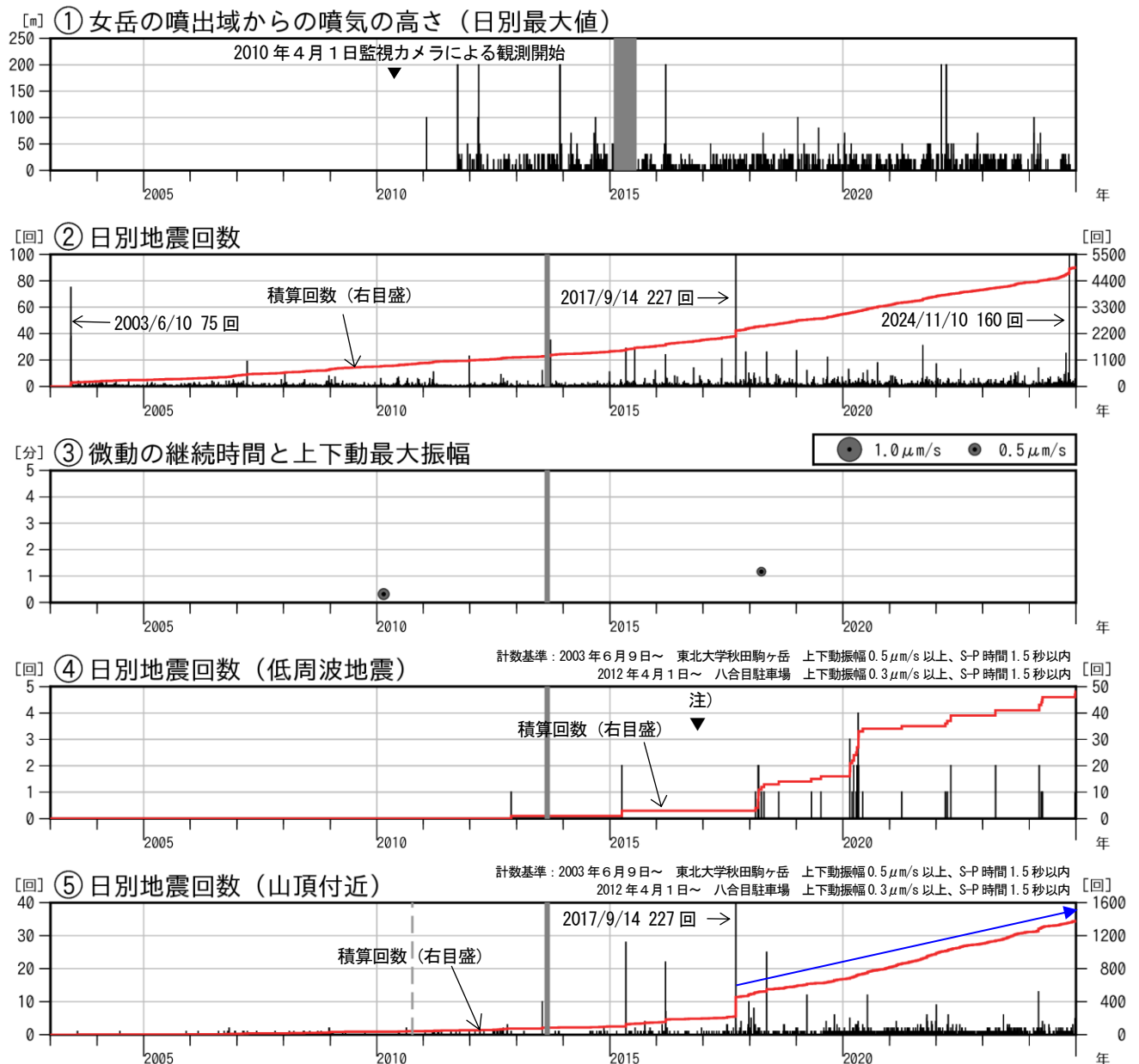
図11 秋田駒ヶ岳 火山活動経過図（2003年6月～2024年12月）
