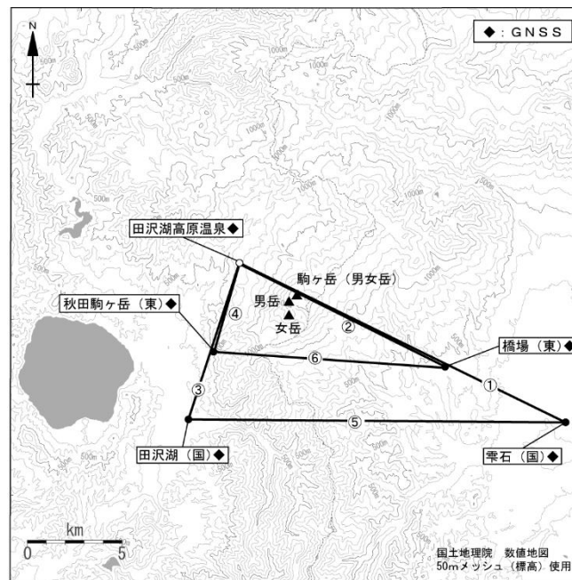
図 16 秋田駒ヶ岳 GNSS 観測基線図
