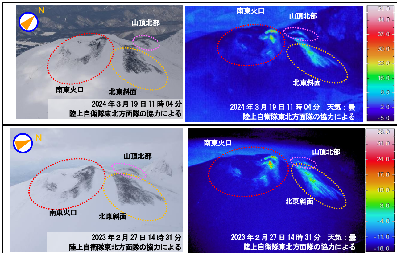
図8 秋田駒ヶ岳 上空からの南東火口の状況と地表面温度分布
