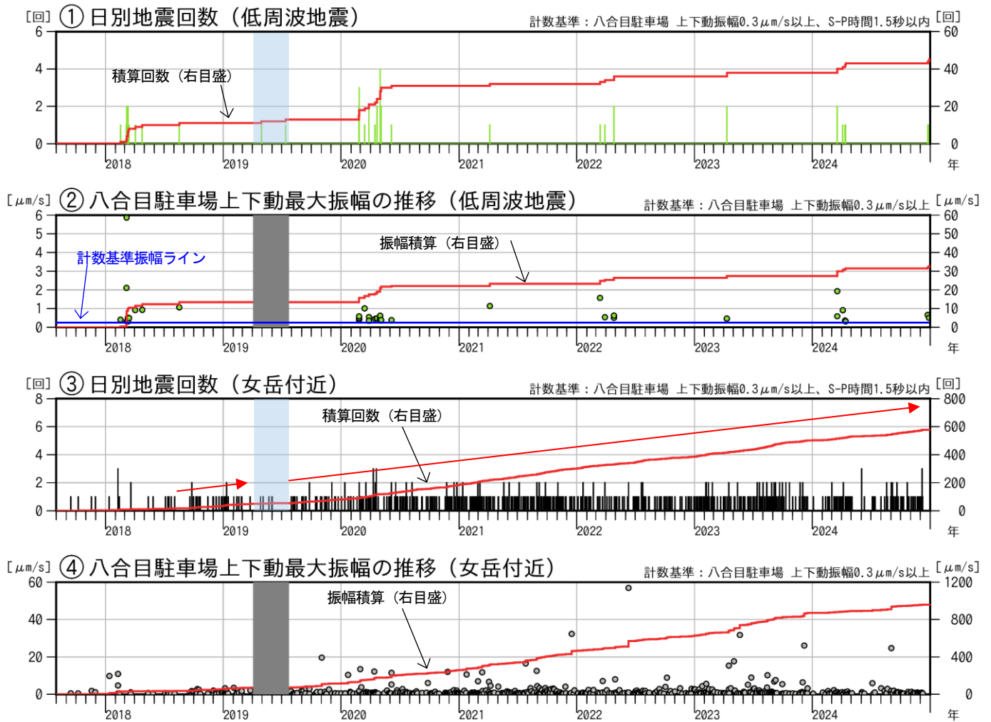
図12 秋田駒ヶ岳 低周波地震及び女岳付近の日別回数と最大振幅（2017年8月～2024年12月）
