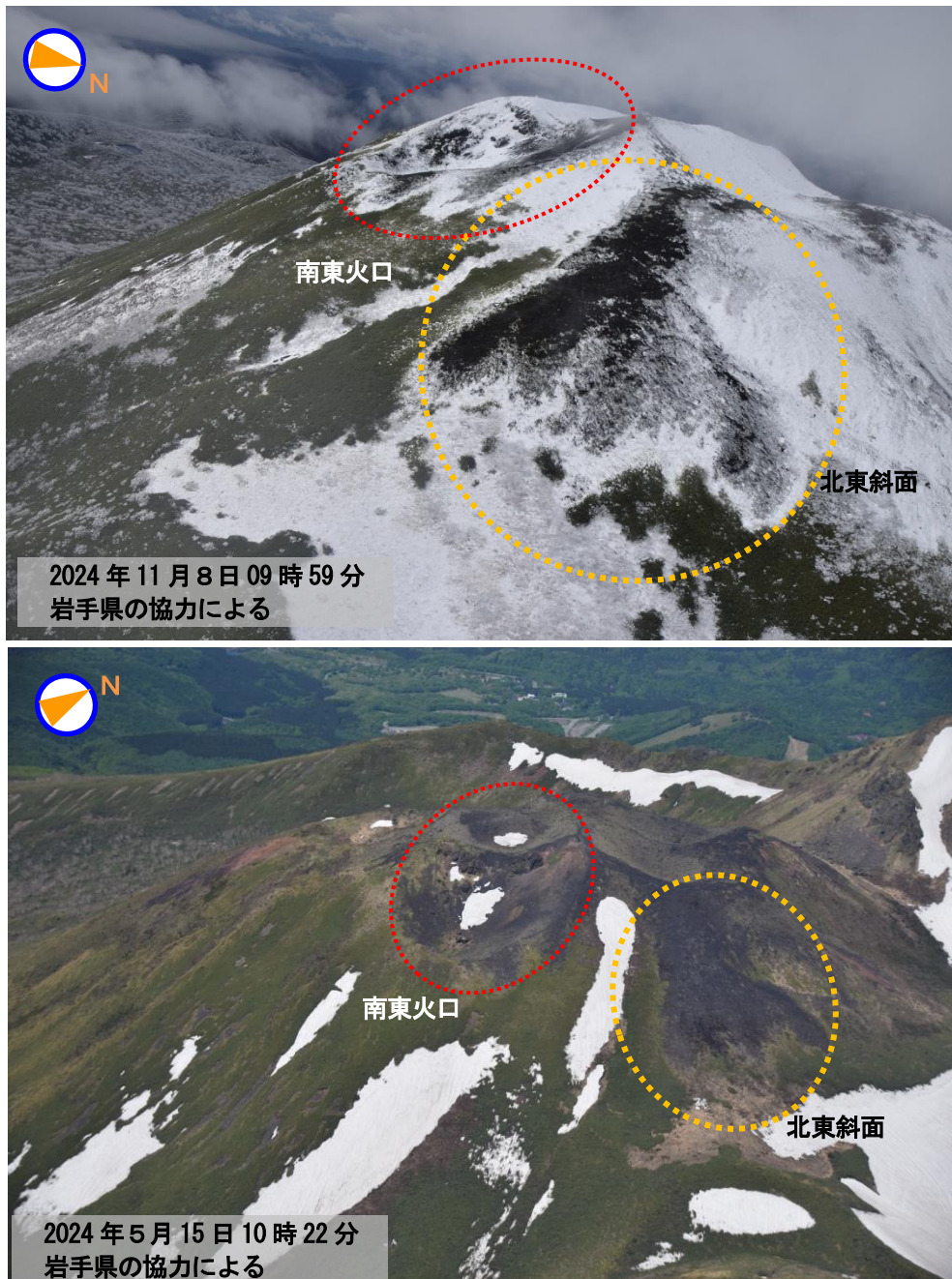
図6 秋田駒ヶ岳 上空からの南東火口及び北東斜面の状況
