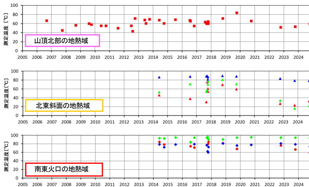
図10 女岳の地熱域における地中温度 (2006年9月～2024年11月)
