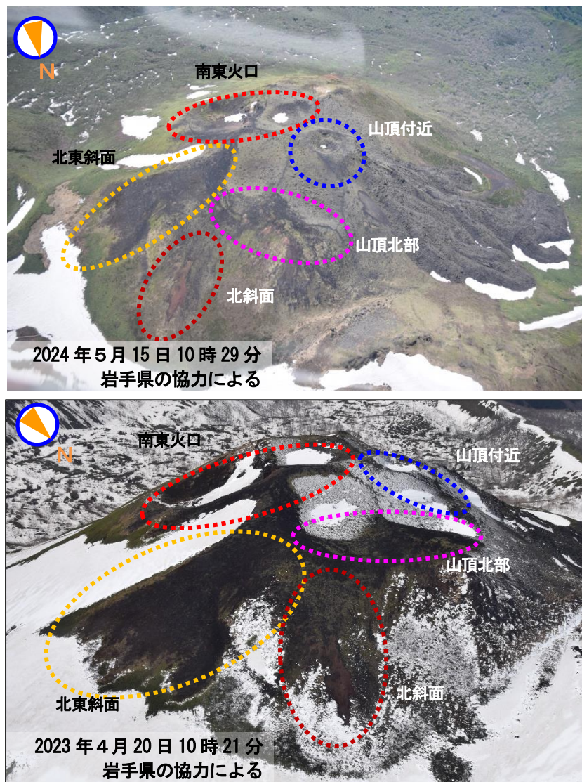
図7 秋田駒ヶ岳 上空からの南東火口、北東斜面、北斜面、山頂北部及び山頂付近の状況 ・ 図中の破線の色は、図2の破線の色に対応します。
