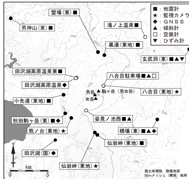
図 15 秋田駒ヶ岳 観測点配置図
