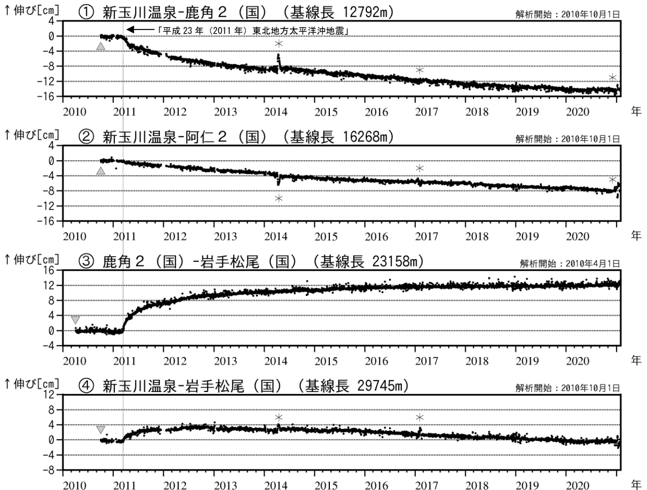
図4 秋田焼山 GNSS 基線長変化図（2010年4月～2021年1月）
