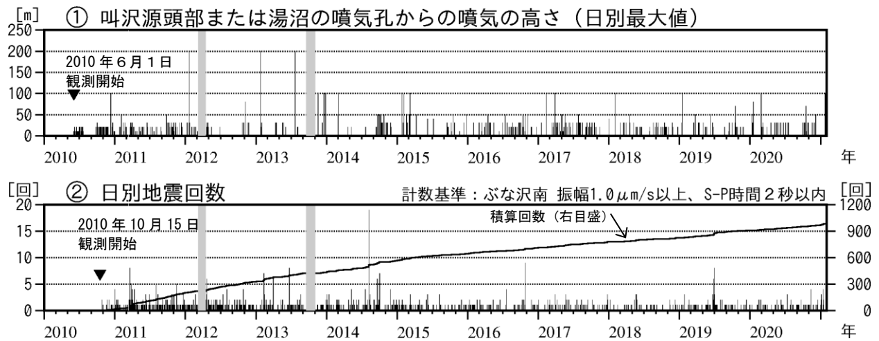
図3 秋田焼山 火山活動経過図（2010年6月～2021年1月）
