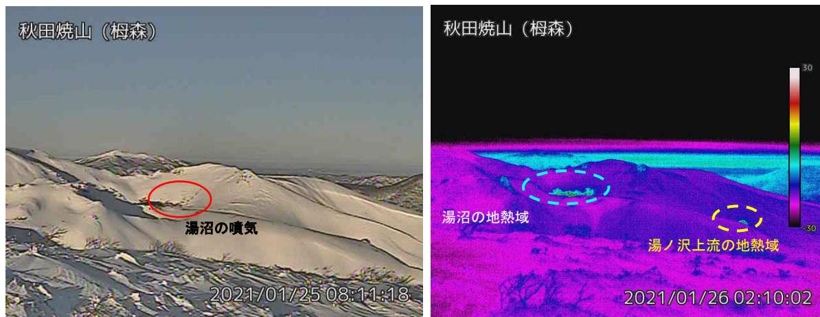
図2 秋田焼山 湯沼と湯ノ沢上流の状況（1月25日）と地表面温度分布（1月26日） ・樽森監視カメラ（湯沼の東約1 km）の映像です。
