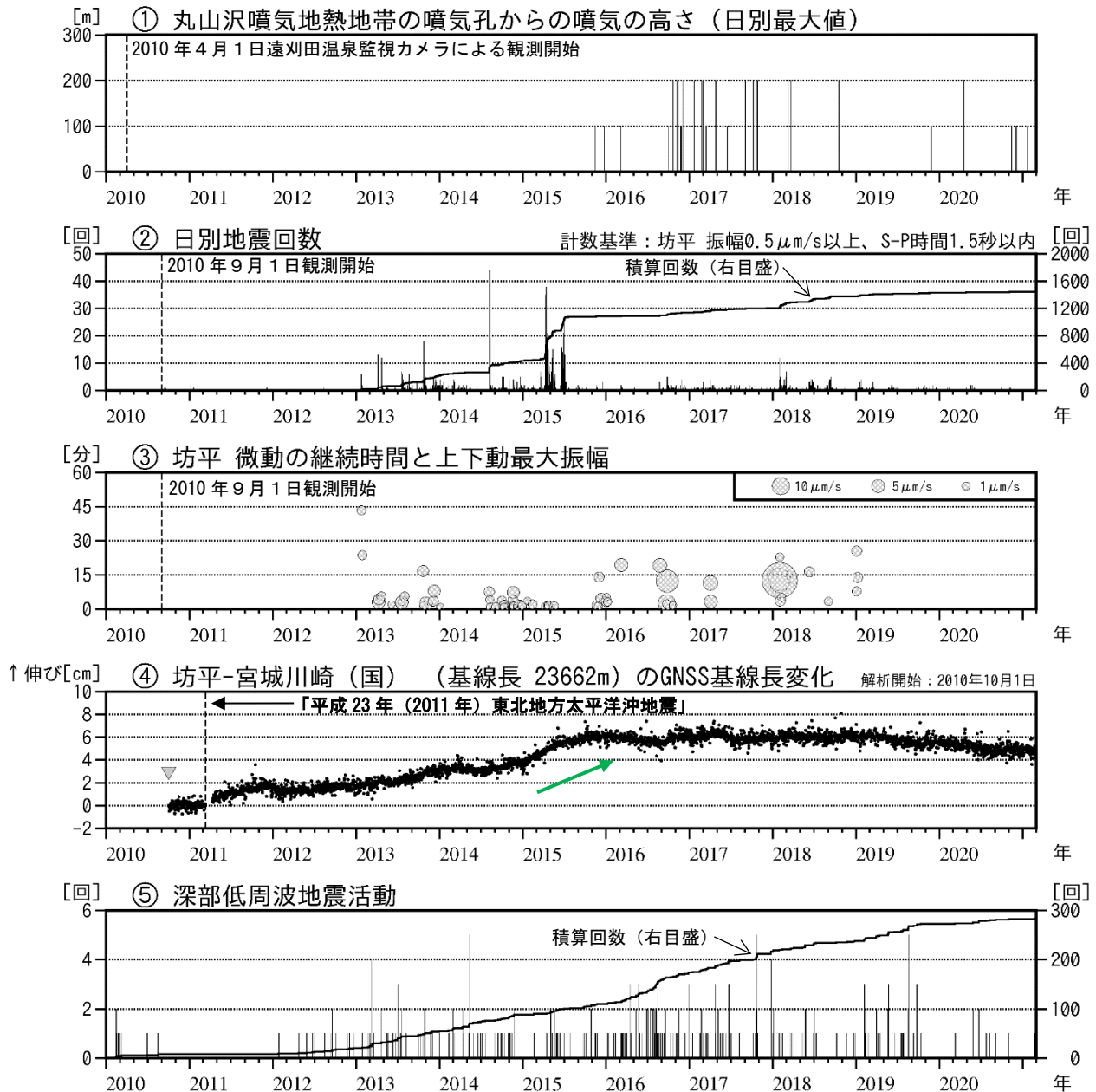
図2 蔵王山 火山活動経過図（2010年4月～2021年2月）
