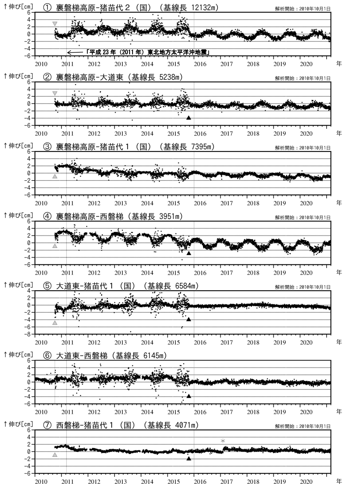
図4 磐梯山 GNSS 基線長変化図 (2010年1月～2021年2月)
