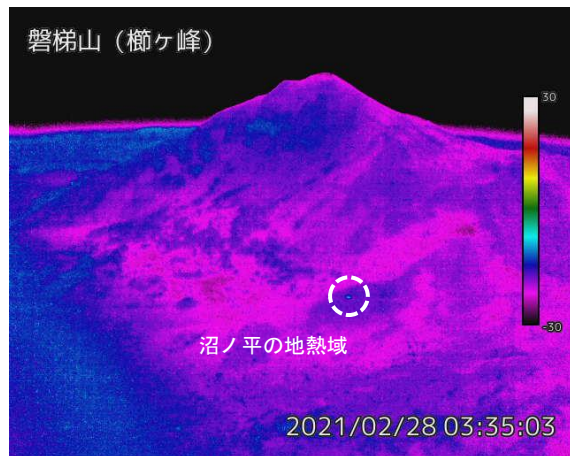
図2 磐梯山 沼ノ平周辺の状況と地表面温度分布（2月28日）
