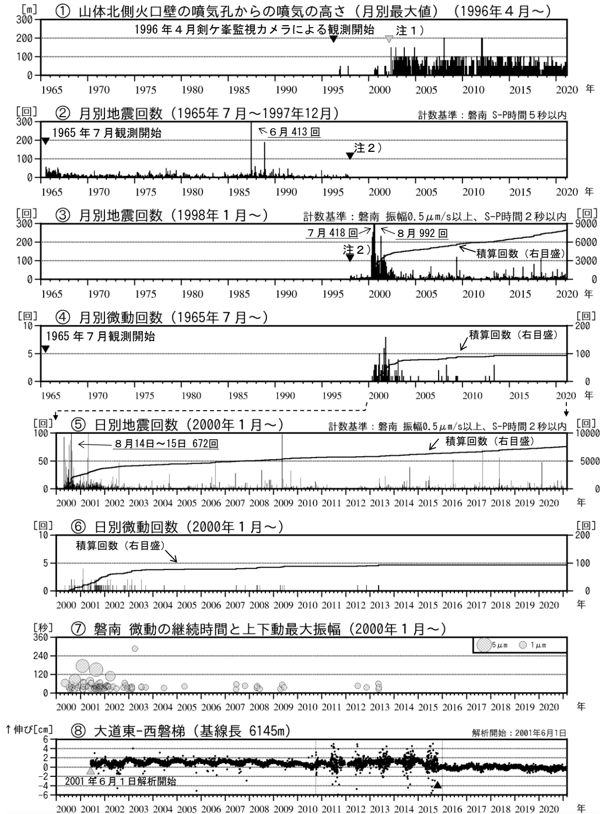
図3 磐梯山 火山活動経過図（1965年7月～2021年2月）
