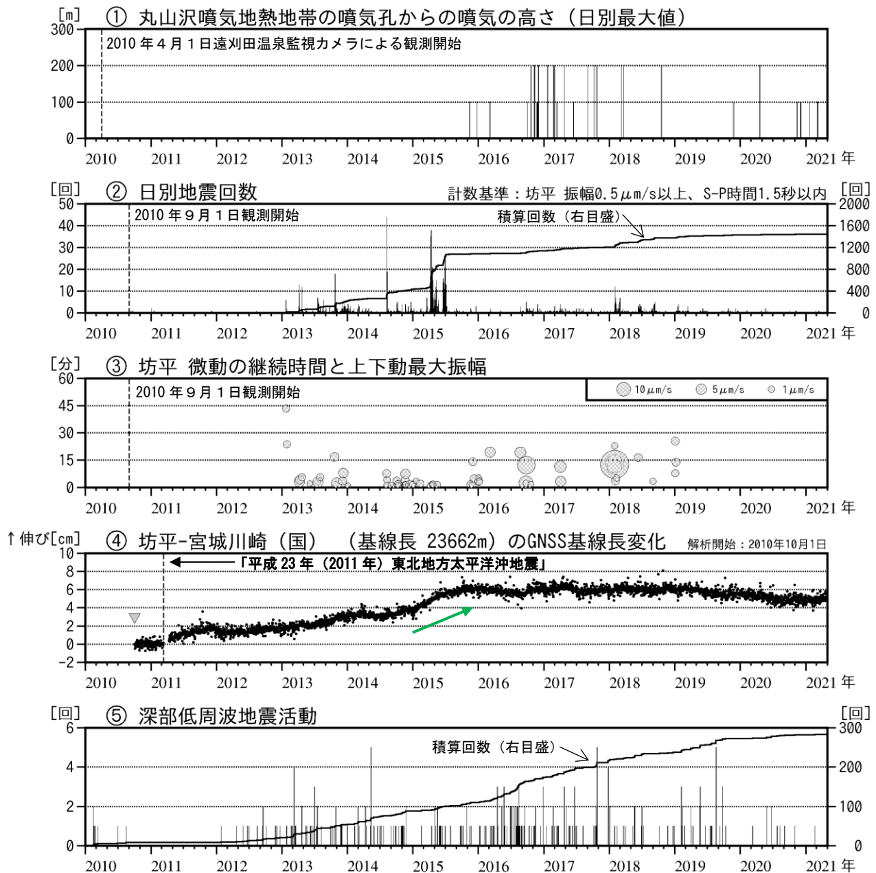
図2 蔵王山 火山活動経過図（2010年4月～2021年4月）
