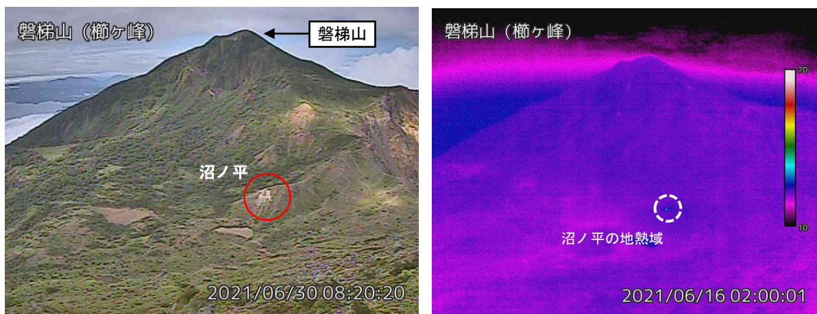
図2 磐梯山 沼ノ平周辺の状況（6月30日）と地表面温度分布（6月16日） ・櫛ヶ峰監視カメラ（沼ノ平の北東約600m）の映像です。
