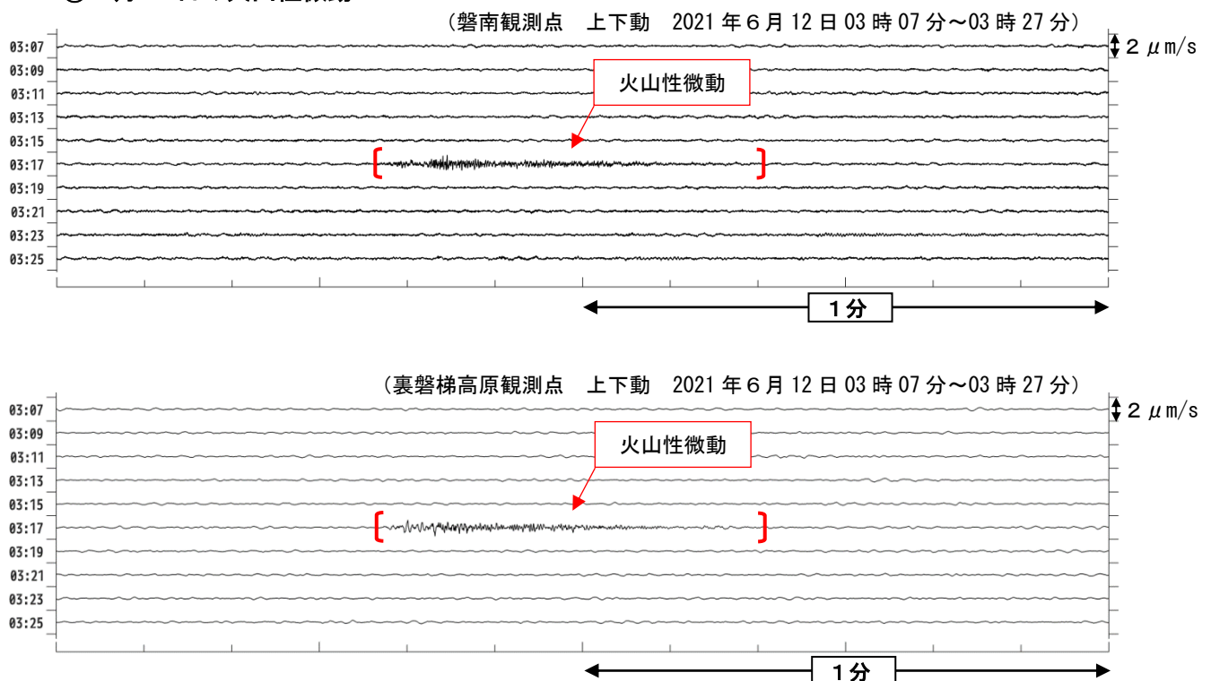
図4 磐梯山 火山性微動の発生状況
