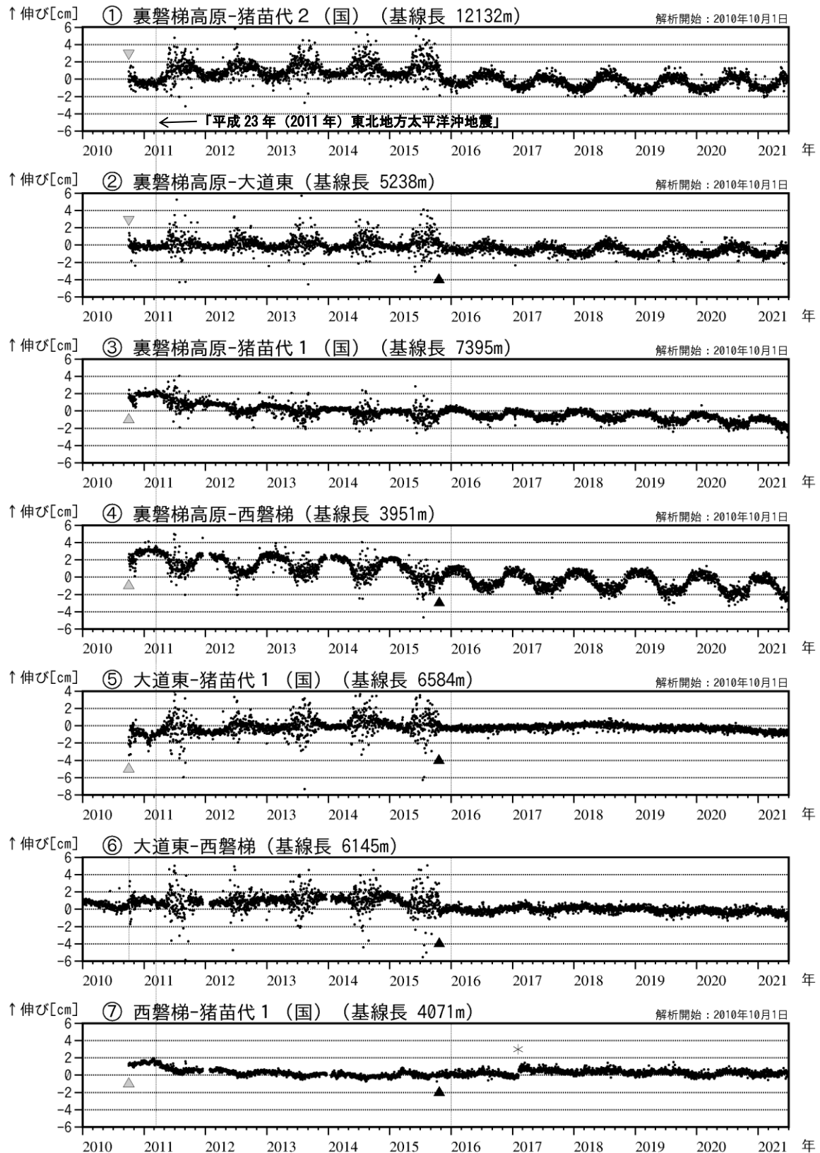
図5 磐梯山 GNSS 基線長変化図 (2010年1月～2021年6月)
