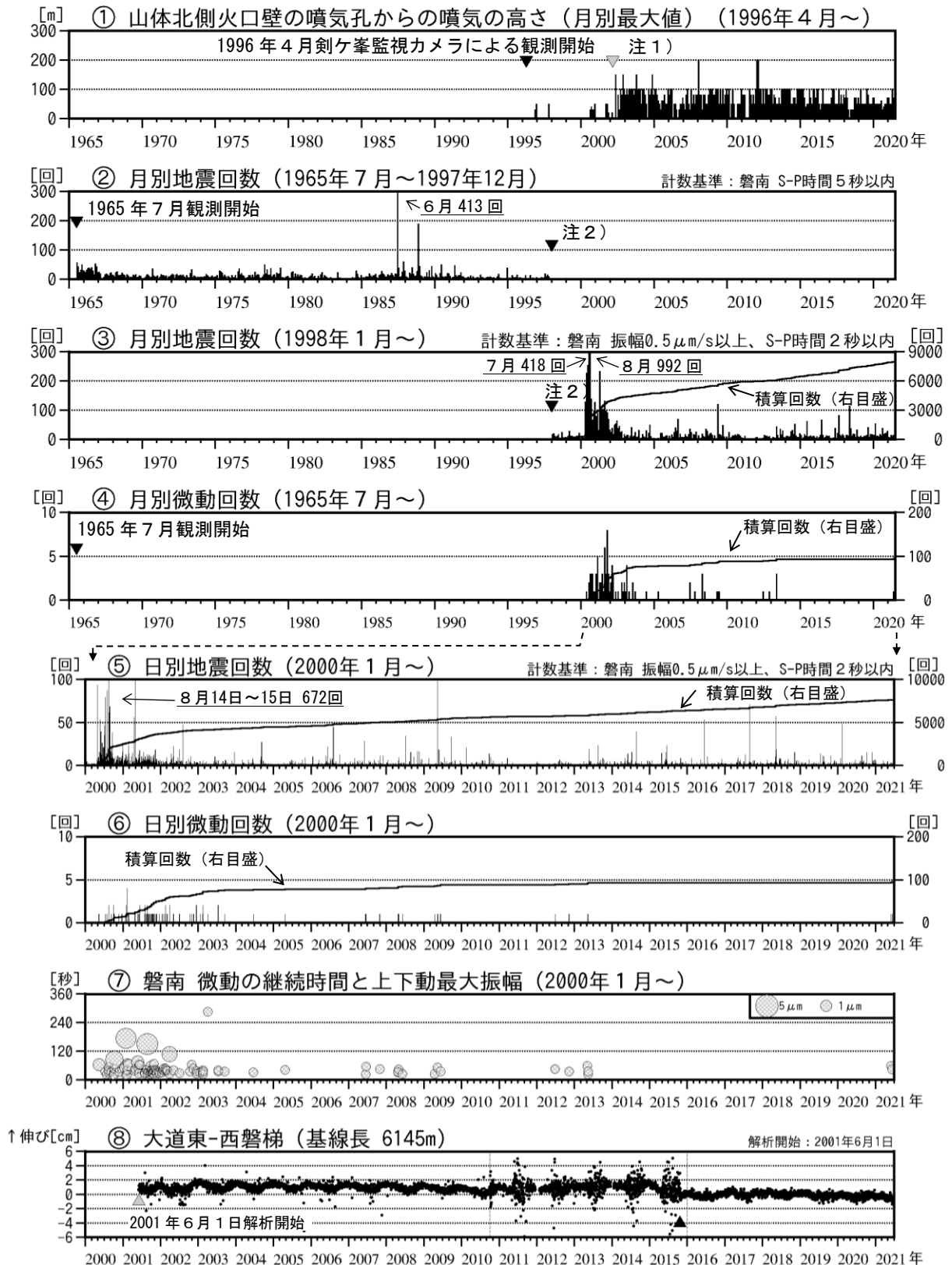
図3 磐梯山 火山活動経過図（1965年7月～2021年6月）
