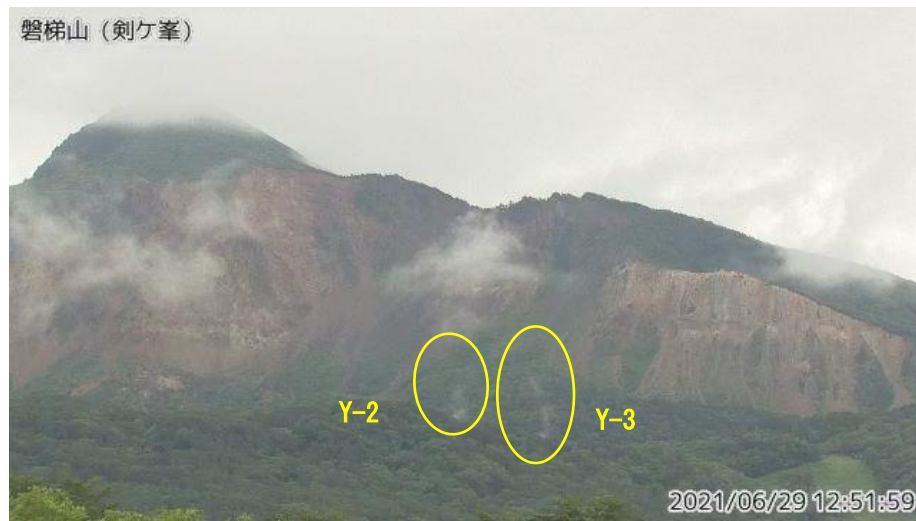
図1 磐梯山 山体北側火口壁の噴気の状態（6月29日） ・剣ヶ峰監視カメラ（山頂の北約7km）の映像です。
