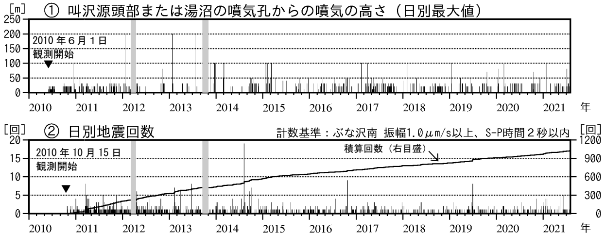
図3 秋田焼山 火山活動経過図（2010年6月～2021年7月）
