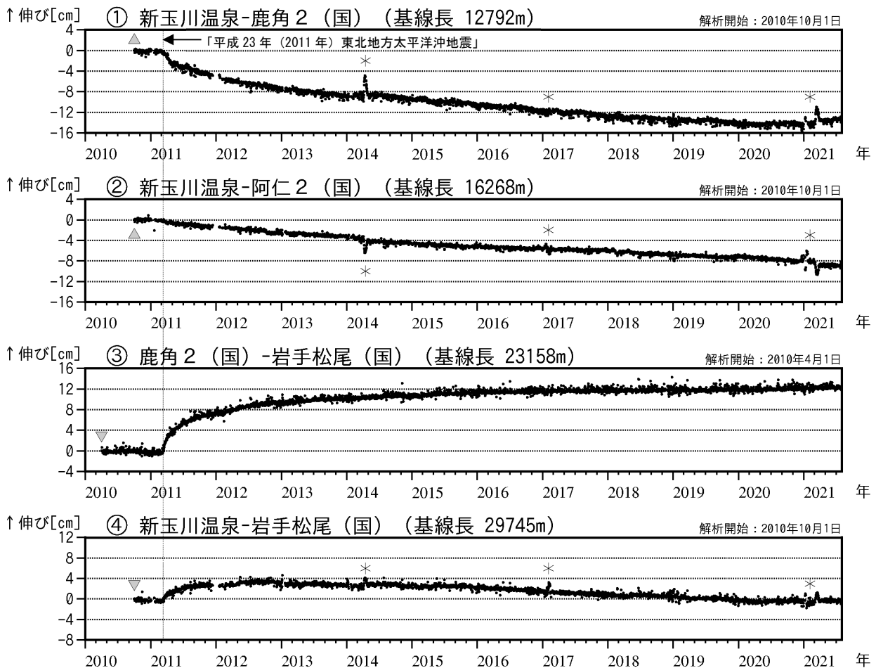
図4 秋田焼山 GNSS 基線長変化図（2010年4月～2021年7月）
