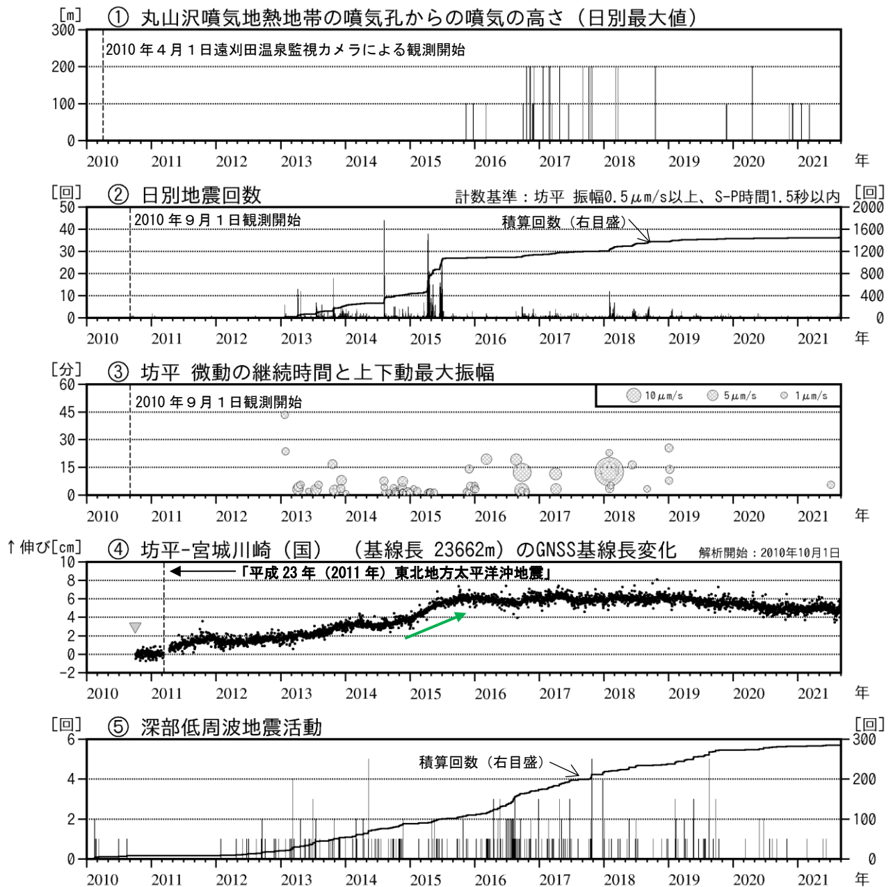
図2 蔵王山 火山活動経過図（2010年4月～2021年8月）
