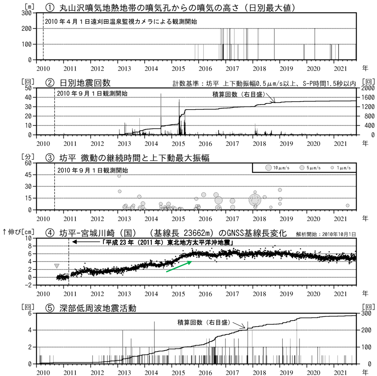
図2 蔵王山 火山活動経過図（2010年4月～2021年10月）
