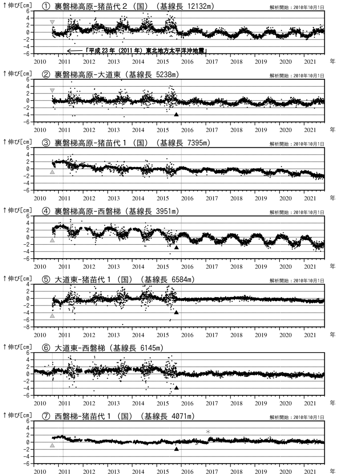
図4 磐梯山 GNSS 基線長変化図 (2010年1月～2021年10月)
