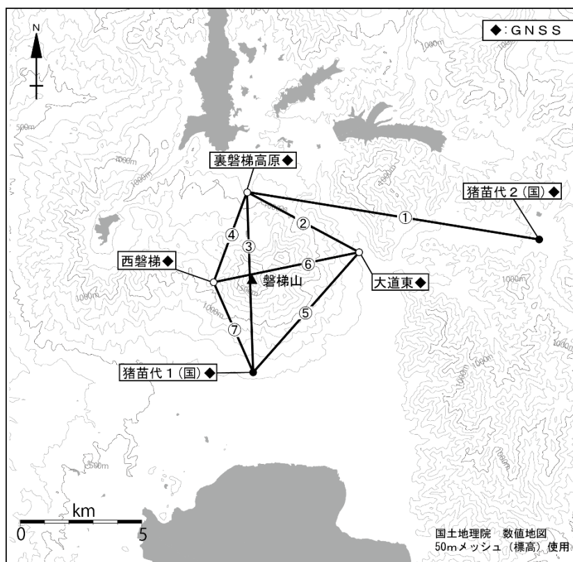
図6 磐梯山 GNSS 観測基線図
