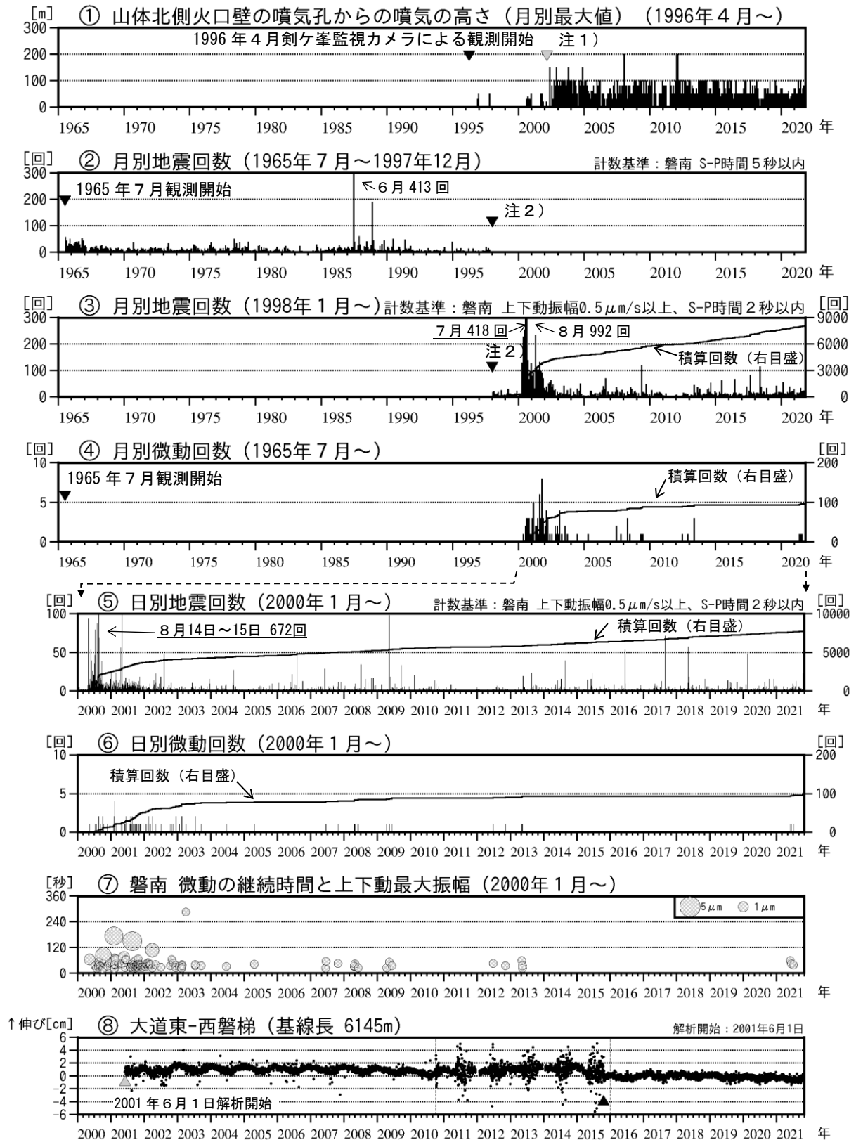
図3 磐梯山 火山活動経過図（1965年7月～2021年10月）
