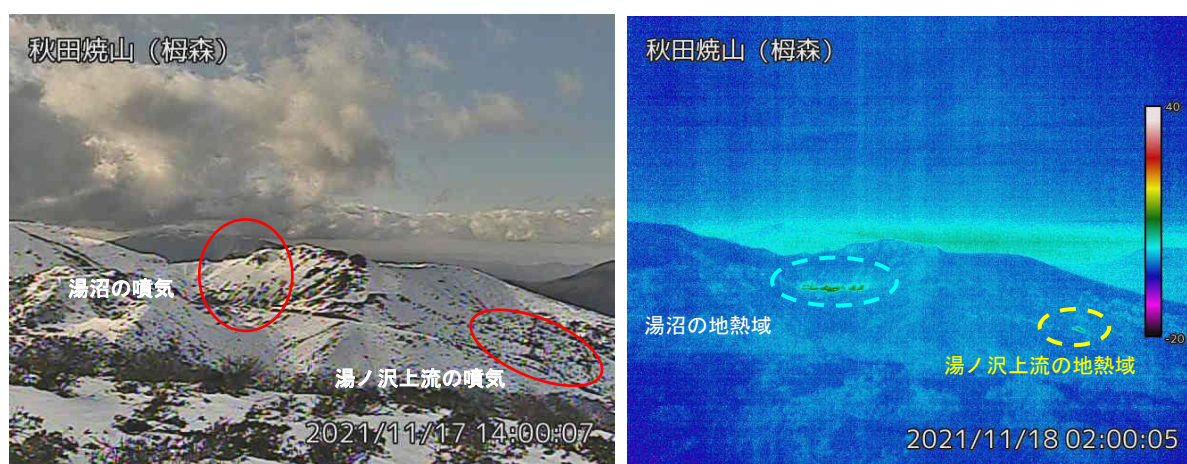
図2 秋田焼山 湯沼と湯ノ沢上流の状況（11月17日）と地表面温度分布（11月18日）
