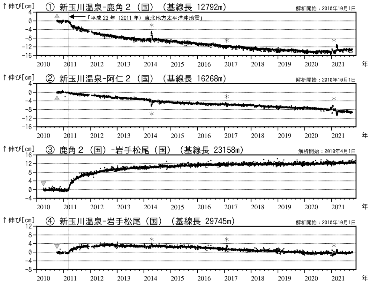
図4 秋田焼山 GNSS 基線長変化図（2010年4月～2021年11月）
