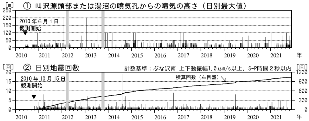
図3 秋田焼山 火山活動経過図（2010年6月～2021年11月）
