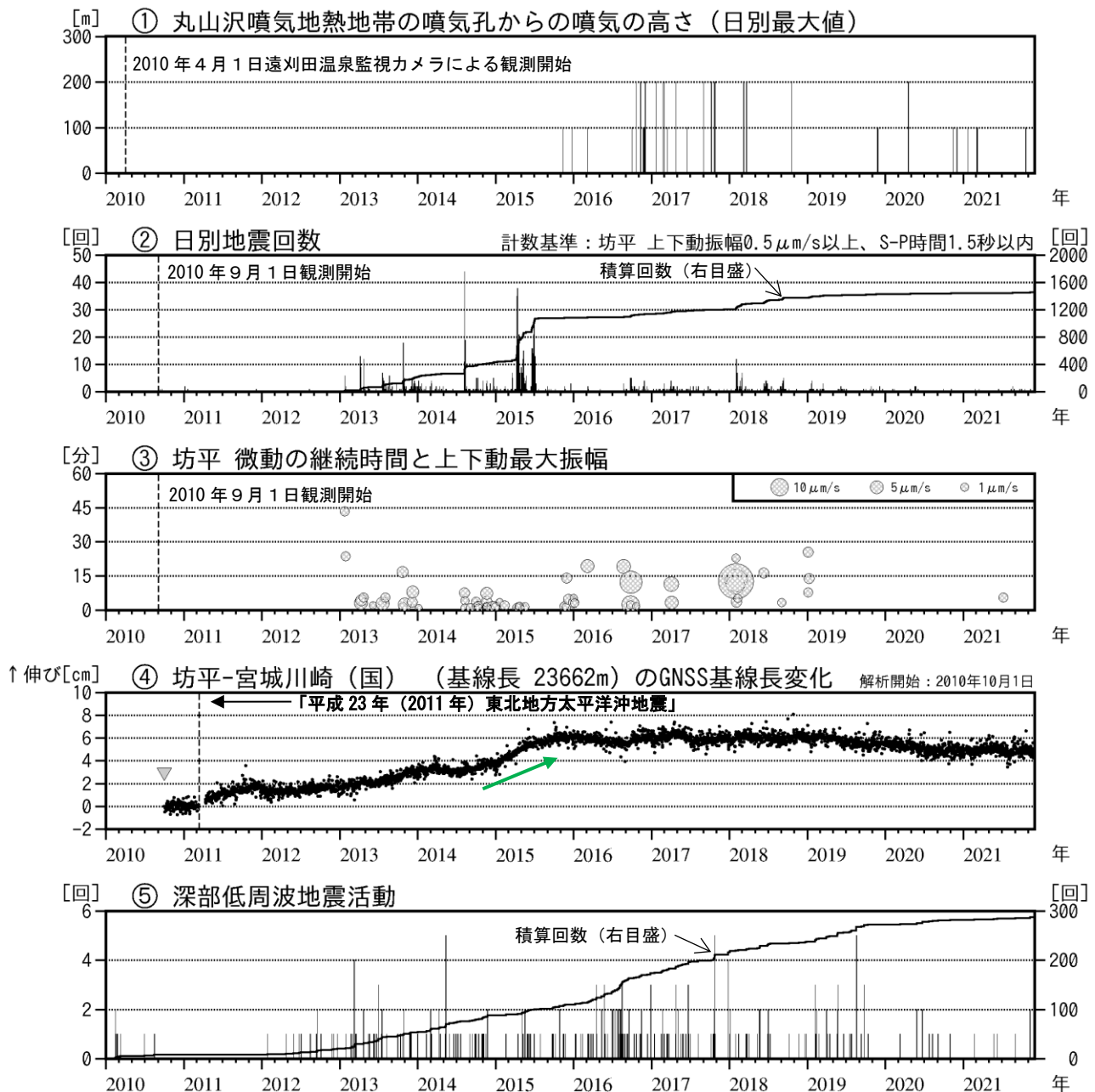
図2 蔵王山 火山活動経過図（2010年4月～2021年11月）
