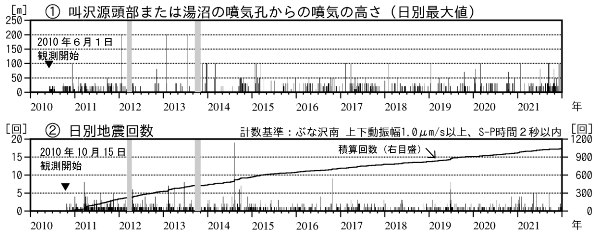
図3 秋田焼山 火山活動経過図（2010年6月～2021年12月）
