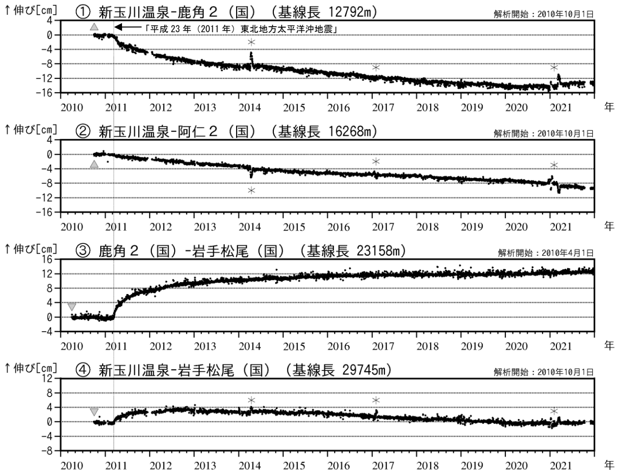
図4 秋田焼山 GNSS 基線長変化図（2010年4月～2021年12月）
