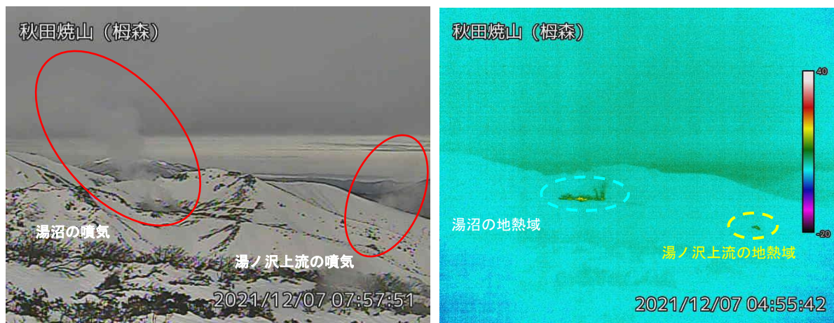
図2 秋田焼山 湯沼と湯ノ沢上流の状況と地表面温度分布（12月7日）
