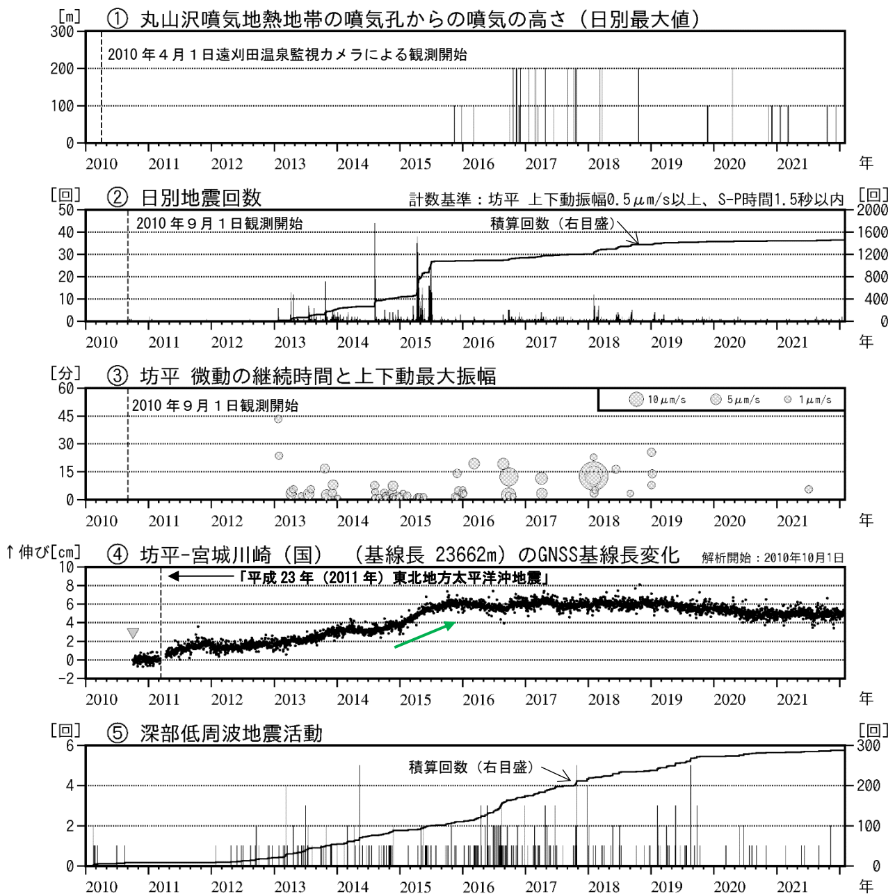
図2 蔵王山 火山活動経過図（2010年4月～2022年1月）
