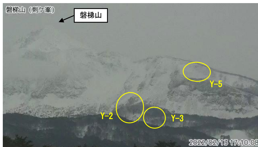
図1 磐梯山 山体北側火口壁の噴気の状況（2月13日）
