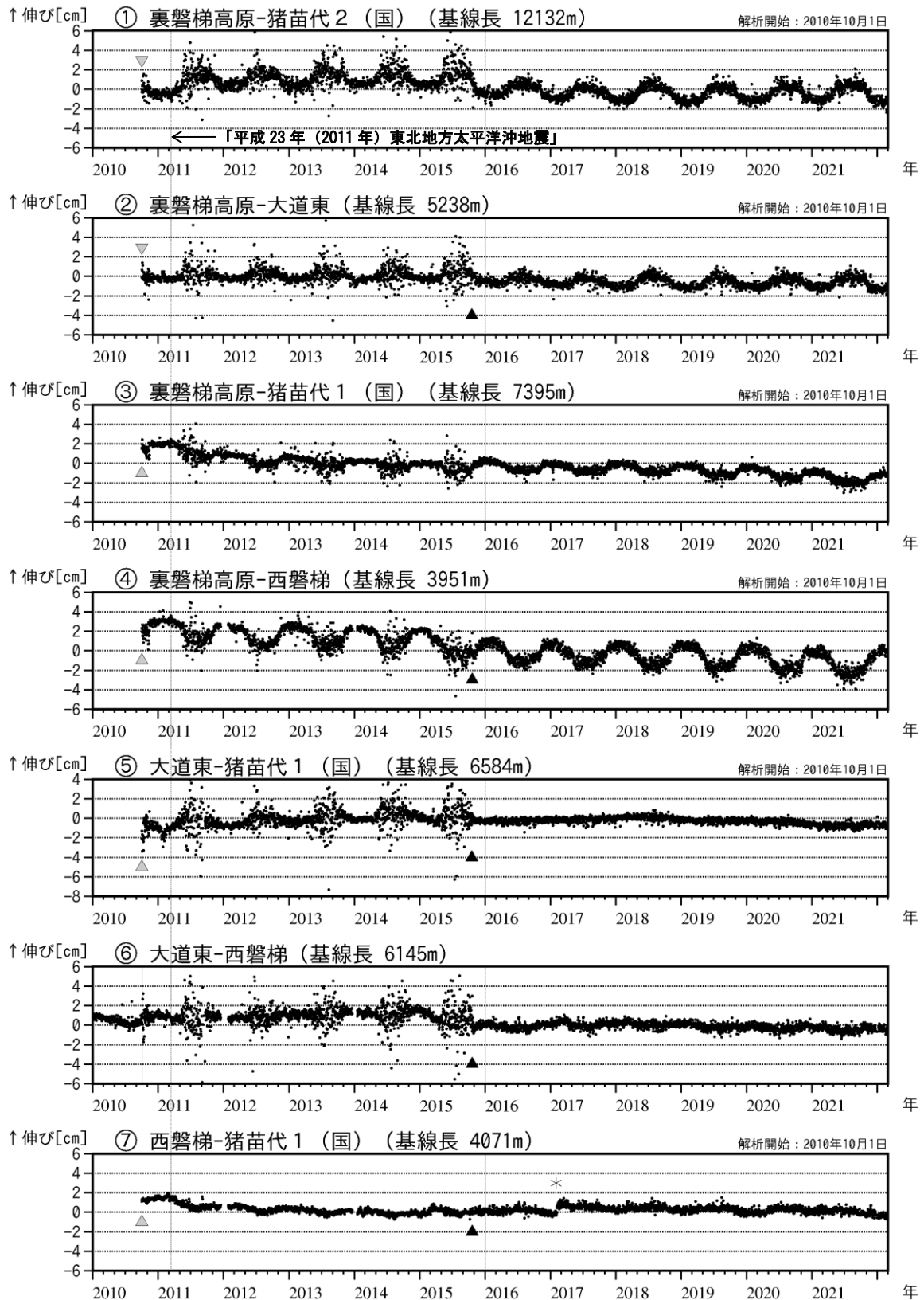
図3 磐梯山 GNSS 基線長変化図 (2010年1月～2022年2月)
