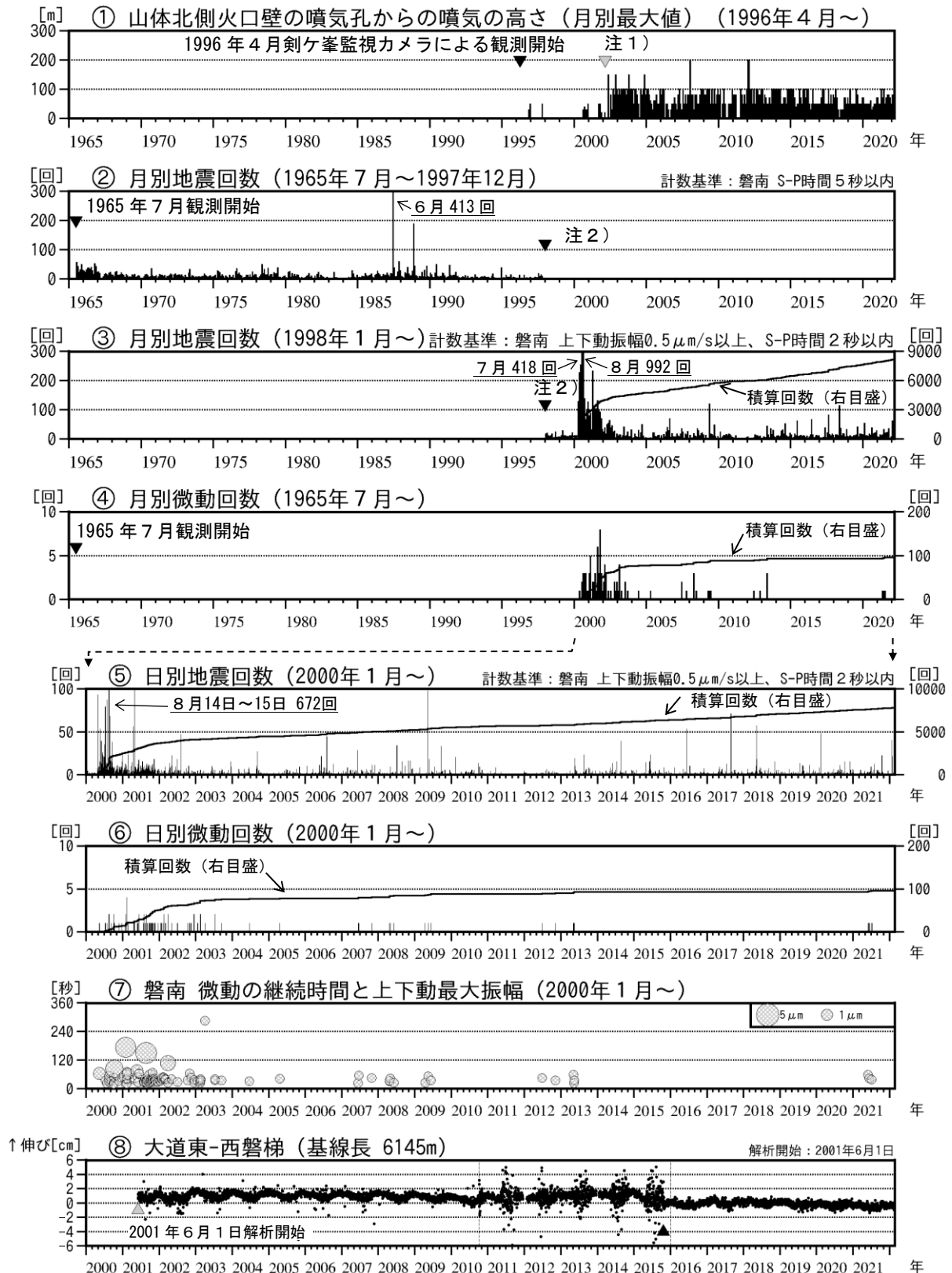
図2 磐梯山 火山活動経過図（1965年7月～2022年2月）
