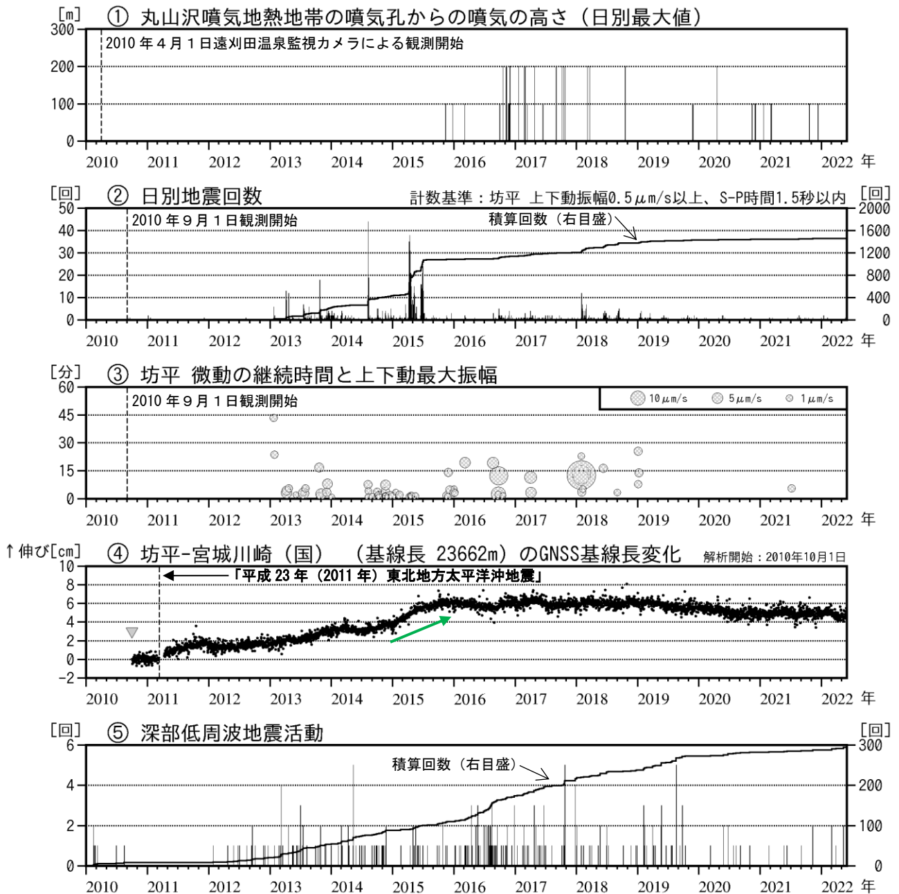
図2 蔵王山 火山活動経過図（2010年4月～2022年5月）
