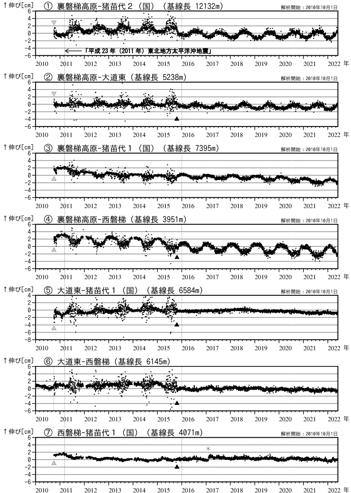
図4 磐梯山 GNSS 基線長変化図 (2010年1月～2022年5月)
