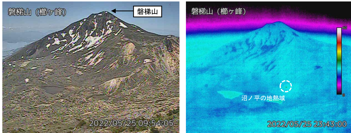
図2 磐梯山 沼ノ平周辺の状況と地表面温度分布（5月25日）
