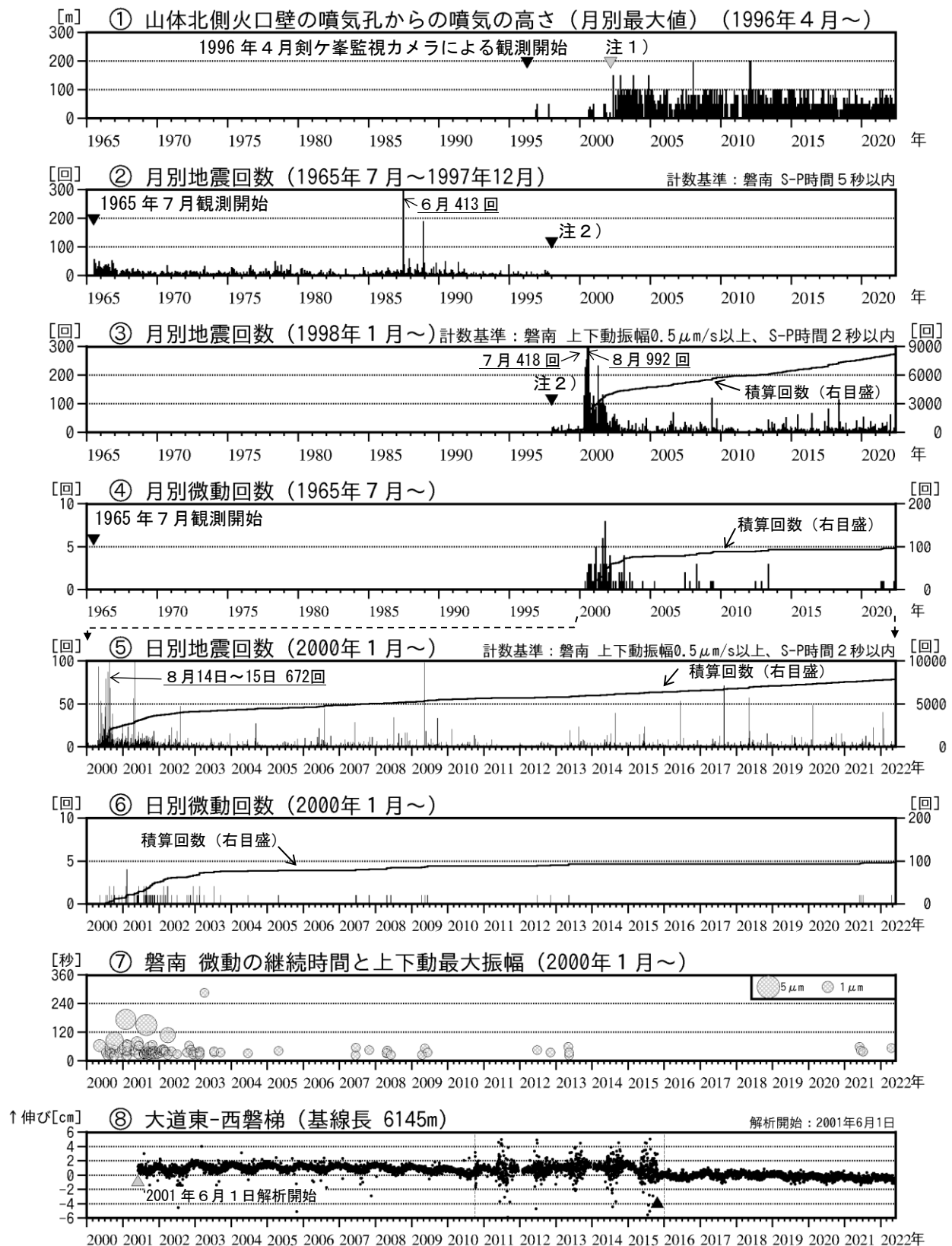
図3 磐梯山 火山活動経過図（1965年7月～2022年5月）
