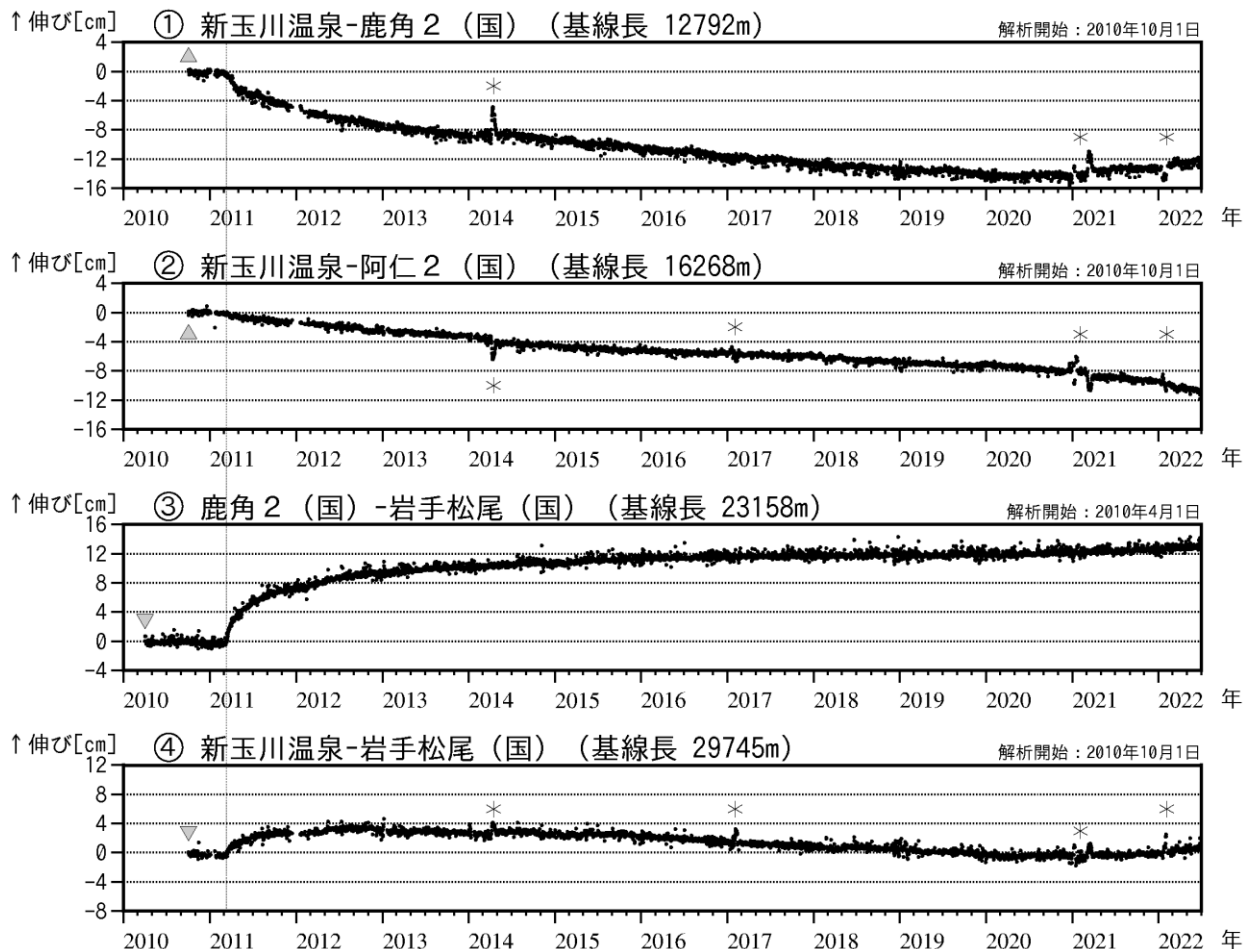
図4 秋田焼山 GNSS 基線長変化図（2010年4月～2022年6月）
