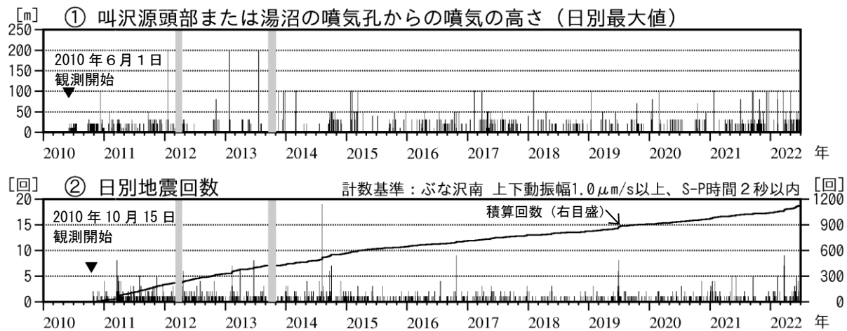
図3 秋田焼山 火山活動経過図（2010年6月～2022年6月）
