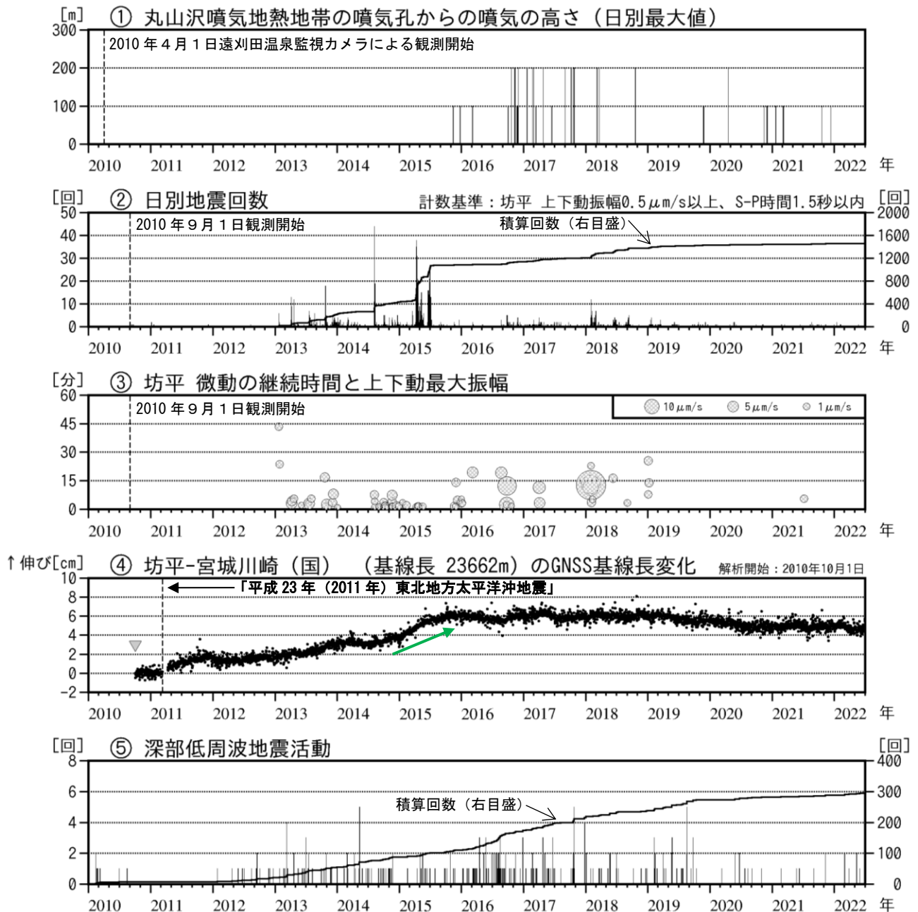
図3 蔵王山 火山活動経過図（2010年4月～2022年6月）
