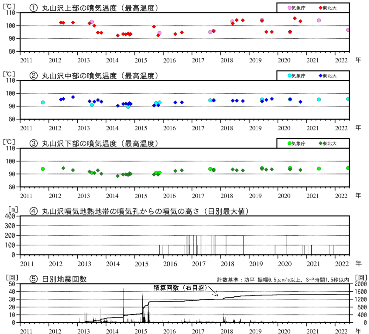
図2 蔵王山 丸山沢の噴気温度、噴気の高さ及び日別地震回数（2011年1月～2022年6月）
