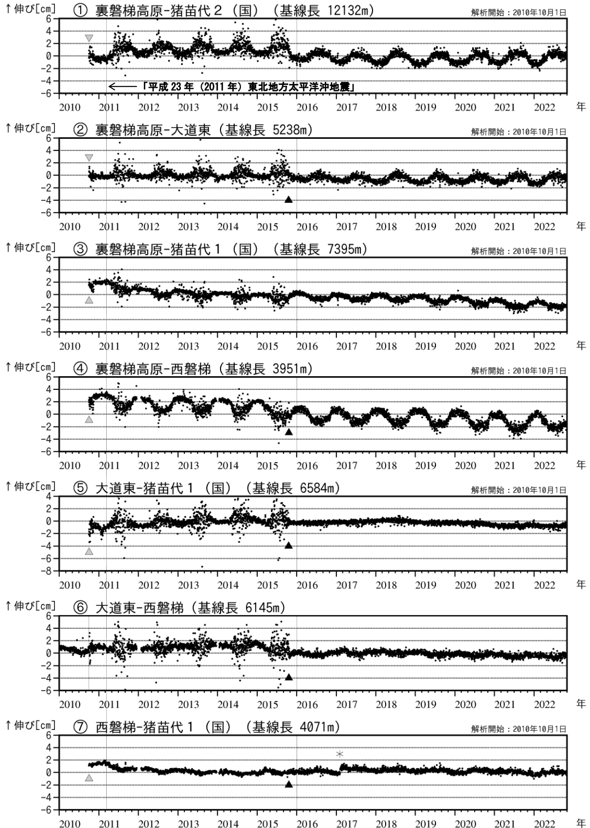
図4 磐梯山 GNSS 基線長変化図 (2010年1月～2022年10月)
