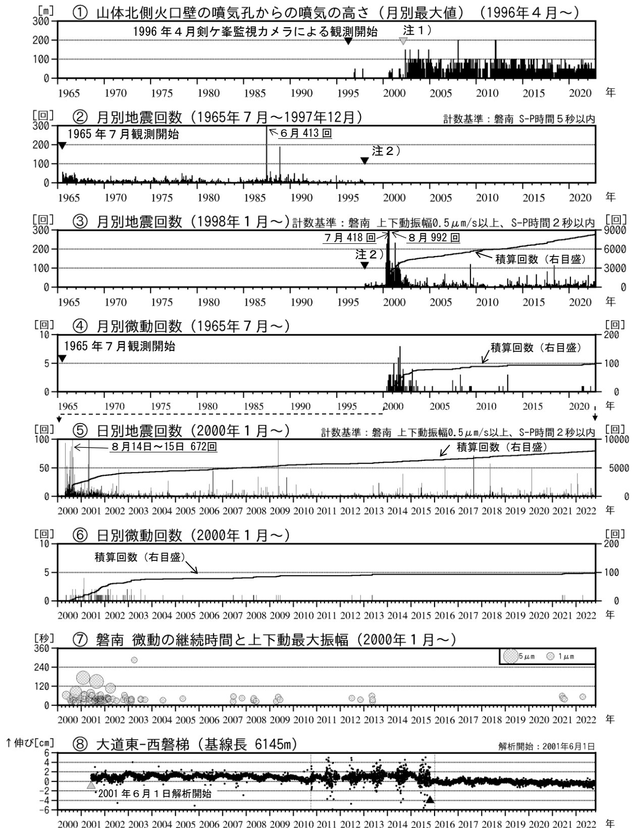
図3 磐梯山 火山活動経過図（1965年7月～2022年10月）
