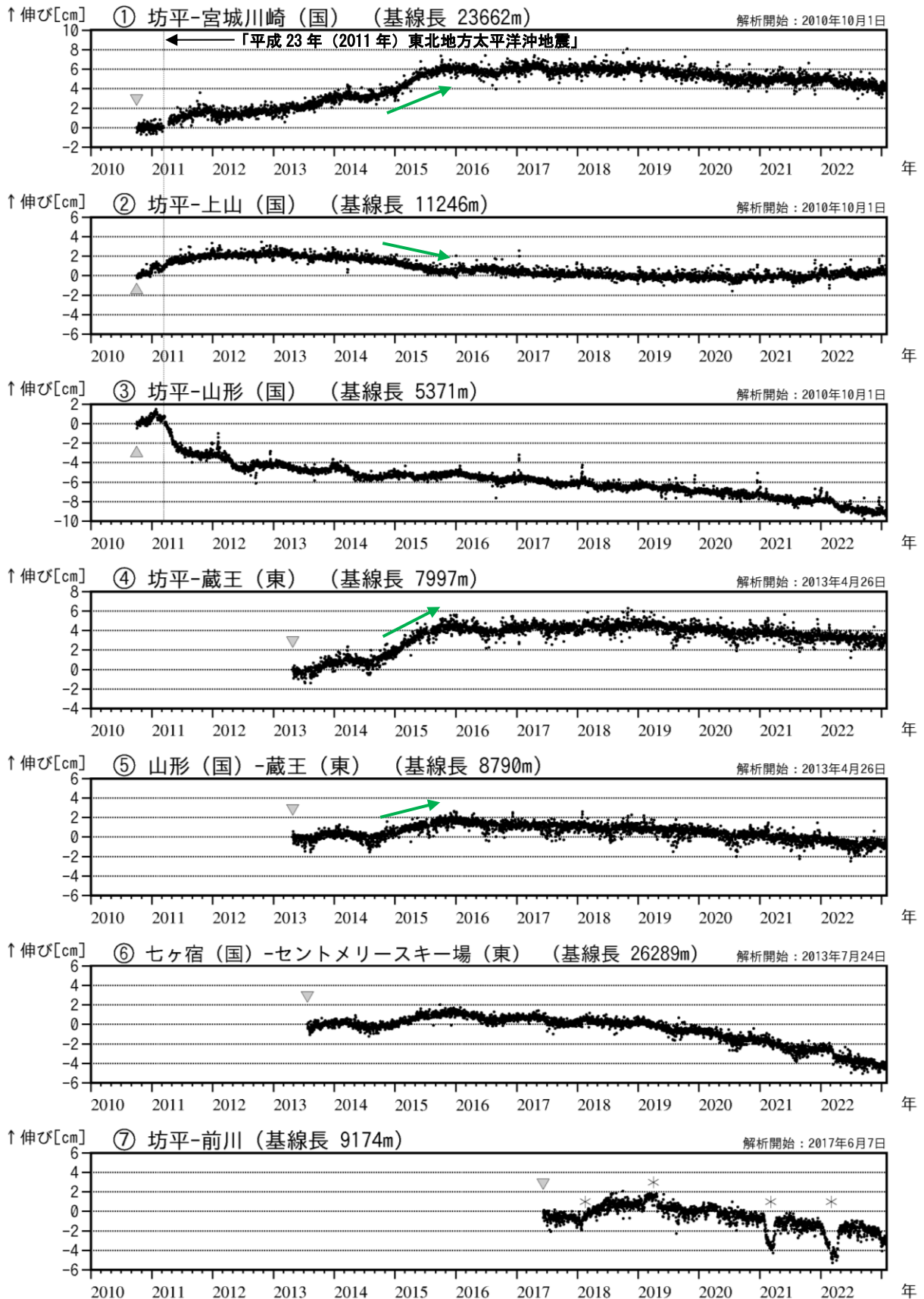
図3 蔵王山 GNSS 基線長変化図（2010年10月～2023年1月）
