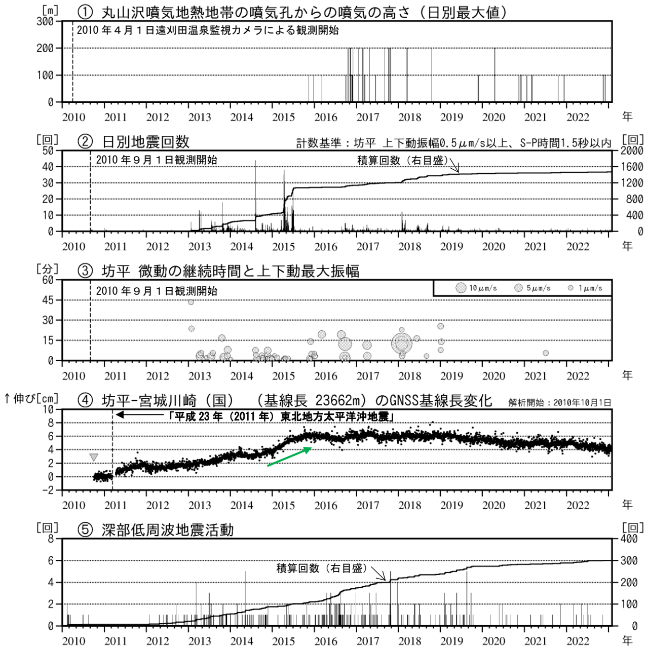
図2 蔵王山 火山活動経過図（2010年4月～2023年1月）
