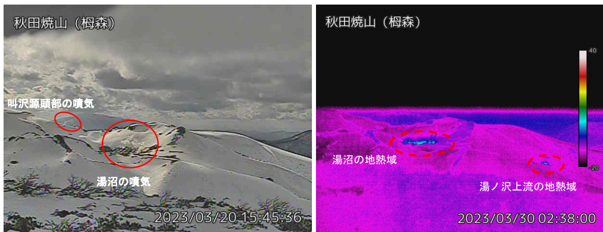
図2 秋田焼山 湯沼と湯ノ沢上流の状況（3月20日）と地表面温度分布（3月30日） ・柵森監視カメラ（湯沼の東約1 km）の映像です。
