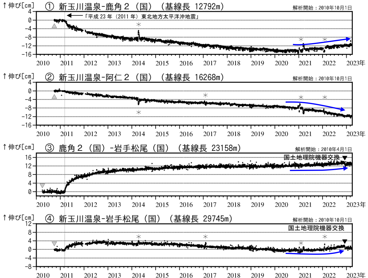
図4 秋田焼山 GNSS 基線長変化図（2010年4月～2023年3月）
