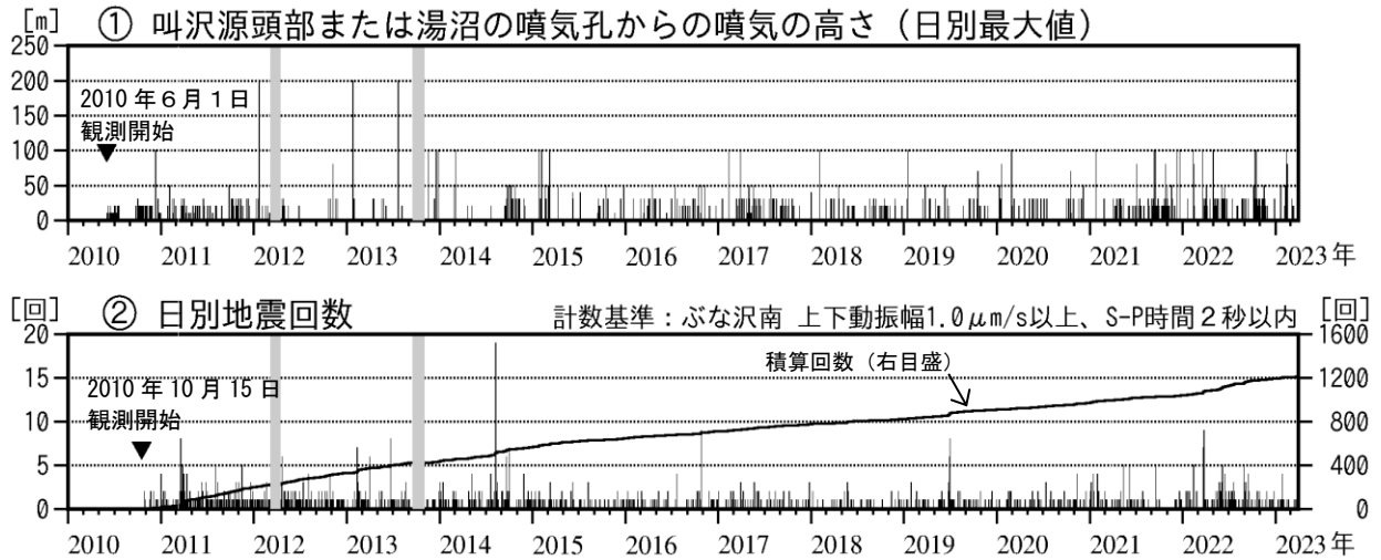
図3 秋田焼山 火山活動経過図（2010年6月～2023年3月）
