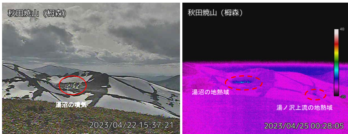
図2 秋田焼山 湯沼と湯ノ沢上流の状況（4月22日）と地表面温度分布（4月25日）
