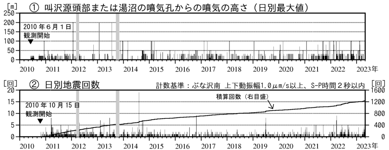
図3 秋田焼山 火山活動経過図（2010年6月～2023年4月）
