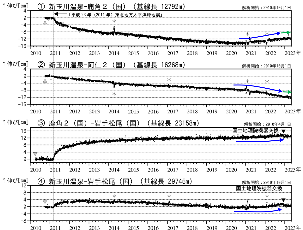
図4 秋田焼山 GNSS 基線長変化図（2010年4月～2023年4月）
