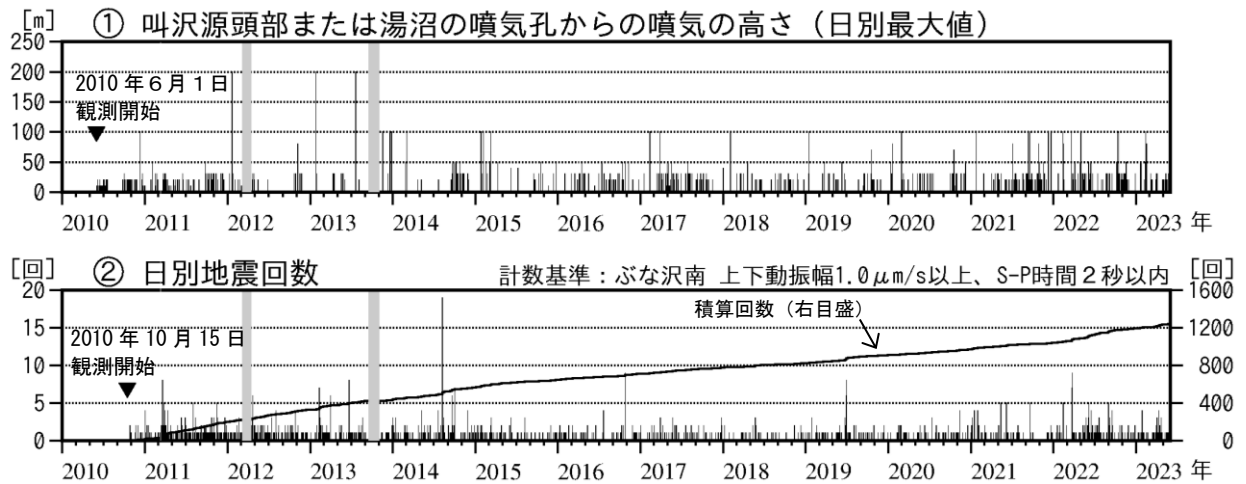
図3 秋田焼山 火山活動経過図（2010年6月～2023年5月）
