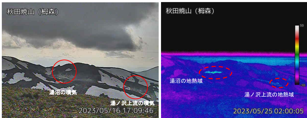
図2 秋田焼山 湯沼と湯ノ沢上流の様（5月16日）と地表面温度分布（5月25日）
