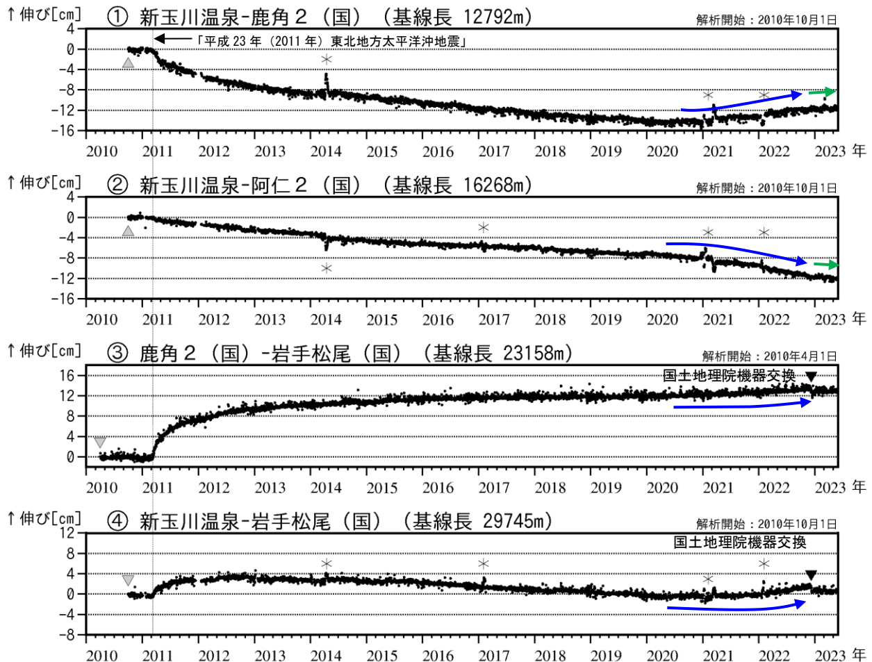
図4 秋田焼山 GNSS 基線長変化図（2010年4月～2023年5月）
