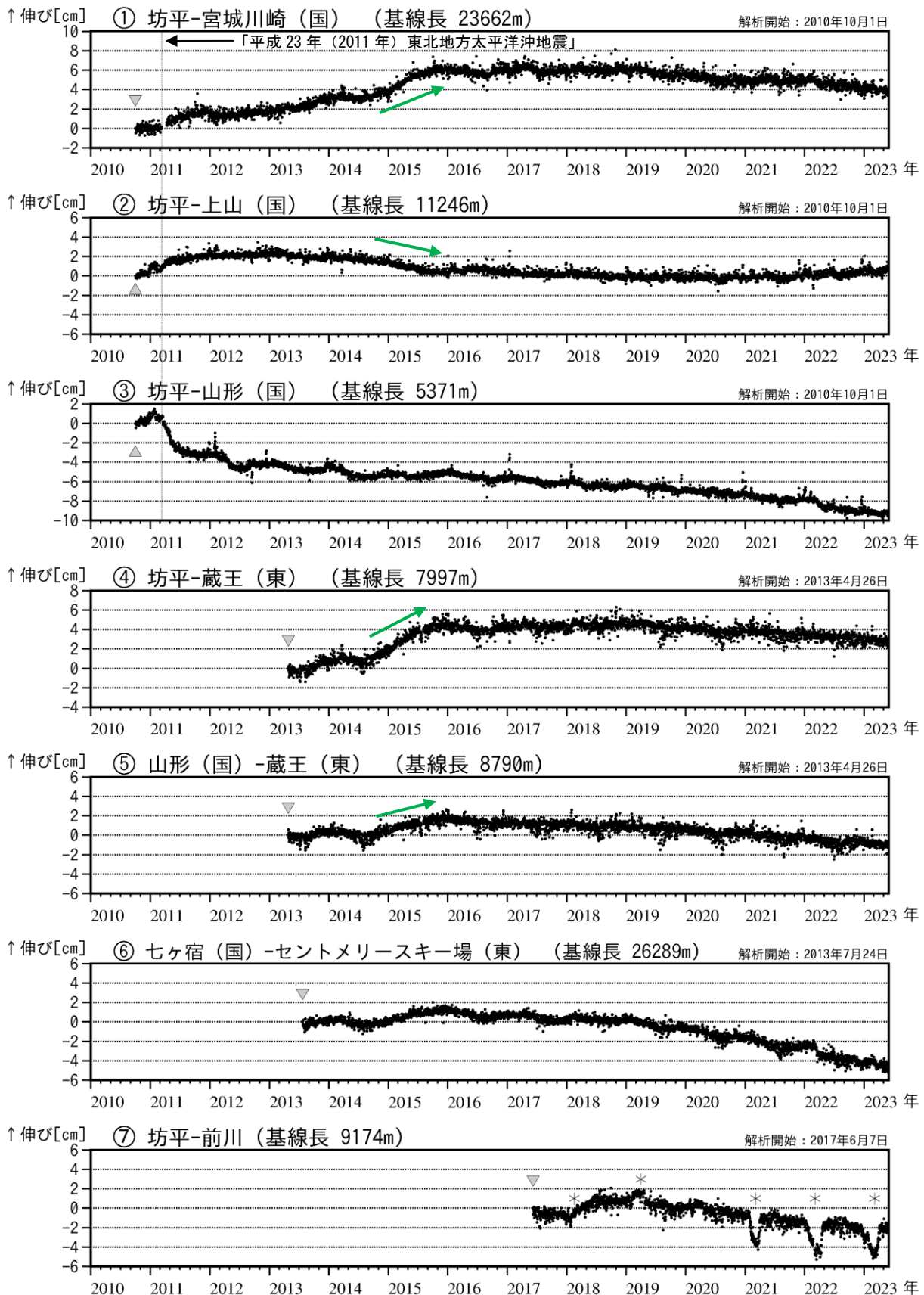
図3 蔵王山 GNSS 基線長変化図 (2010 年 10 月～2023 年 5 月)
