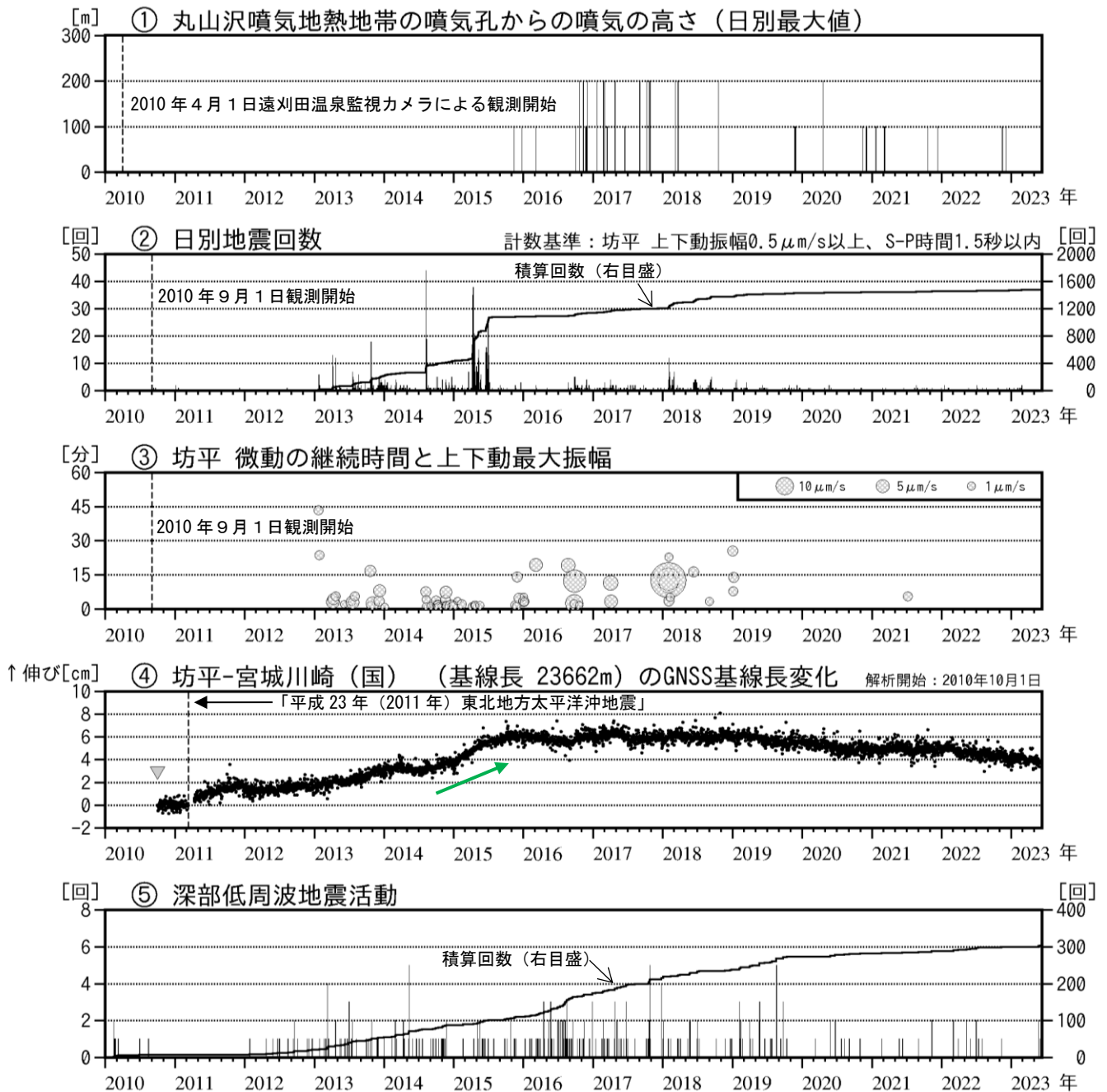
図2 蔵王山 火山活動経過図（2010年4月～2023年5月）
