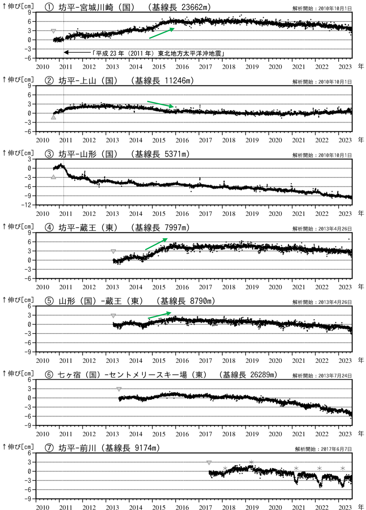
図3 蔵王山 GNSS 基線長変化図（2010年10月～2023年7月）
